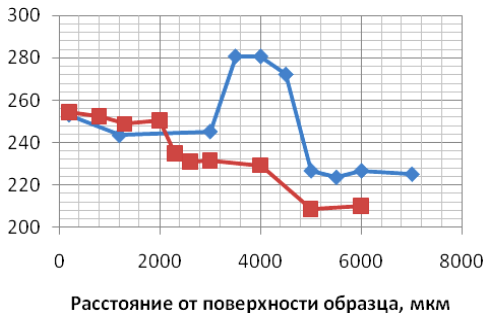
Рис. 1. Микротвердость в сечениях 1 – 1, 2 – 2 образца № 13: ряд 1 – поперечное 1 – 1, от наплавки к центру стержня; ряд 2 – продольное 2 – 2, от края поверхности к центру
