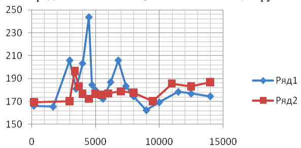
Рис. 4. Микротвердость в сечениях 1 – 1, 2 – 2 образца № 57-1: ряд 1 – сечение 1 – 1, от наплавки к центру стержня; ряд 2 – продольное сечение 1 – 1, от края к центру
