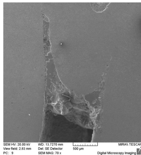
Рис. 7. Фрагмент непровара в корне шва образца № 65
