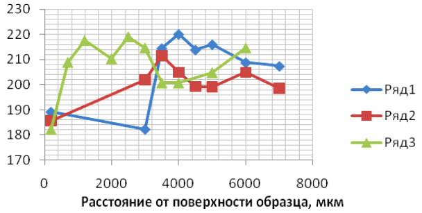
Рис. 3. Микротвердость в сечениях 1 – 1, 2 – 2 образца № 41: ряд 1 – сечение 1 – 1, от шва к центру левого стержня; ряд 2 – сечение 1 – 1, от шва к центру правого стержня; ряд 3 – сечение 2 – 2, от излома шва к центру
