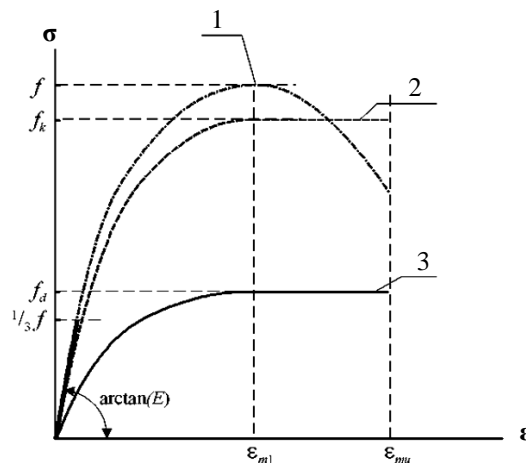
Рис. 1. Диаграмма деформирования (состояния) каменной кладки при осевом кратковременном сжатии по [2]:
