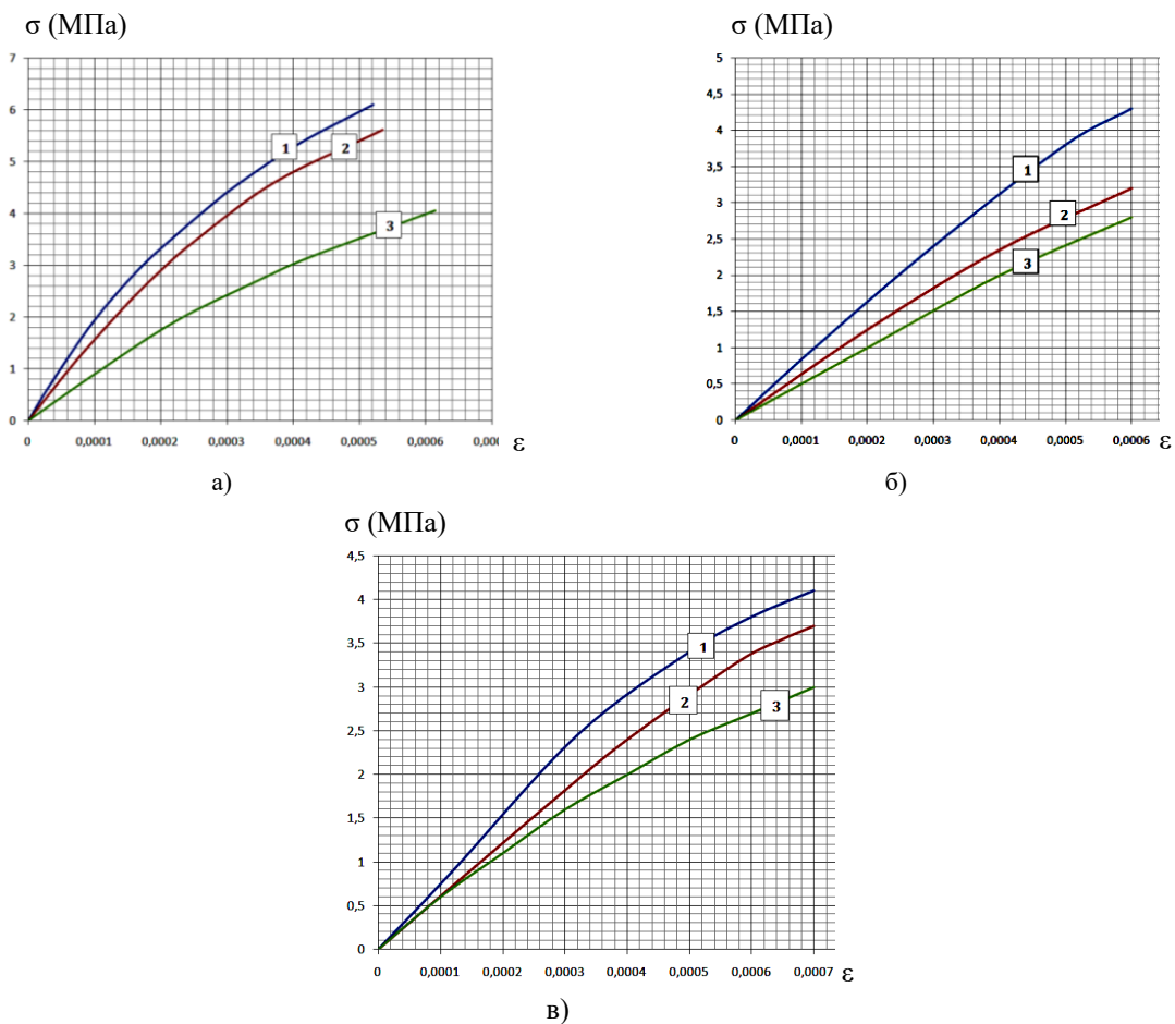
Рис. 3. Зависимости « \sigma - \varepsilon » образцов серии КРО (а), серии КРПУ (б), серии СУР (в): 1 – при прочности раствора 10,9 МПа; 2 – при прочности раствора 7,9 МПа; 3 – при прочности раствора 3,1 МПа
