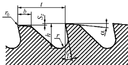
Рис. 3. Профиль стружечной канавки
