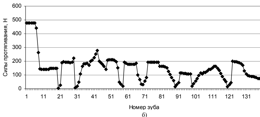
Рис. 6. Изменения уровней удельных k_c и главных P_z сил резания на отдельных зубах протяжки
