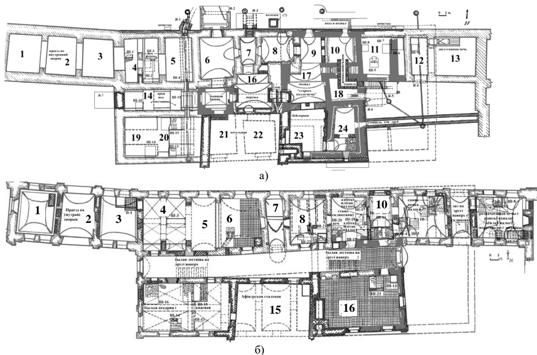
Мал. 1. Планы падвала (а) і першага паверха (б) перад рамонтам 2006 – 2008 гадоў.
