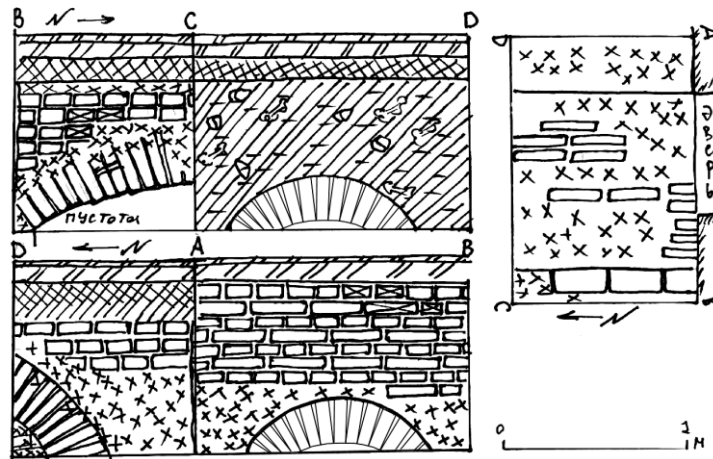
Мал. 5. Выгляд скляпення каналізацыйнага тунэля і арак-перамычак для лесвіцы сярэдзіны XVIII стагоддзя на другі паверх у шурфе калідора
