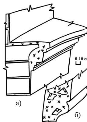
Мал. 3. Вапнавыя карнізы сярэдзіны XVIII – XIX стагоддзяў: а – па лекальнай цэгле; б – з кавалкамі дахоўкі XVIII – XIX стагоддзяў
