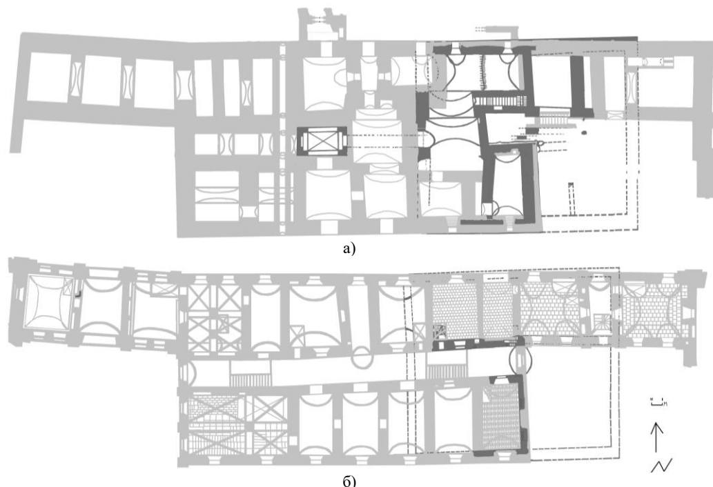
Мал. 10. Магчымая першапачатковая планіроўка XVIII стагоддзя падвала (а) і першага паверха (б) па выніках натуральных даследаванняў і планах 1828 года і пачатку XX стагоддзя (чорным колерам пазначаны рэшткі старадаўніх пабудов)
