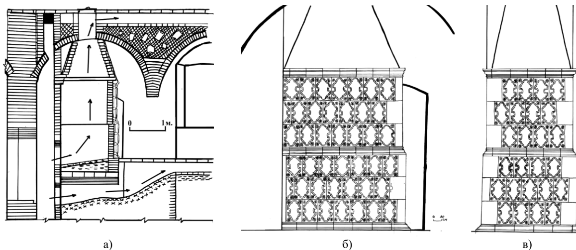
Мал. 6. Печ канца XVIII стагоддзя ў памяшканні № 13: рэканструкцыя разрэза (а) і знешняга выгляду паўднёвага (б) і ўсходняга (в) фасадаў
