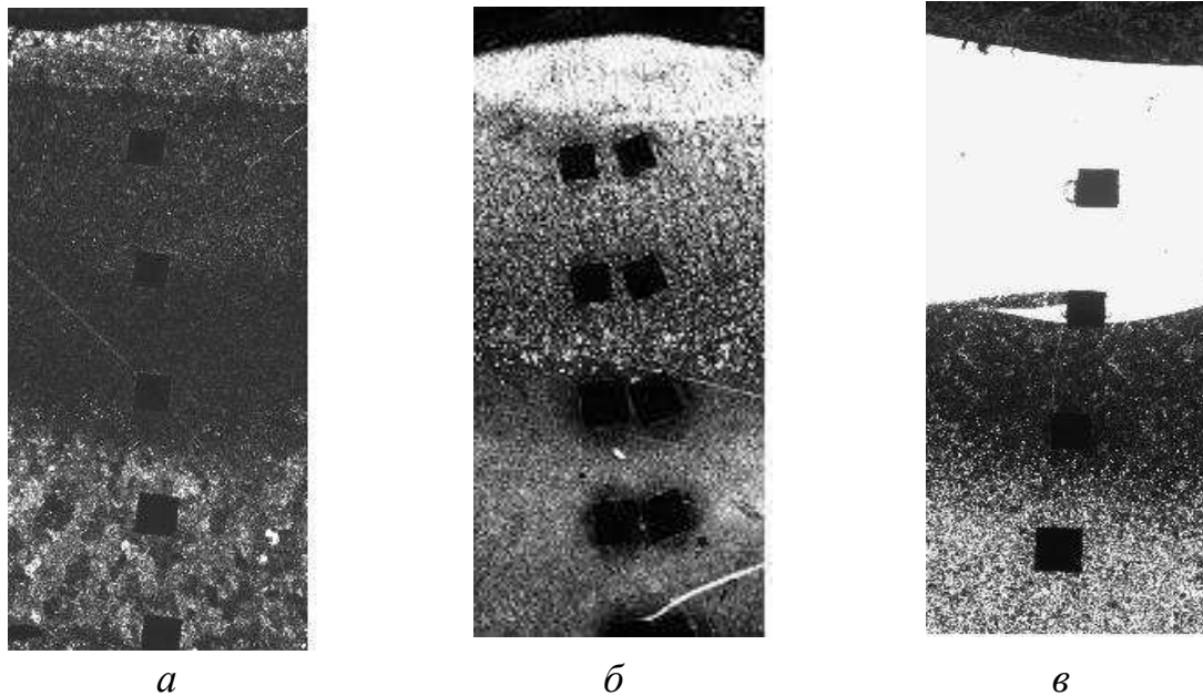
Рис. 1. Фотографии микроструктуры покрытий после МЭУ и лазерной обработки. Покрытия из ФМП: a – Fe-Ti (×50), б – Fe-5%V (×50), в – ФБХ-6-2 (×50)
