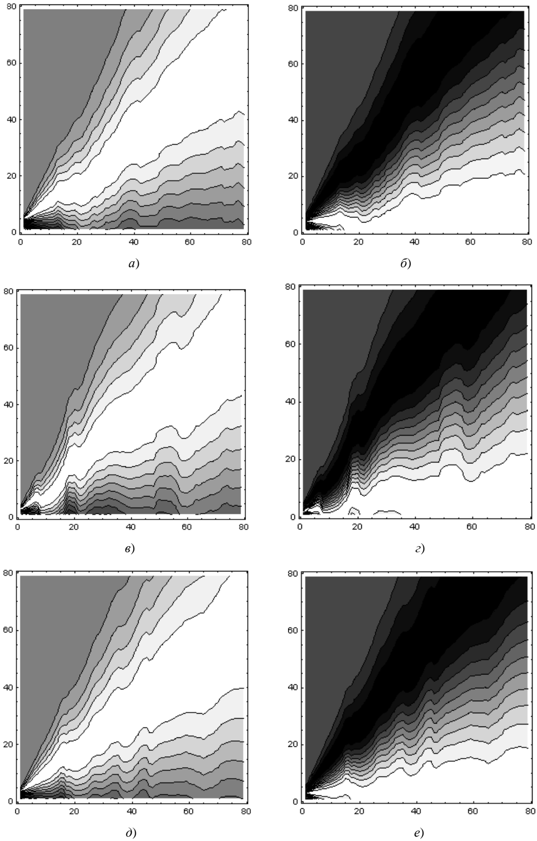
Рис. 5. Картины линий уровней вейвлет-спектров для профилограмм: с 1-го образца – WAVE (a) и MНAT (б); с 2-го образца – WAVE (e) и MНAT (з); с 3-го образца – WAVE (д) и MНAT (e)
