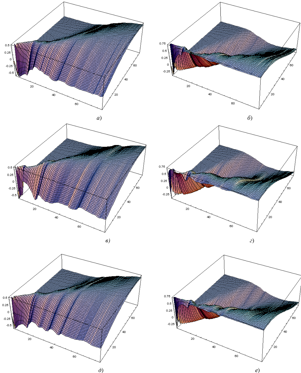
Рис. 4. Поверхности вейвлет-спектров для профилограмм: с 1-го образца – WAVE (a) и МНАТ (б); с 2-го образца – WAVE (в) и МНАТ (г); с 3-го образца – WAVE (д) и МНАТ (е)
