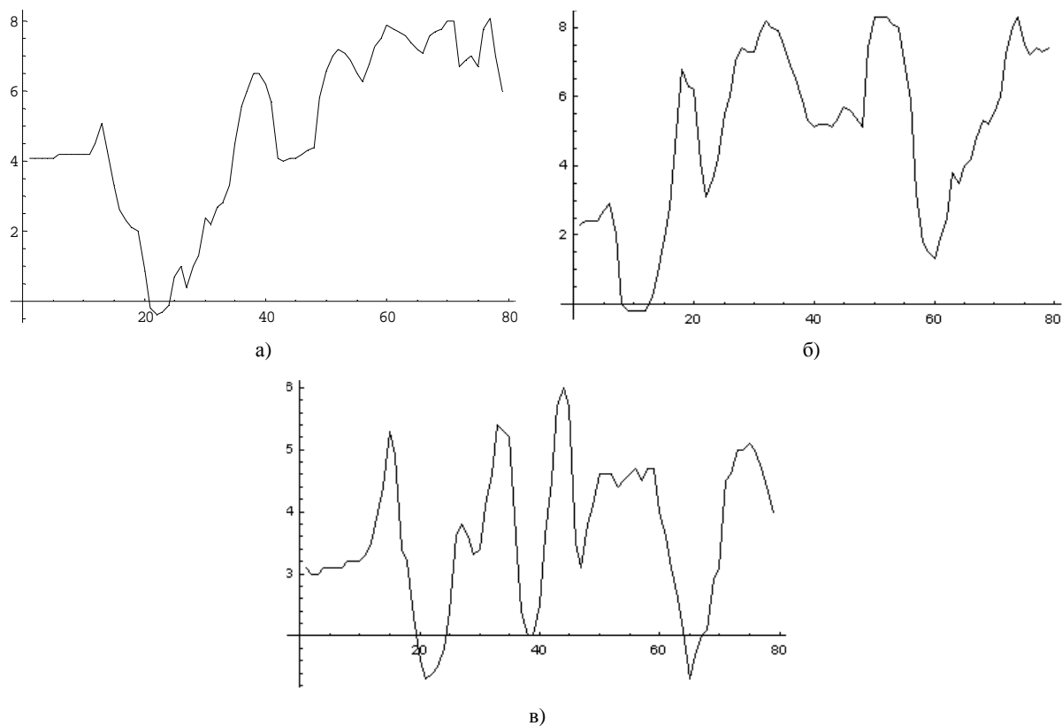
Рис. 3. Профили анализируемых поверхностей трения для образцов с номерами 1(а), 2(б), 3(в)
