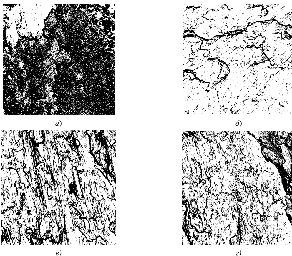
Рис. 1. Рельеф задира образцов с номерами: 2 – 5 % SiC (а); 3 – 2,5 % SiC + 1,25 % C (б); 4 – 2,5 % Al 2 O 3 (в); 5 – 2,5 % Al 2 O 3 + 2,5 % C (г)
