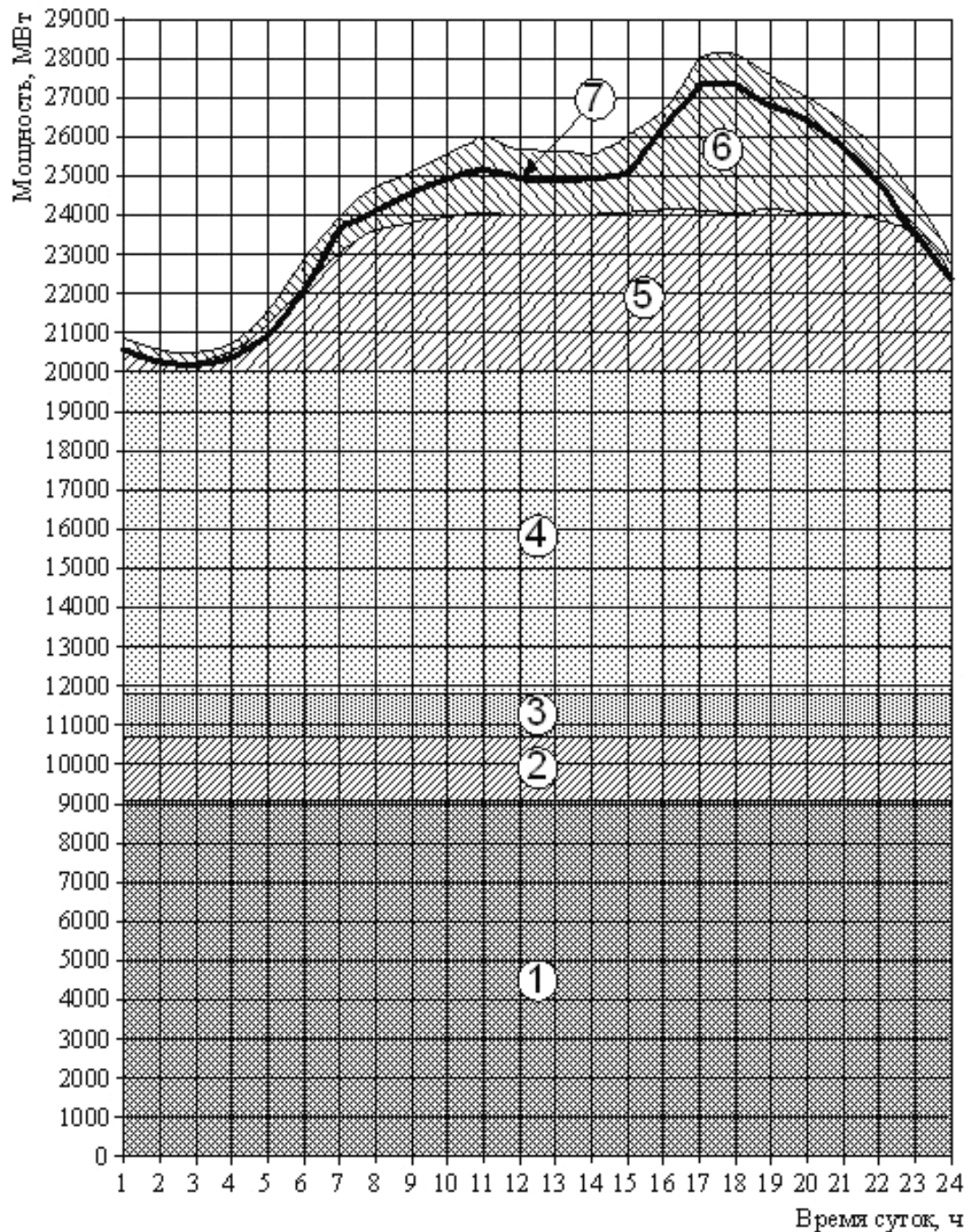
Рис. 5.3. Фактический график базовой и регулирующей мощности в балансе ОЭС Украины за 2 декабря 2002 г.
