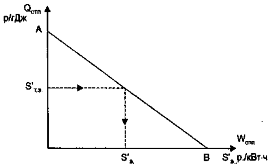
Рис. 5.1. Определение себестоимости электрической и тепловой энергии по методу Гинтера: S'_{тэ} – себестоимость производства единицы тепла в котельной; S'_э – себестоимость единицы электроэнергии; Q_{отп} – количество тепловой энергии, отпускаемой на сторону, ГДж; W_{отп} – количество электрической энергии, отпускаемой на сторону, кВт ч
