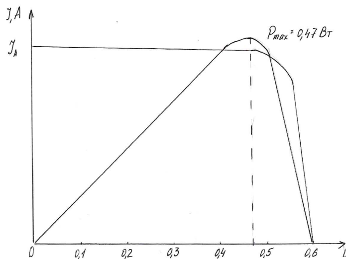
Рис. 4.2 График зависимости выходной мощности от напряжения
