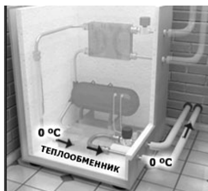
Рис. 2.8. Дросселирование хладона
