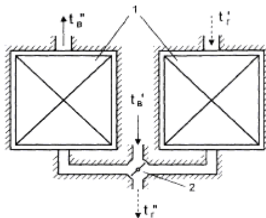
Рис. 6.6. Схема регенератора с неподвижной насадкой – 1; 2 – переключатель направления течения дымовых газов
