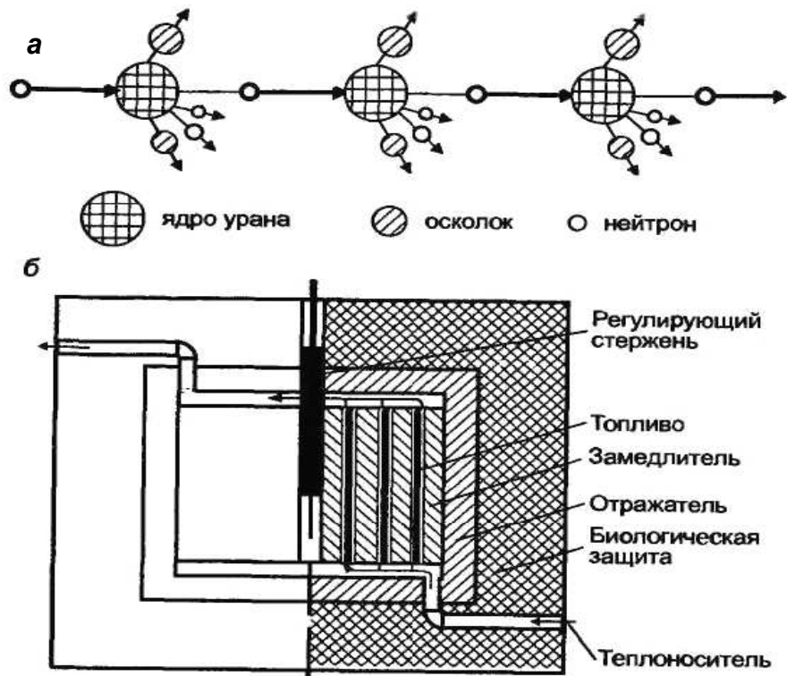
Рис. 3.7. Схема управляемой ядерной реакции (а) и канального ядерного реактора на тепловых нейтронах (б)
