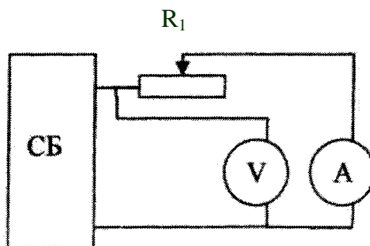
Рис. 4.5. Схема измерения напряжения ВАХ солнечной батареи
