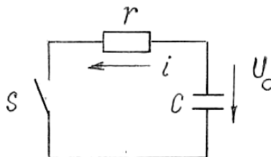
Рис. 5.3. Схема разрядки конденсатора
