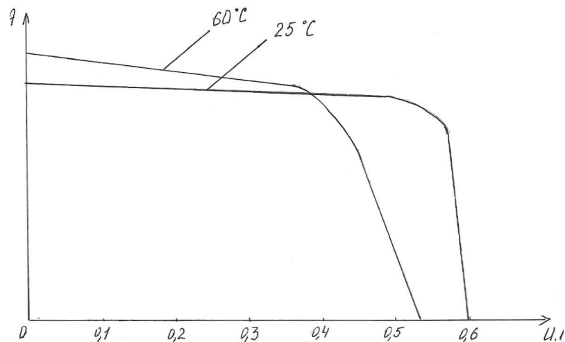
Рис. 4.3. Потери мощности солнечного элемента от напряжения при повышении температуры его поверхности
