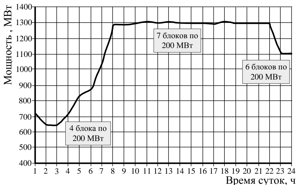
Рис. 5.5. Пример суточного режима работы блочной КЭС
