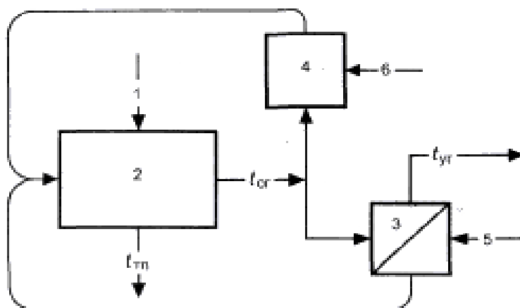
Рис. 6.14. Химическая генерация теплоты при конверсии топлива в среде продуктов сгорания: 1 – технологическое сырье; 2 – точка промышленной печи; 3 – воздухоподогреватель; 4 – реактор для конверсии топлива отходящими газами; 5 – холодный воздух; 6 – топливно-природный газ
