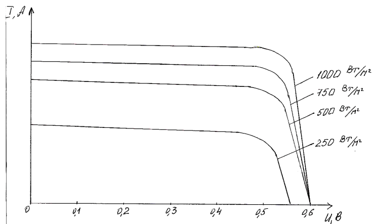
Рис. 4.1. Зависимость тока и напряжения солнечной батареи от освещения
