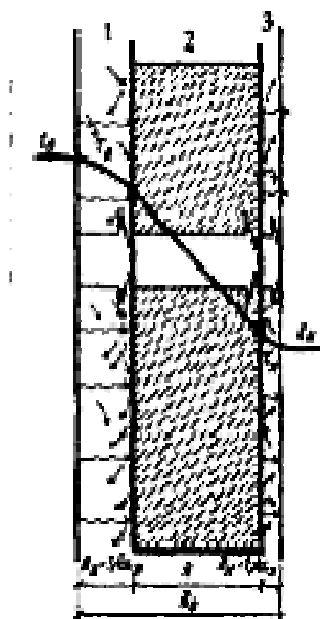
Рис. 9.4. Сопротивление теплопередаче стены: 1 – теплообмен у внутренней поверхности стены, 2 – теплопередачи через толщу ограждения, 3 – теплообмен у наружной поверхности стены; \alpha_v – коэффициент теплоотдачи внутренней поверхности ограждающей конструкции, Вт/(м 2 ·К), \alpha_{нз} – коэффициент теплоотдачи наружной поверхности ограждающей конструкции для зимних условий, Вт/(м 2 ·К)
