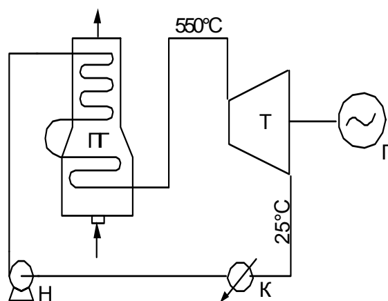
Рис. 3.2. Принципиальная тепловая схема КЭС. Основное оборудование: котел-парогенератор – ПГ, турбина – Т, генератор – Г, конденсатор – К, насос – Н
