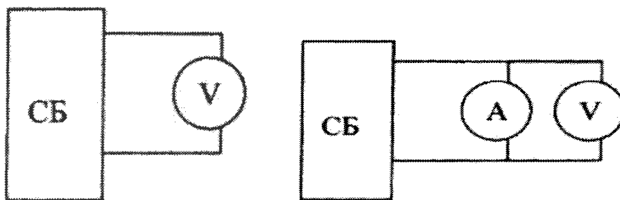
Рис. 4.4. Схемы измерения напряжения холостого хода – U_{XX} и тока короткого замыкания – I_{KЗ} солнечной батареи
