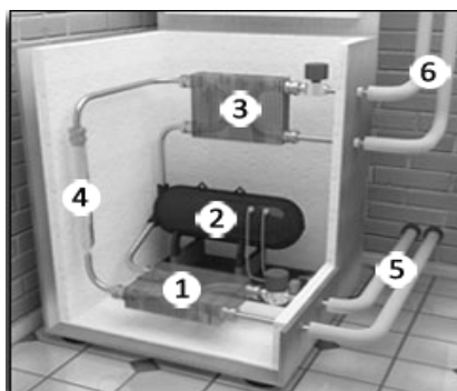
Рис. 2.4. Основные узлы теплового насоса
