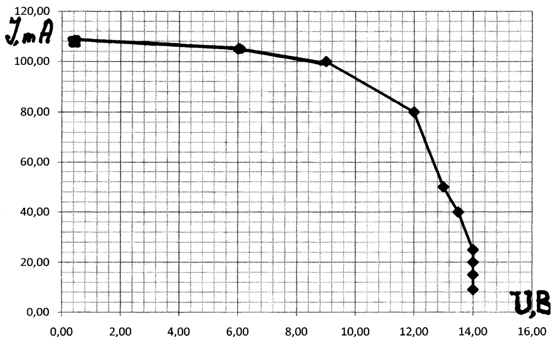
Рис. 4.7. Вольт-амперная характеристика солнечной батареи
