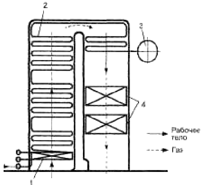
Рисунок 6.8. Схема котла утилизатора: 1 – пароперегреватель, 2 – испарительные пакеты, 3 – барабан – сепаратор, 4 – экономайзер
