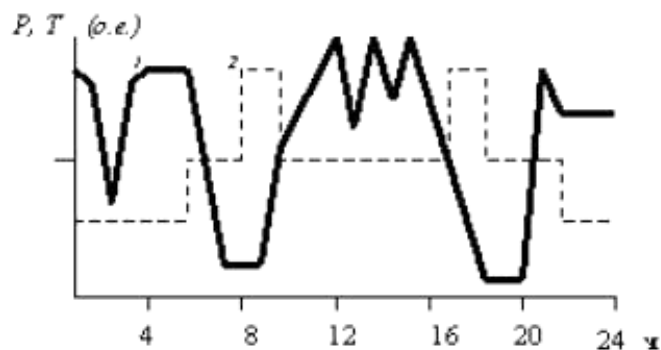
Рис. 5.7. Суточное электропотребление (1) и тариф, дифференцированный по времени суток (2), для электрометаллургического завода в Германии
