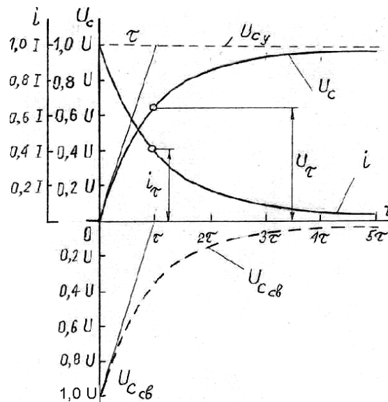
Рис. 5.2. Изменение напряжения и тока от времени зарядки конденсатора
