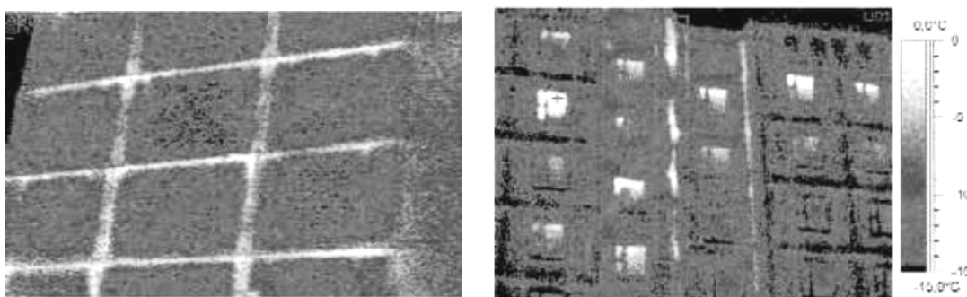
Рис. 7.4. Брак в выполнении плоского вертикального стыка между стеновыми панелями
