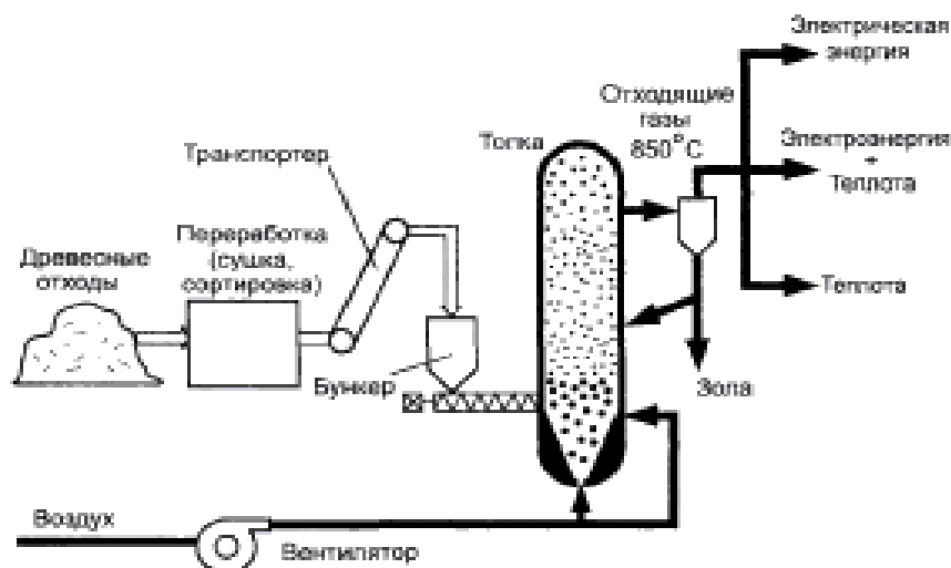
Рис. 6.1. Схема использования древесных отходов для получения энергии
