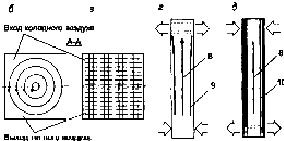
Рис. 6.11. Схема утилизатора теплоты вытяжного воздуха (а) с регенеративной вращающейся насадкой (б) и тепловыми трубами (в) и схемы термосифона (г) и тепловой трубы (д): 1 – вращающаяся теплоаккумулирующая насадка; 2 – корпус; 3 – вытяжной воздухопровод; 4 – приточный воздухопровод; 5 – вытяжной вентилятор; 6 – приточный вентилятор; 7 – подогреватель воздуха; 8 – пар; 9 – пленка конденсата; 10 – капилляр
