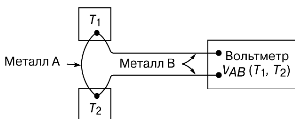
Рис. 6.2. Эффект Т. Зеебека
