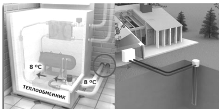
Рис. 2.5. Схема забора тепла Земли
