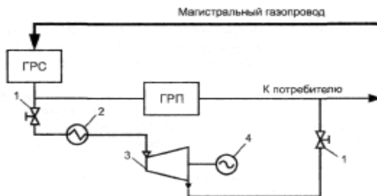
Рис. 6.12. Утилизация энергии избыточного давления в системе распределения природного газа: 1 – клапаны; 2 – подогреватель; 3 – турбина; 4 – электрогенератор
