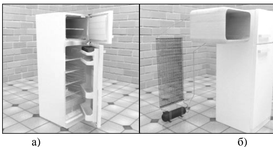
Рис. 2.1. а) Современный холодильник; б) Тепловой насос. Отдельно показаны трубчатые панели конденсатора, испарительная камера, компрессор
