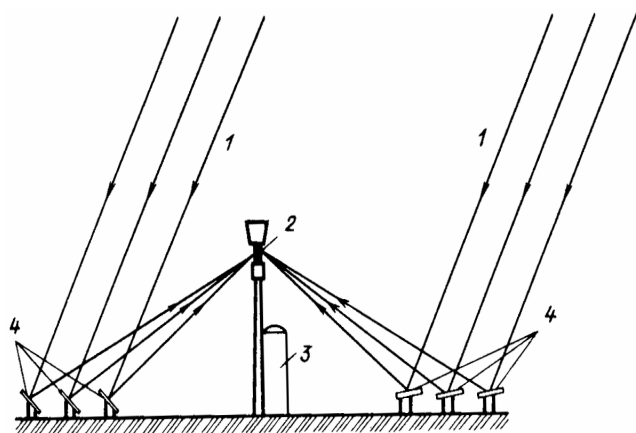
Рис. 4.2. Схема работы Крымской экспериментальной солнечной электростанции мощностью 5000 кВт: 1 – солнечные лучи; 2 – парогенератор-гелиоприемник; 3 – пароводяной аккумулятор энергии вместимостью 500 м; 4 – гелиостаты с площадью зеркал 25 м 2 (общее их число 1000 штук).
