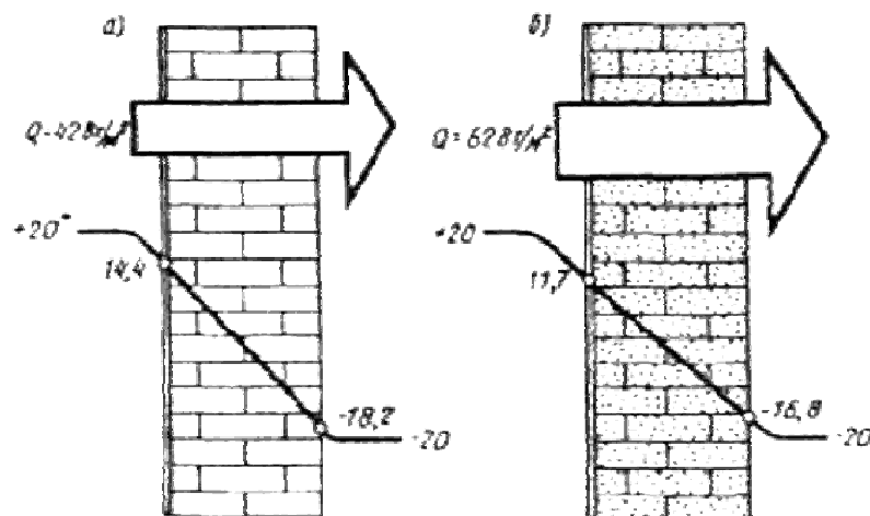
Рис. 9.3. Влияние влажности материала на теплозащитные свойства кирпичной стены: а) – сухая стена, влажность материала 5 %; б) – сырая стена, влажность материала 15 %
