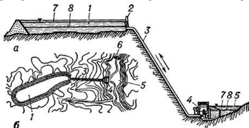
Рис. 5.6. Схема ГАЭС (а – вертикальный разрез; б – план): 1 – верхний аккумулятирующий бассейн; 2 – водоприемник; 3 – напорный водовод; 4 – здание ГАЭС; 5 – нижнее питающее водохранилище; 6 – плотина с водосбросом; 7 – нормальный подпорный уровень воды; 8 – уровень сработки
