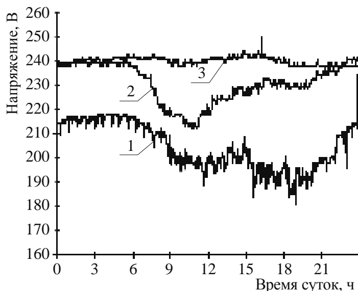
Рис. 5.4. Примеры суточных циклов изменения напряжения в сети
