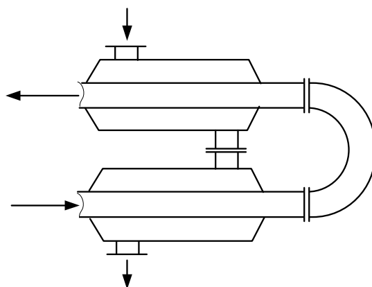
Рис. 6.2. Рекуперативный теплообменник типа «труба в трубе»
