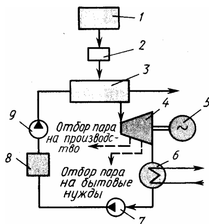
Рис. 3.1. Принципиальная схема КЭС, работающей на угле
