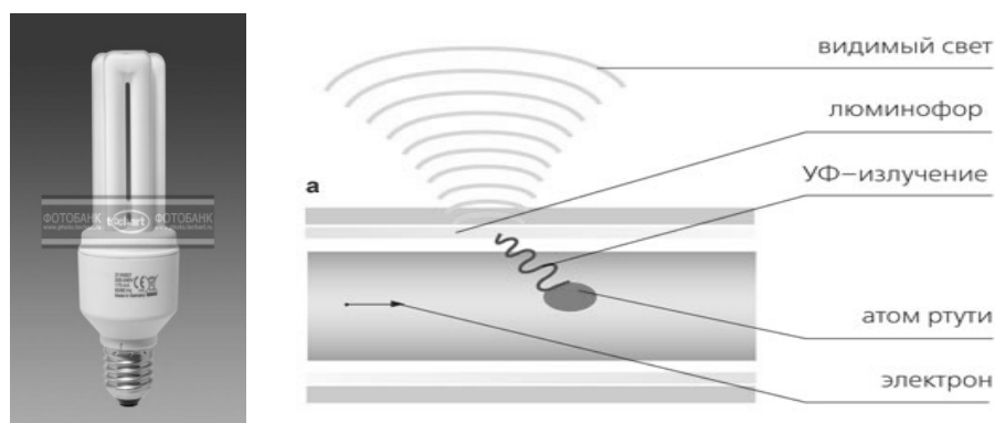
Рис. 7.1. Устройство и принцип работы люминесцентной лампы
