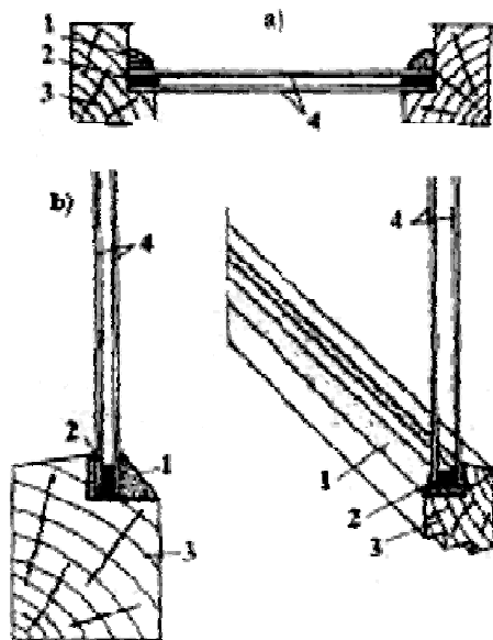
Рис. 9.5. Установка дополнительного стекла на картонную или резиновую прокладку: а) – вид в плане, б) – вид в разрезе; 1 – замазка, 2 – резиновая или картонная прокладка, обмазанная краской, 3 – переплет, 4 – скрепленные между собой стекла.
