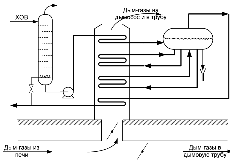
Рис. 6.4. Принципиальная схема работы котла-утилизатора пакетно-конвективного типа
