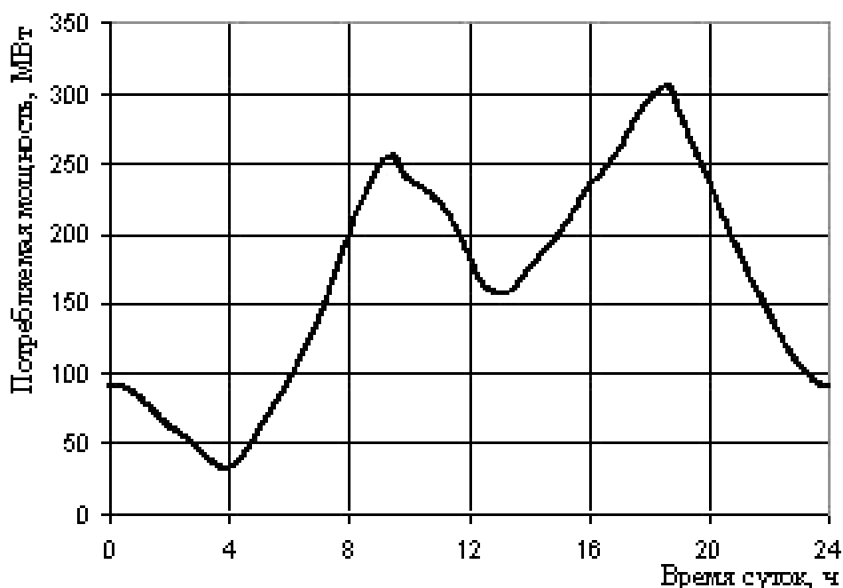
Рис. 5.2. Пример графика потребления электроэнергии в течение зимних суток в большом городе
