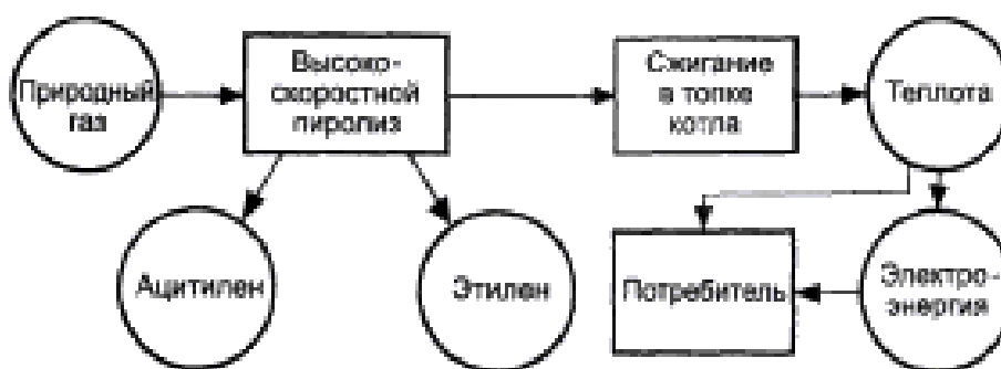
Рис. 6.13. Схема энерготехнологических процессов при использовании природного газа
