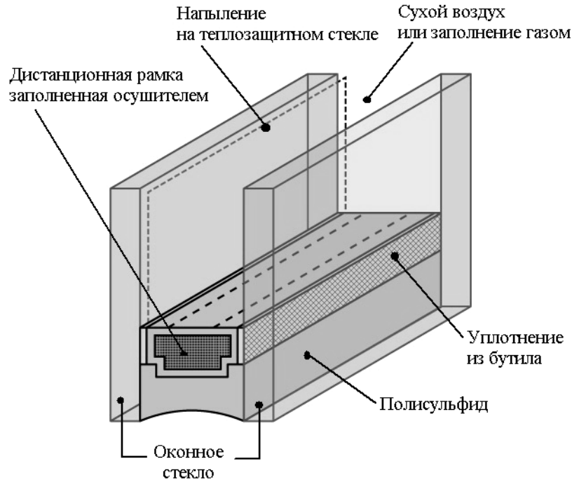
Рис. 9.7. Схема стеклопакета
