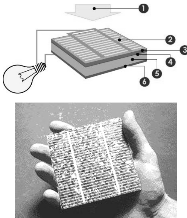
Рис. 4.3. Структура солнечного элемента: 1. – свет (фотоны); 2. – фронтальный контакт; 3. – просветляющий слой; 4. – слой р-п перехода; 5. – слой кремния; 6. – задний контакт. Внешний вид кремниевого солнечного элемента
