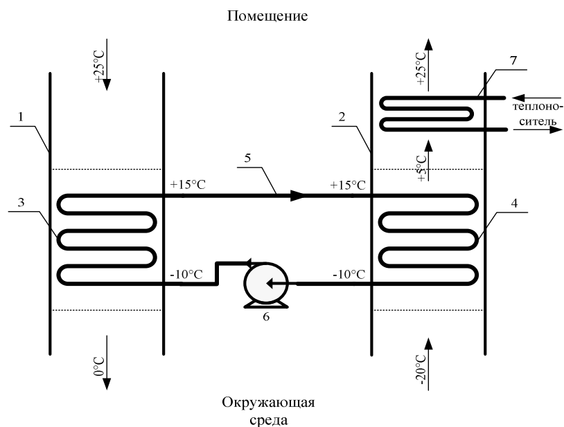
Рис. 6.5. Схема теплообмена с промежуточным циркулирующим теплоносителем:
