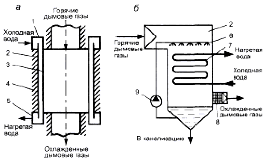
Рис. 6.7. Радиационный рекуператор кольцевой (а) и контактный теплообменник с активной насадкой (б): 1 – раздающий коллектор, 2 – корпус, 3 – поверхность нагрева, 4 – тепловая изоляция, 5 – коллектор, 6 – система орошения, 7 – активная насадка, 8 – сепарационное устройство, 9 – насос системы орошения
