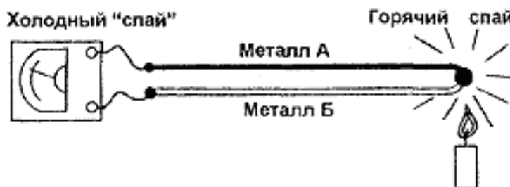
Рис. 6.5. Термопара
