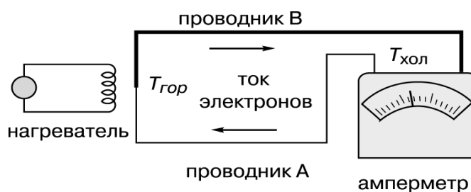
Рис. 6.1. Появление электрического тока в цепи, вызванного нагревом спаев проводников А и В
