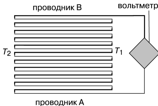
Рис. 6.6 Термобатарея
