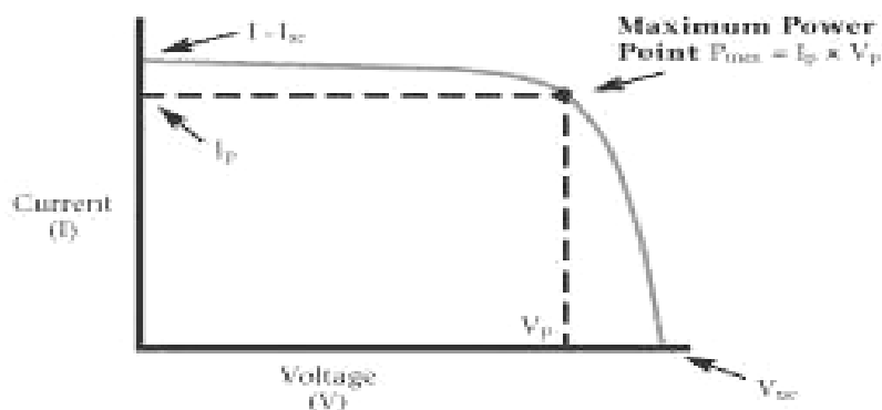
Рис. 4.4. Вольтамперная характеристика солнечного элемента
