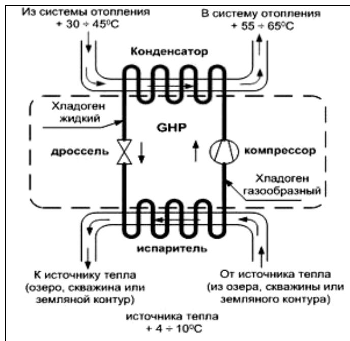
Рис. 2.2. Принципиальная схема действия теплового насоса
