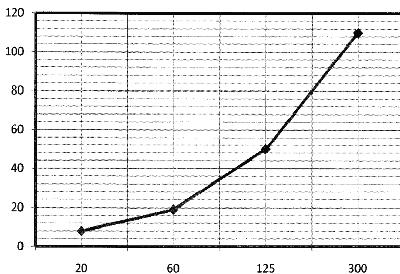
Рис. 4.6. График зависимости тока СБ от освещенности
