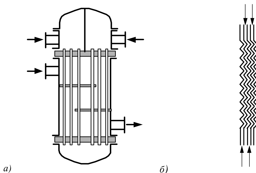
Рис. 6.3. а) Многоходовой кожухотрубчатый теплообменник; б) Пластинчатые теплообменники
