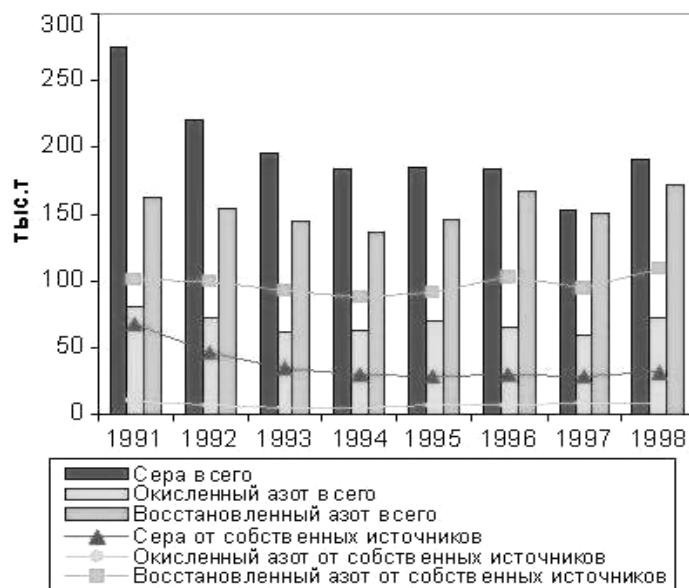
Рис. 11.4. Динамика выпадения закисляющих соединений на территории Беларуси
