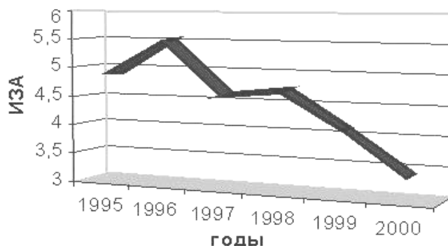
Рис. 11.7. Динамика индекса загрязнения атмосферы в городах Республики Беларусь за период 1996 – 2000 гг.
