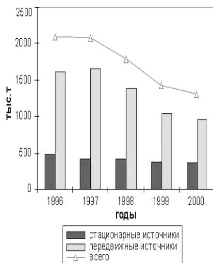
Рис. 11.2. Динамика выбросов в атмосферу на территории Беларуси
