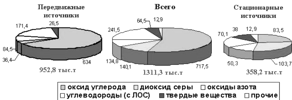
Рис. 11.1. Структура выбросов в атмосферу на территории Беларуси в 2000 г.
