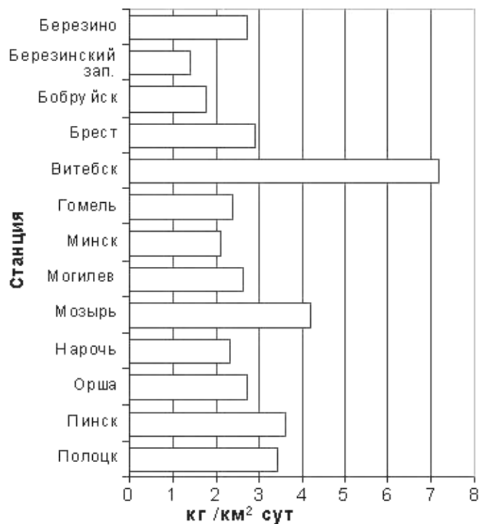
Рис. 11.6. Средняя интенсивность влажного выпадения соединений серы в 1996 – 2000 гг.
