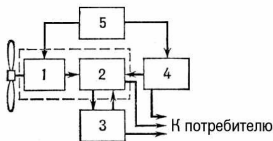
Рис. 4.1. Принципиальная схема ветряной электрической станции: 1 – генератор электрического тока; 2, 3, 4 – аккумуляторные батареи; 5 – контрольно-измерительное устройство
