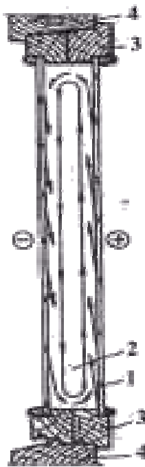
Рис. 9.2. Передача тепла конвекцией в межстекольном пространстве оконного блока со спаренным остеклением: 1 – стекло, 2 – воздушная прослойка, 3 – переплет, 4 – оконная коробка
