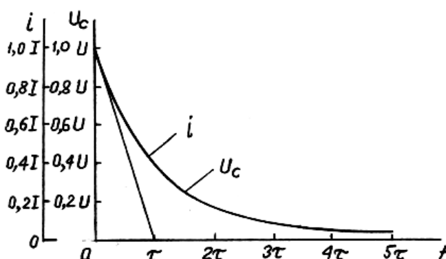
Рис. 5.4. Изменение напряжение и тока во время разрядки конденсатора
