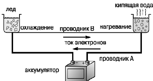
Рис. 6.3. Эффект Ж.Ш. Пельтье
