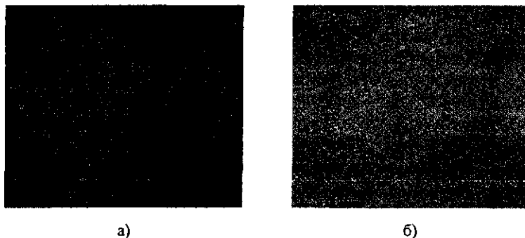
Фрагменты поверхностей плит: а – использована традиционная технология; б – использован состав БПС
