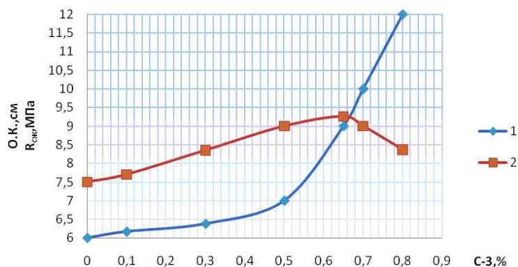
Рис. 2. Зависимость свойств бетонной смеси и бетона от количества добавки С-3: 1 – зависимость С-3 – ОК; 2 – зависимость С-3 – R сж (прочность в возрасте 3-х суток)
