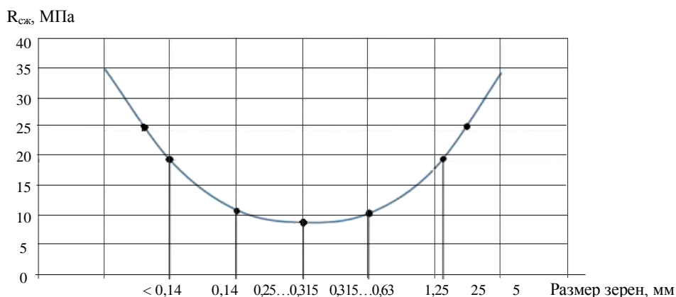
Рис. 3. Зависимость прочности бетона на стекольном заполнителе от размера зерен в возрасте 28 суток
