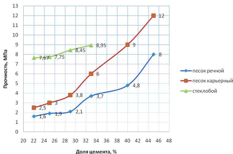
Рис. 1. Зависимость прочности бетона от доли цемента в смеси: 1 – стеклобой; 2 – песок карьерный; 3 – песок речной
