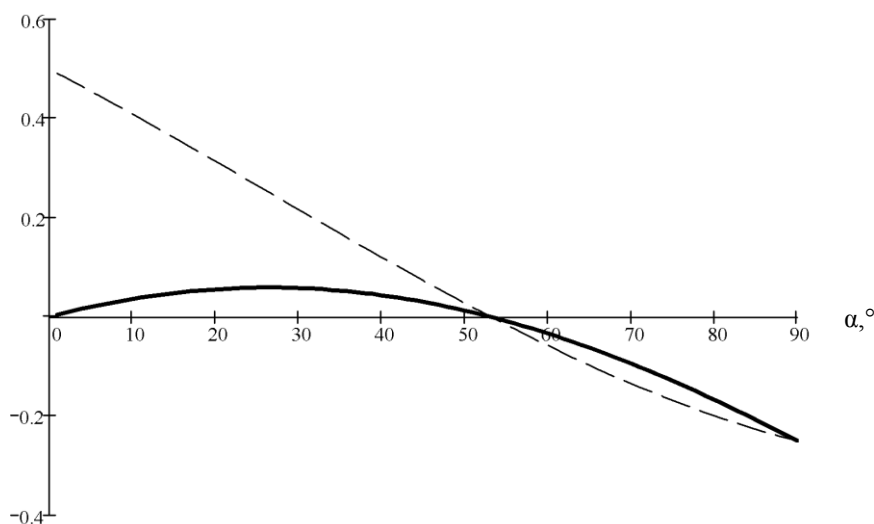
Рис. 9. Характер изменения относительных составляющих сил Q , обеспечивающих взаимодействие зерна с шаржируемой поверхностью: Q_{\text{г}} / N_1 (штриховая линия); Q_{\text{в}} / N_1 (сплошная толстая линия) в диапазоне изменения угла \alpha от 0 до 90° ( \mu_1 = 0,5 , \mu_2 = 0,3 ) при введении в зону шаржирования ультразвуковых колебаний
