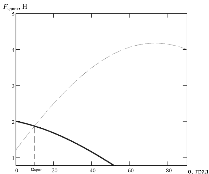
Рис. 5. Характер изменения сил, действующих на зерно в горизонтальном направлении и стремящихся сдвинуть его от деформирующего инструмента (штриховая тонкая линия) и к деформирующему инструменту (сплошная линия) в диапазоне изменения угла \alpha от 0 до 90^\circ ( \mu_1 = 0,5 , \mu_2 = 0,3 , N_2 = 4 Н)
