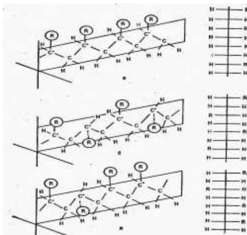
Рис. 2.2 Различные конфигурации полимеров типа -\text{CHR}-\text{CH}_2- (а- изотактическая, б – синдиотактическая, в – атактическая).
