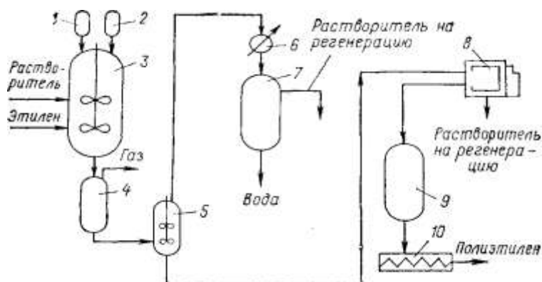
Рис. 2.9 Технологическая схема получения ПЭНД суспензионной полимеризацией на высокоактивных катализаторах:
