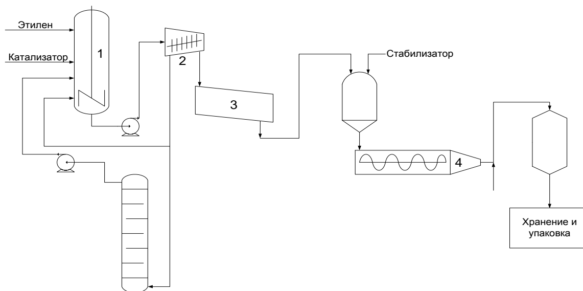
Рис. 2.11 – Схема процесса СХ
