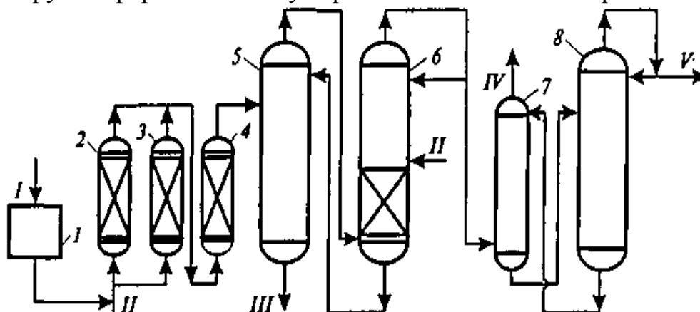
Рис. 7.1 Принципиальная схема блока синтеза МТБЭ и регенерации метанола:
