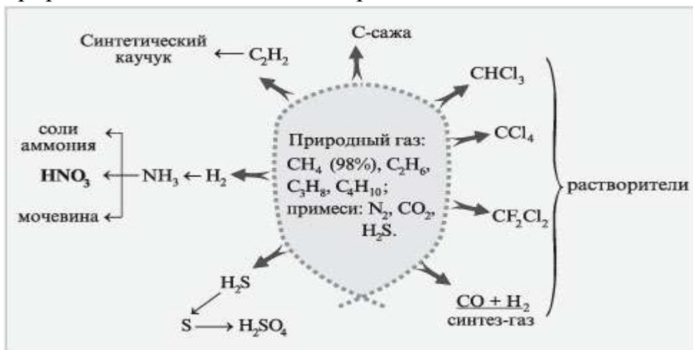
Рис. 1.1 Состав природного газа и вещества, получаемые на его основе
