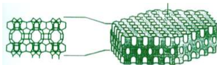
Рисунок 3.3 - Структура кристаллической решетки цеолита типа MCM-22
