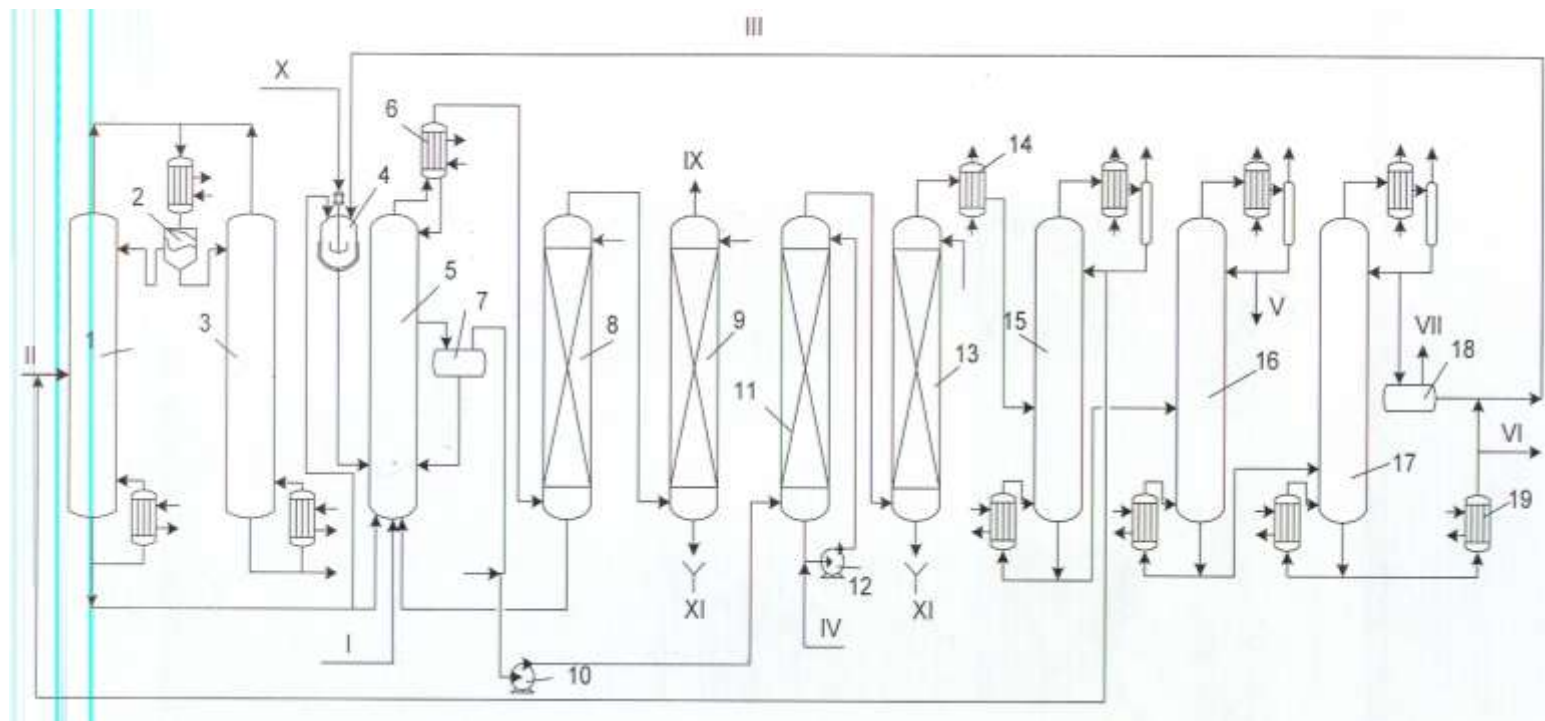
Рис. 3.1 - Технологическая схема производства этилбензола с использованием катализатора на основе \text{AlCl}_3 :
