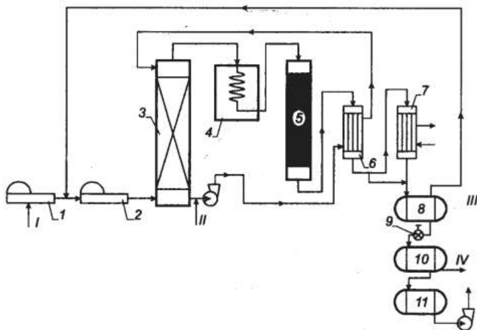
Рис. 6.2 Технологическая схема прямой гидратации этилена с рекуперацией тепла потоков
