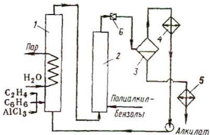
Рис. 3.2- Технологическая схема реакторного узла жидкофазного алкилирования (фирма «Monsanto»):
