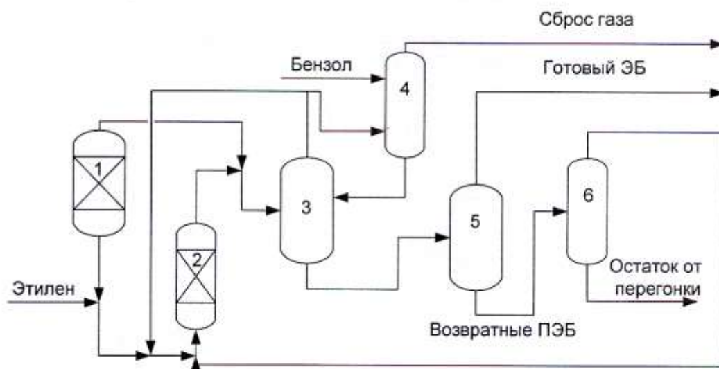
Рисунок 3.4 - Технологическая схема процесса фирмы «Mobil-Badger»:
