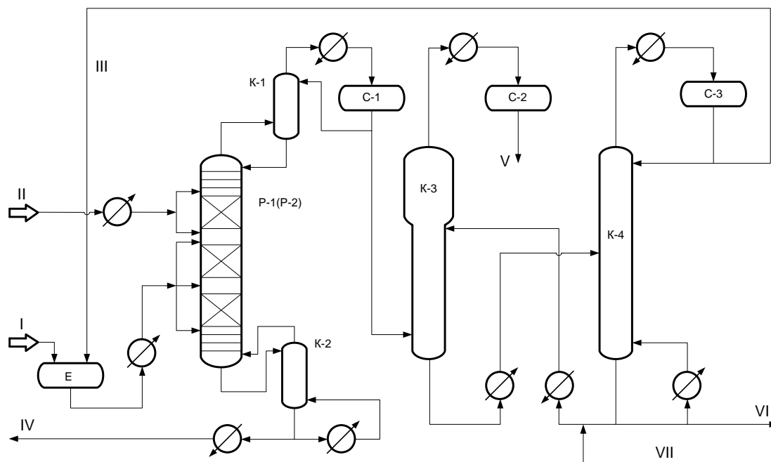
Рис. 7.2 Принципиальная технологическая схема установки получения метилтретбутилового эфира:
