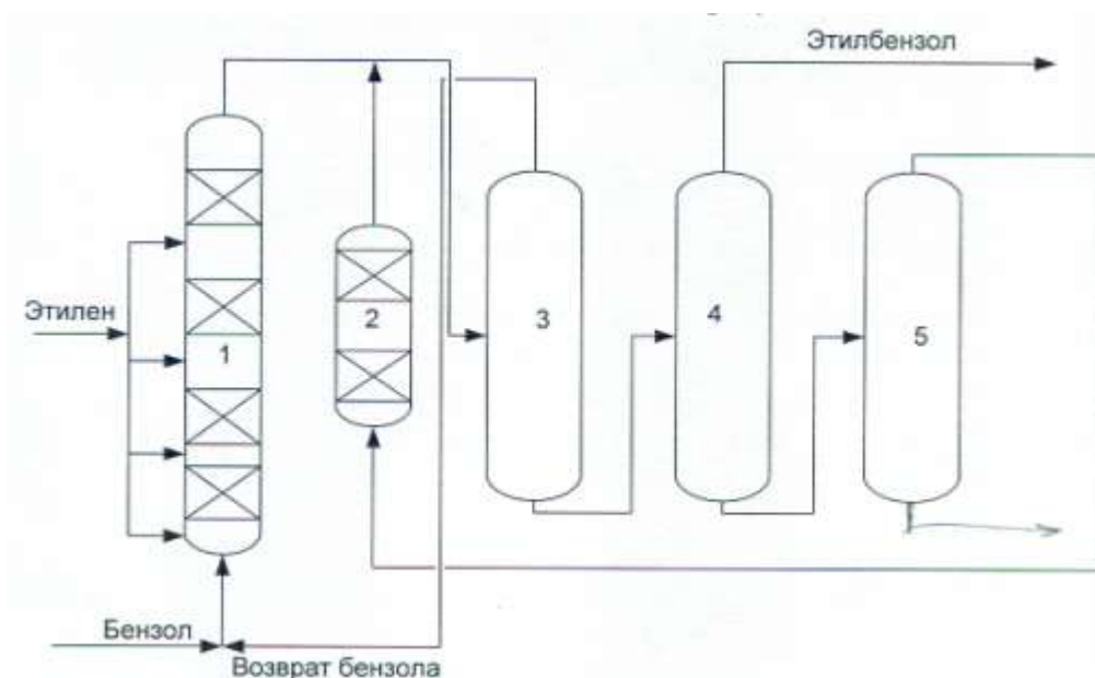
Рисунок 3.5 - Технологическая схема процесса алкилирования фирмы Lummus/UOP EBOne:
