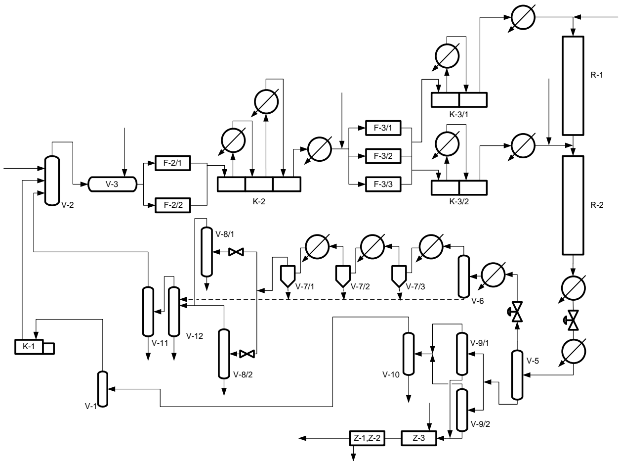
Рис.2.7 Технологическая схема получения полиэтилена высокого давления
