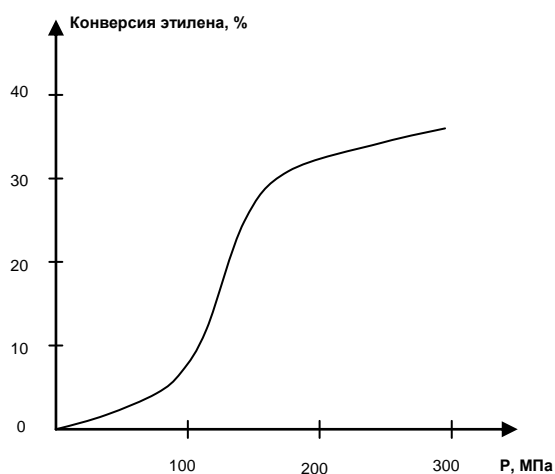
Рис. 2.3 Зависимость конверсии этилена от давления: температура 190 °С; концентрация кислорода 0,0455%; время пребывания в реакторе 3 мин
