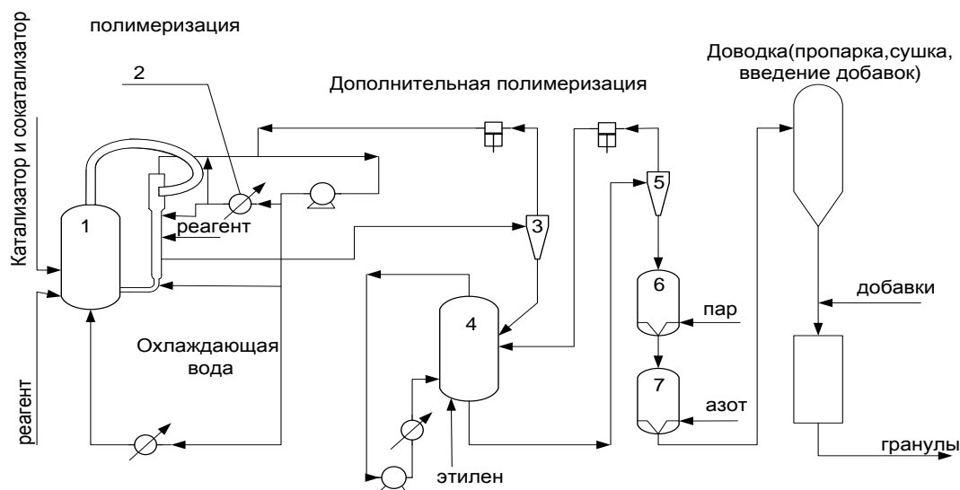
Рис. 2.16 Получение полимеров на базе полипропилена с использованием технологии Spherizone.
