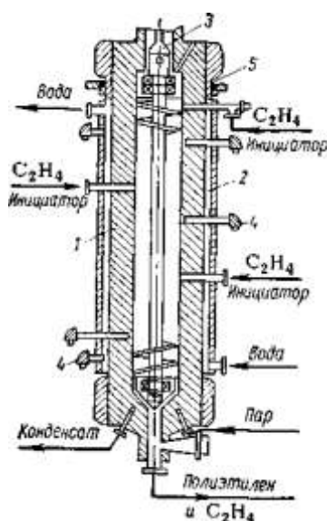
Рис. 2.5 Реактор с перемешивающим устройством:
