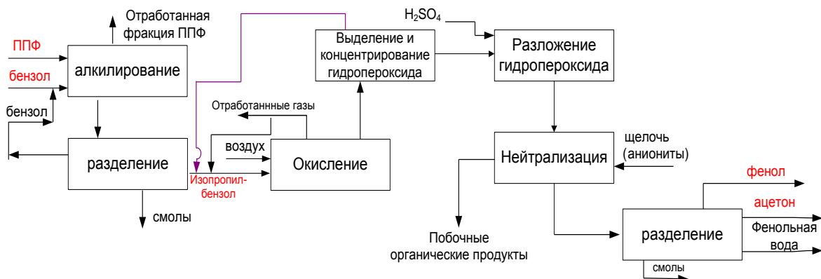
Рис. 4.6 Поточная схема кумольного метода получения фенола и ацетона
