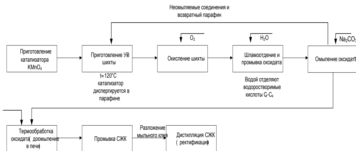
Рис. 4.3 Поточная схема производства синтетических жирных кислот.
