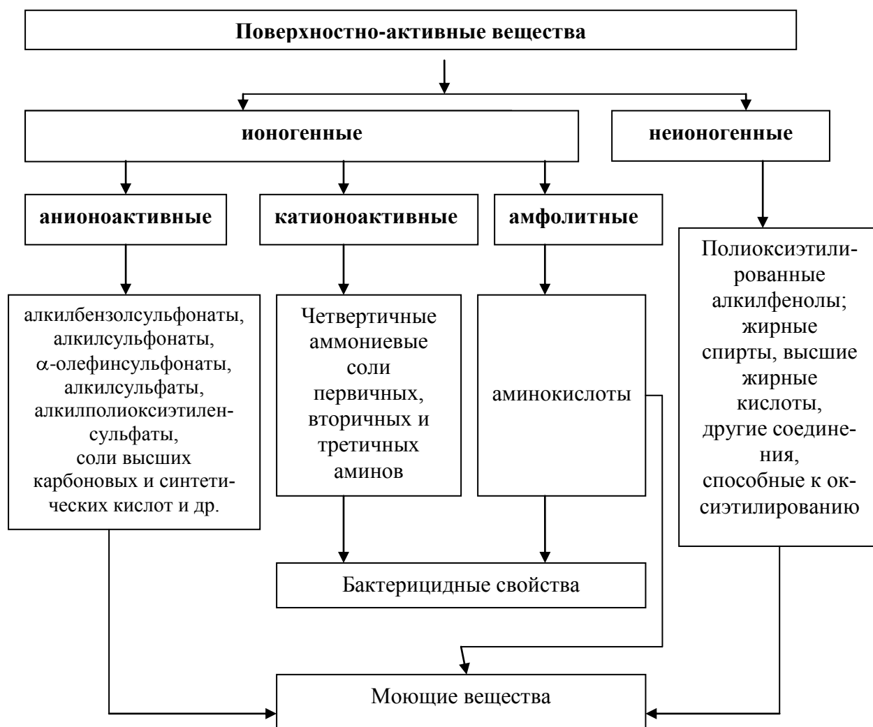
Рис. 5.1 Классификация ПАВ
