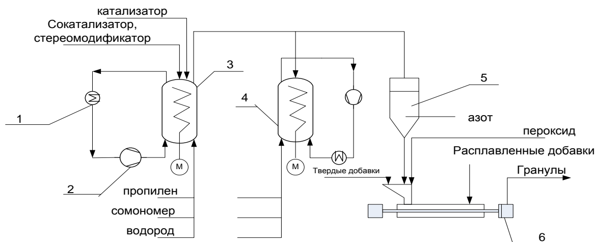
Рис. 2.15 Схема процесса получения полипропилена Novolen (с использованием металлоценовых катализаторов).
