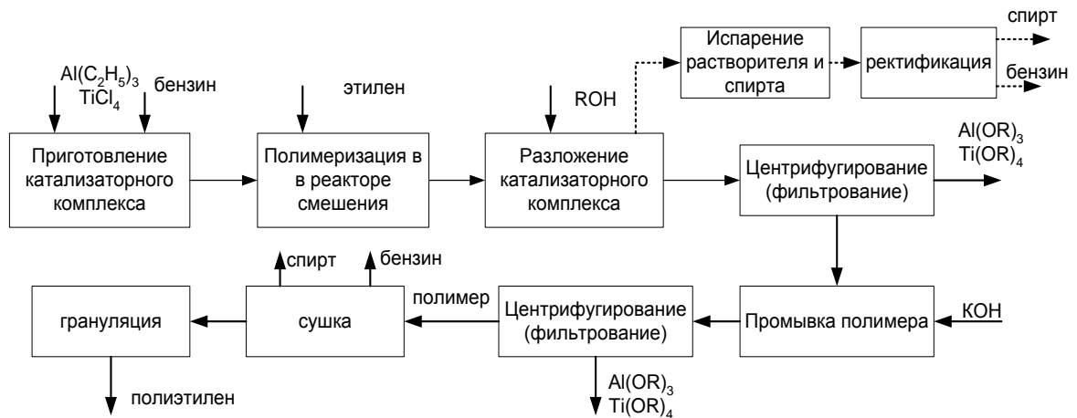
Рис. 2.8 Поточная схема получения полиэтилена высокой плотности при низком давлении
