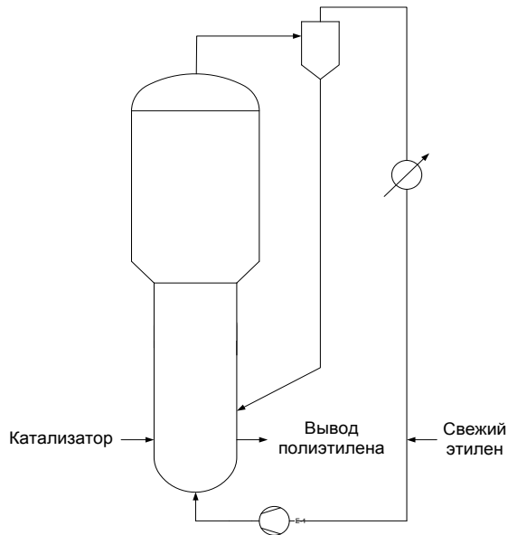
Рис. 2.12 – Принципиальная схема работы реактора газофазной полимеризации
