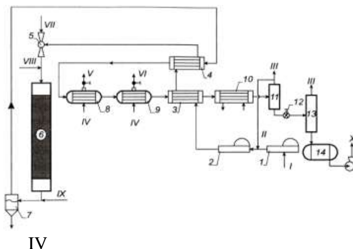
Рис. 6.1. Технологическая схема прямой гидратации этилена
