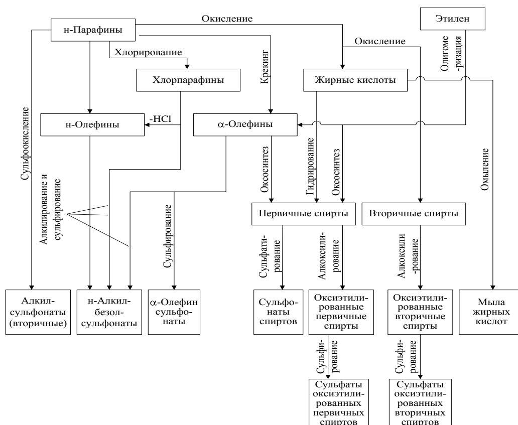
Рисунок 5.3– Схема переработки нефтехимического сырья для получения биоразлагаемых ПАВ
