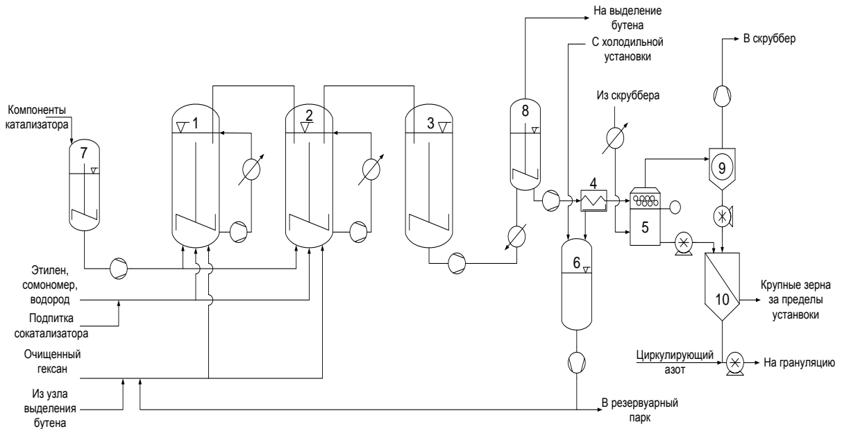
Рис. 2.10 – Схема процесса Hostalen
