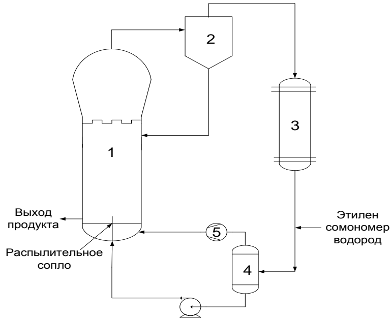
Рис. 2.13 Схема процесса Innoven:
