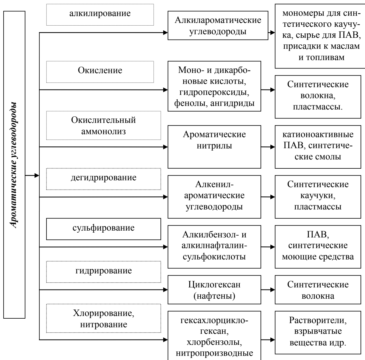
Рис. 1.5 Основные направления химической переработки ароматических углеводородов
