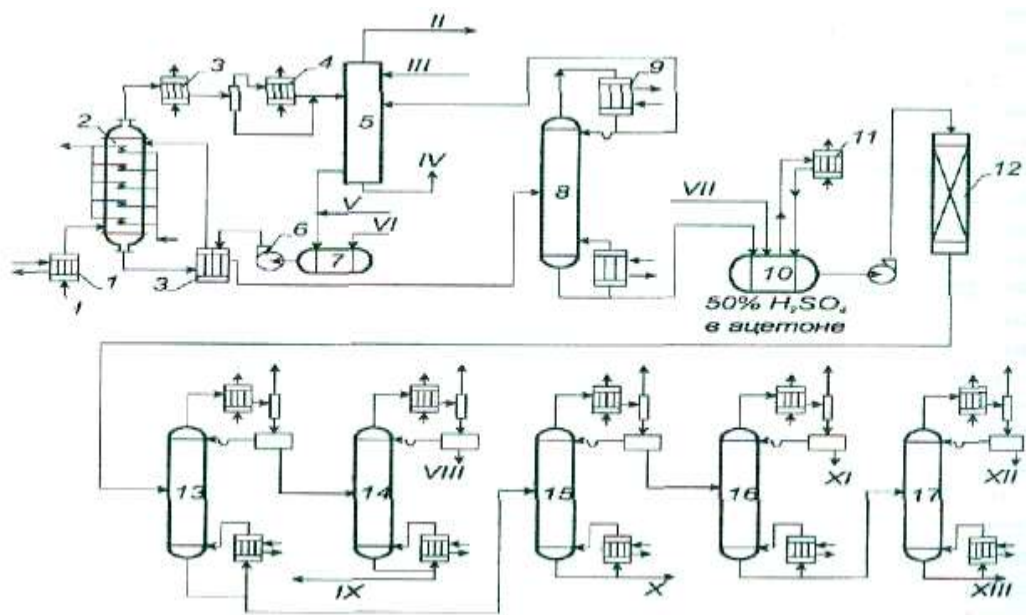
Рис. 4.5. Технологическая схема производства фенола и ацетона кумольным методом:
