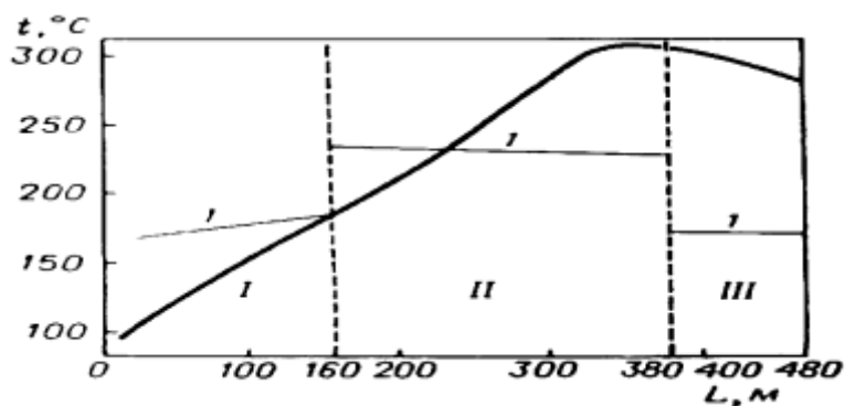
Рис. 2.4 Температурный профиль полимеризации в трубчатом реакторе. I – участок нагрева; II – участок реакции; III – участок охлаждения; 1 – температура теплоносителя
