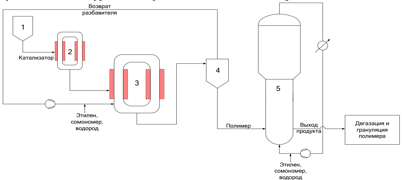
Рис. 2.14 – Схема процесса Vorstar:
