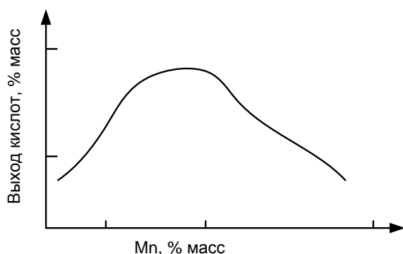
Рис. 4.2 Влияние количества катализатора ( KMnO_4 ) на выход кислот
