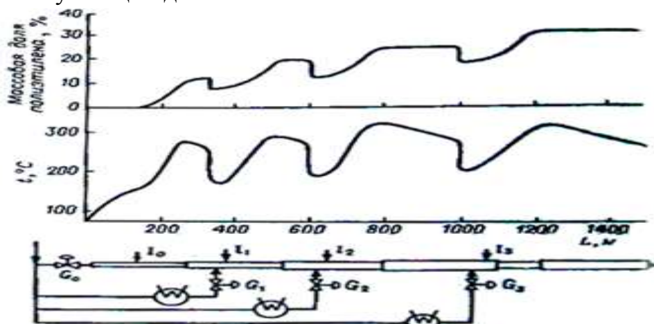
Рис. 2.6 Схема трубчатого реактора с боковыми вводами этилена, профиль температур и конверсия по длине реактора: I_0 - I_3 – подача инициатора; G_0 - G_3 - подача этилена.
