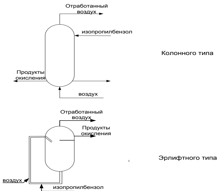
Рис. 4.4 Реакторы процесса окисления
