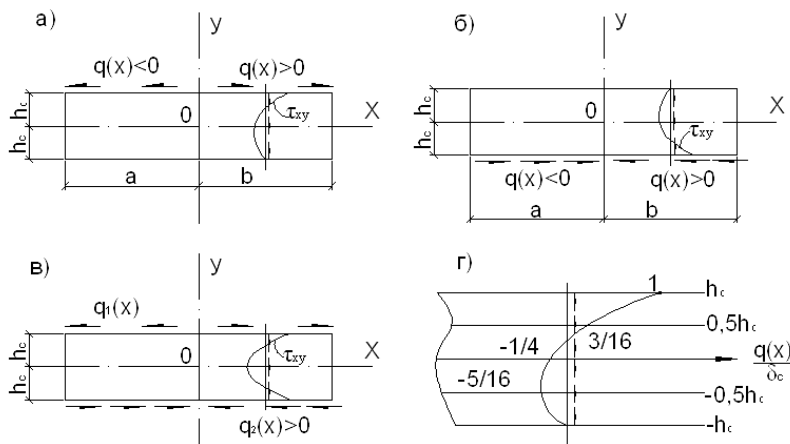
Рис. 2. Эпюры касательных напряжений полосы тонкостенного стержня
