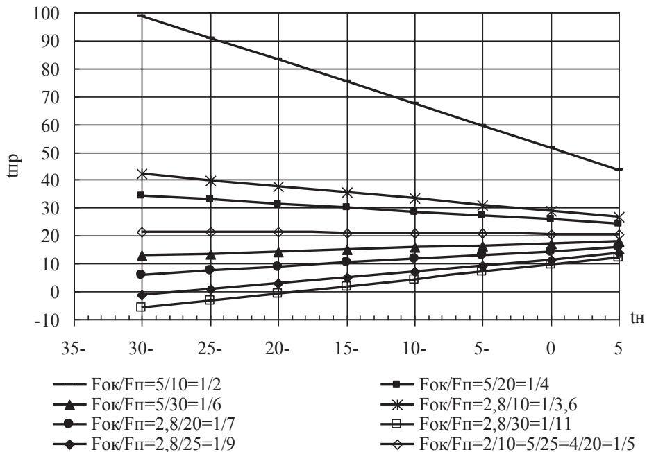
Рисунок 1 - Интенсивность нагрева приточного наружного воздуха t_{np} за счет рекуперативного теплообмена двухслойного вентилируемого оконного стеклопакета при инфильтрации в зависимости от соотношения F_{ок}/F_n и в соответствии с действующей нормативной базой теплотехнического расчета наружных ограждений
