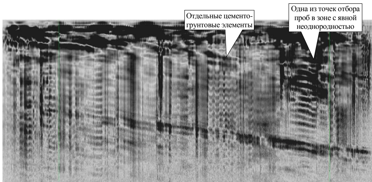
Рисунок 4 – Георадарный профиль экранированной антенны с частотой 100 МГц
