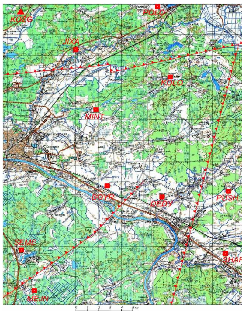
Расположение тектонических разломов и пунктов ГДП «Полоцкая ГЭС»: DEDY, BOYR, SEME, MEJN – пункты, контролирующие Туровлянский разлом; POLO, KOLO, JIXA. MINT– Полоцкий; DEDY, KOLO, PUSH, SHAR – Чашникский
