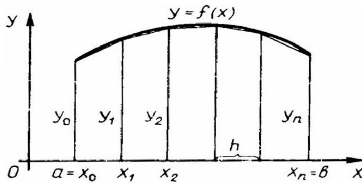
Рис. 3.12. Метод трапеций
