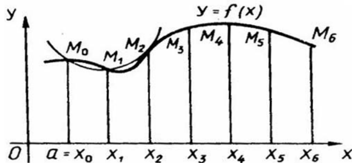
Рис. 3.13. Метод парабол
