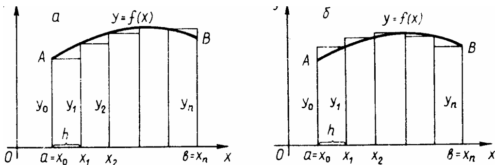
Рис. 3.11. Метод прямоугольников
