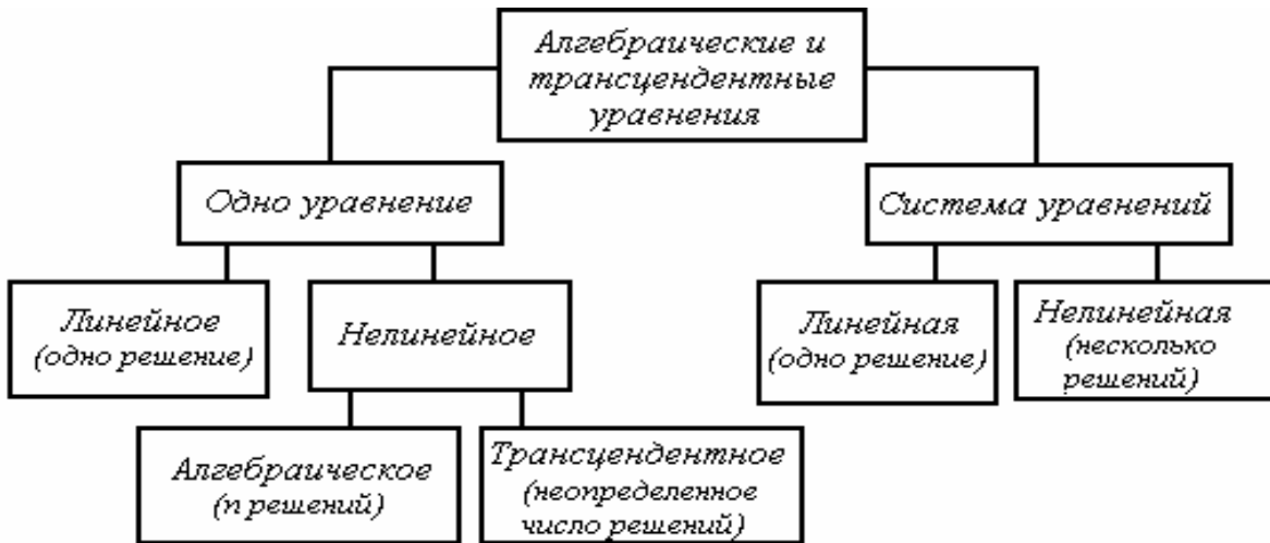
Рис. 3.9. Классификация уравнений
