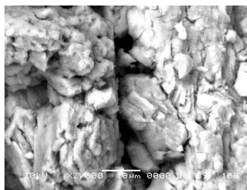
Рисунок 5 – Электронная микроскопия частиц наполнителя (увеличение 2000 крат)
