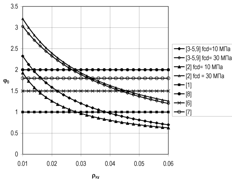
Рис. 1. Зависимость коэффициента \varphi_0 от коэффициента \rho_{xy} по [1 – 9]
