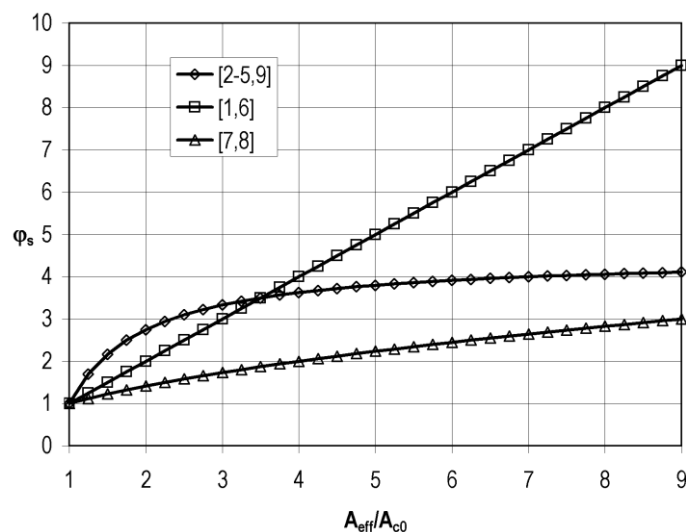
Рис. 2. Зависимость коэффициента \varphi_s от отношения A_{eff}/A_{c0} по [1 – 9]
