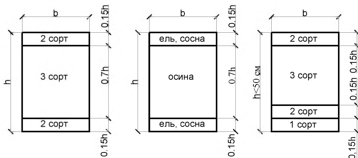
Рис. 11.4. Варианты компоновки поперечного сечения доштокклееных балок
