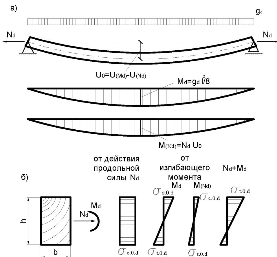
Рис. 5.6. Сжато-изгибаемый элемент: а – схема работы и эпюры изгибающих моментов; б – эпюры нормальных напряжений
