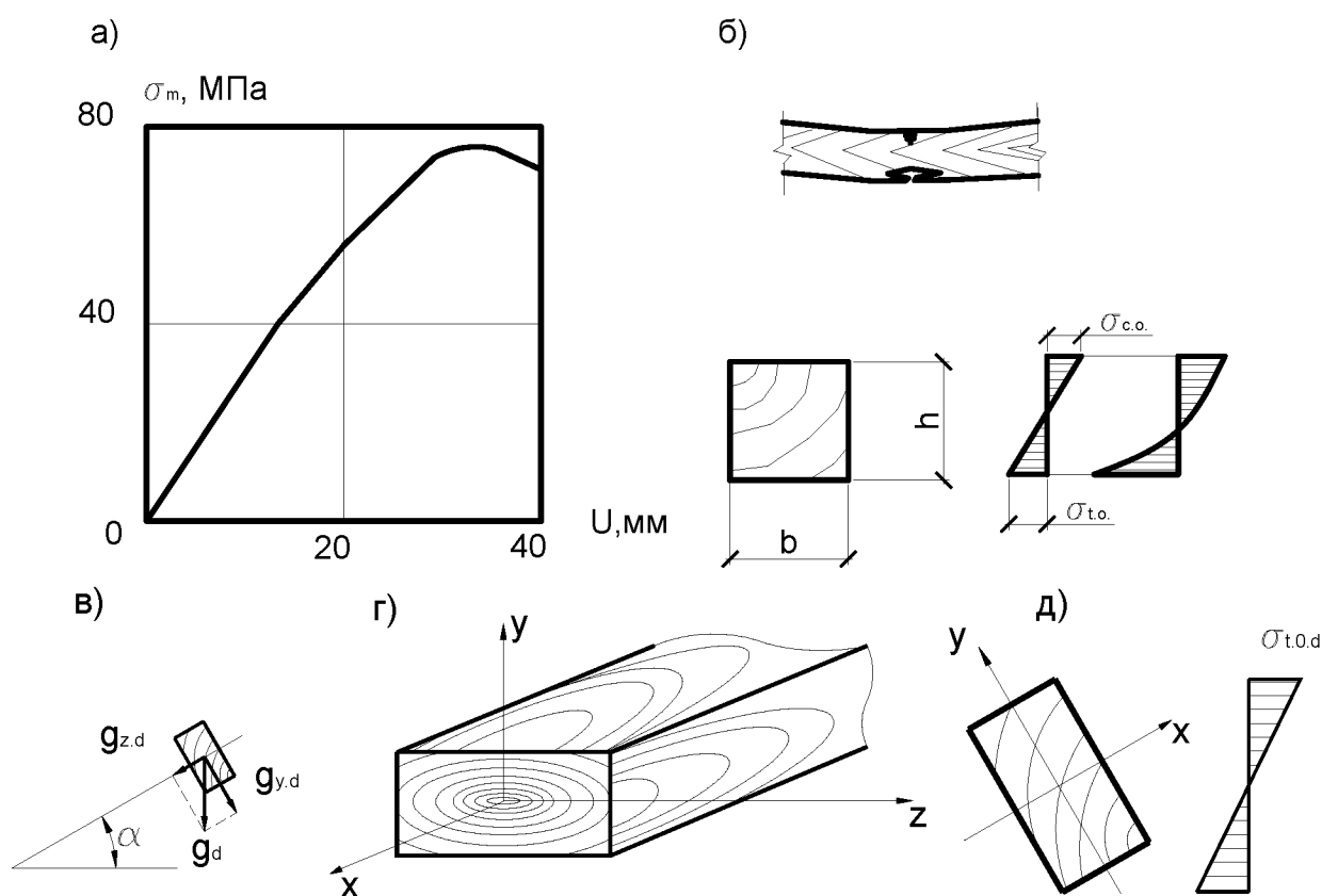
Рис. 5.4. Изгибаемый элемент:
