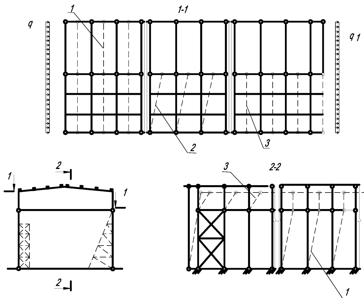
Рис. 9.7. Кинематическая схема каркаса здания без связей с защемленными колоннами
