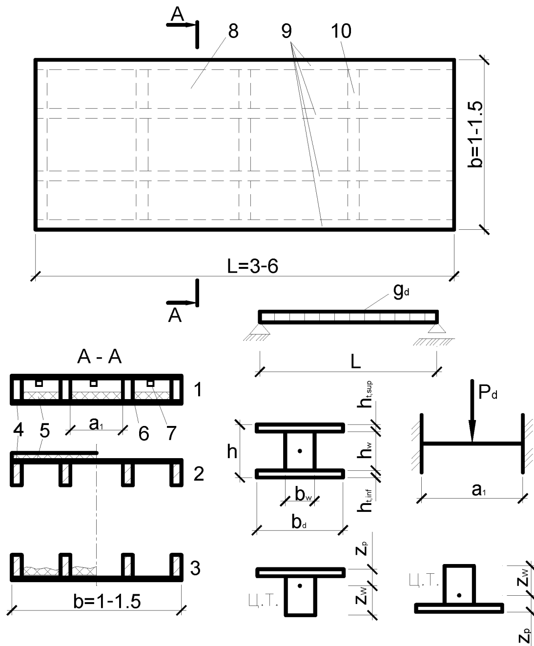
Рис. 8.8. Клеефанерные плиты или панели настила: конструкция и расчетные схемы;
