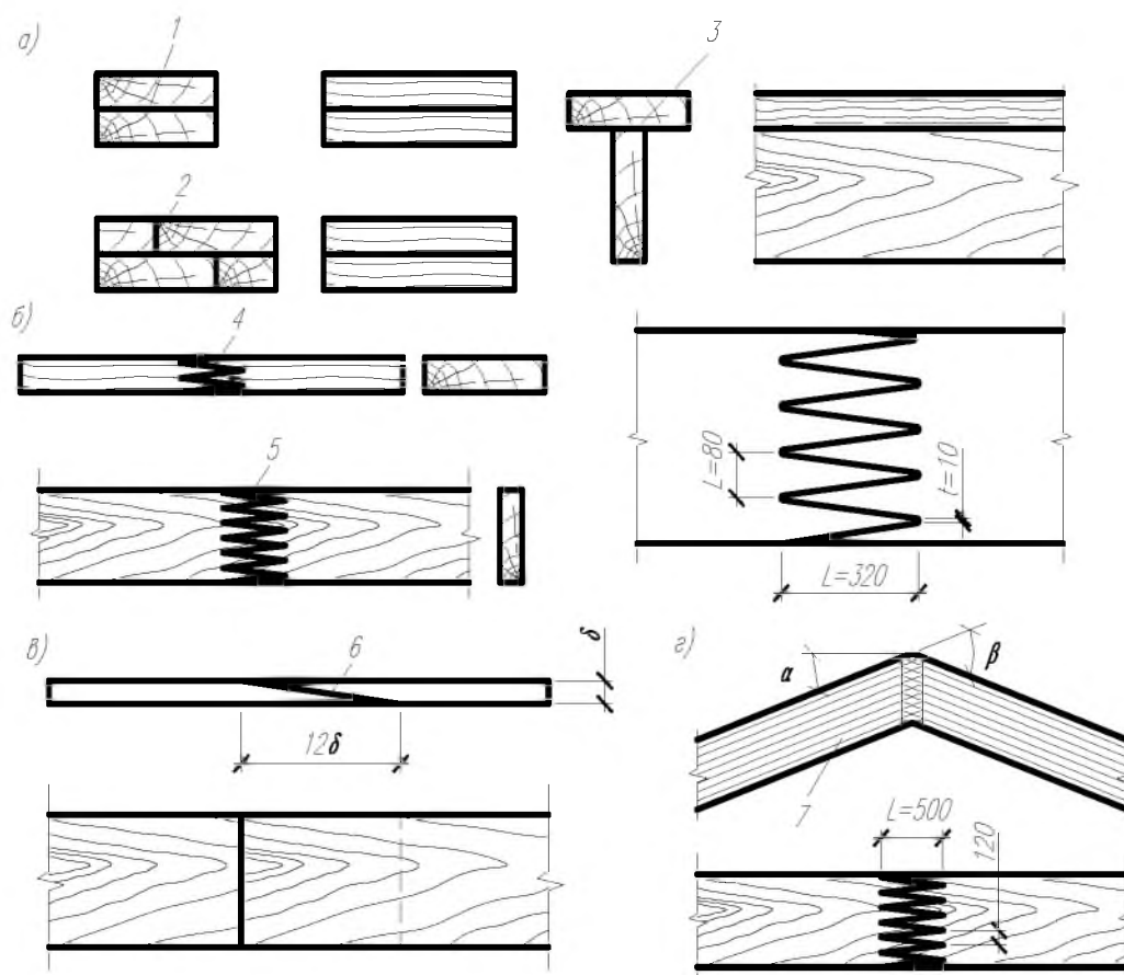
Рис. 6.3. Клеевые стыки:
