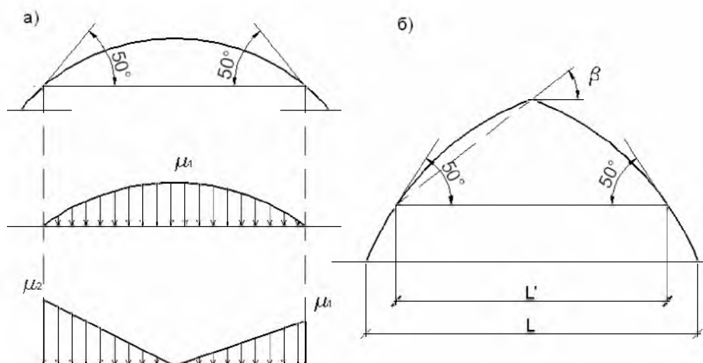
Рис. 4.1. Определение снеговой нагрузки
