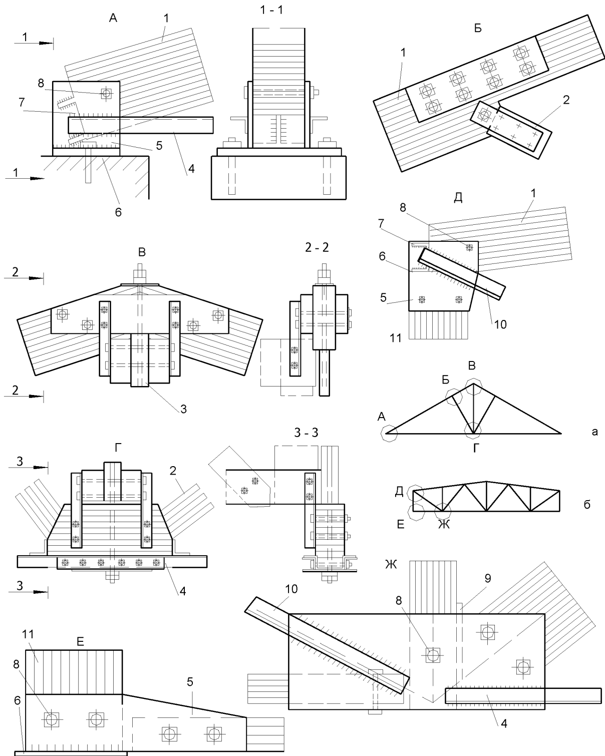
Рис. 12.4. Треугольная и пятиугольная металлодеревянные клееные фермы: а – общий вид треугольной фермы; б – то же, пятиугольной; 1 – верхний пояс; 2 – кар- кас; 3 – стойка; 4 – нижний пояс; 5 – траверса; 6 – опорная плита; 7 – опорная швеллер- ная шайба; 8 – болт; 9 – металлическая диафрагма; 10 – опорный каркас; 11 – опорная стойка
