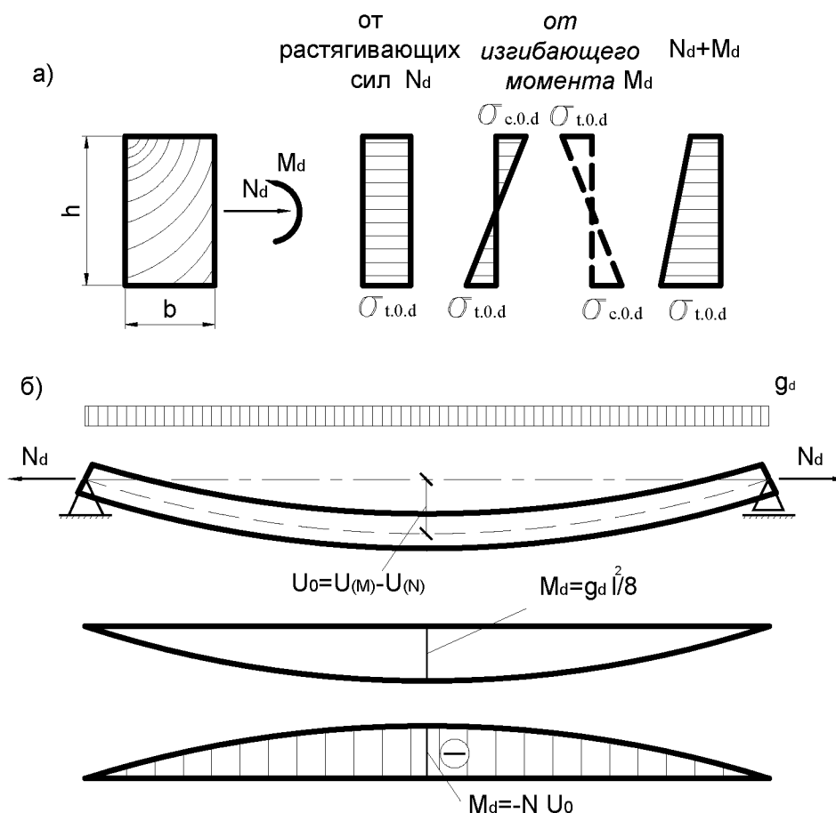
Рис. 5.5. Растянуто-изгибаемый элемент: а – эпюры нормальных напряжений; б – схема работы и эпюры изгибающих моментов
