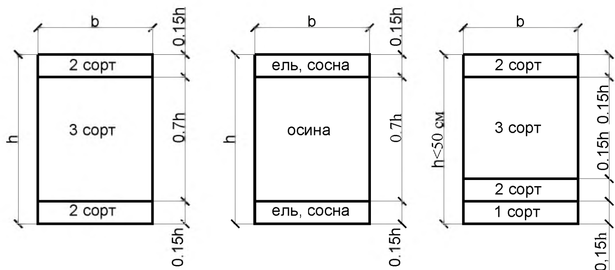
Рис. 11.4. Варианты компоновки поперечного сечения доштокклееных балок
