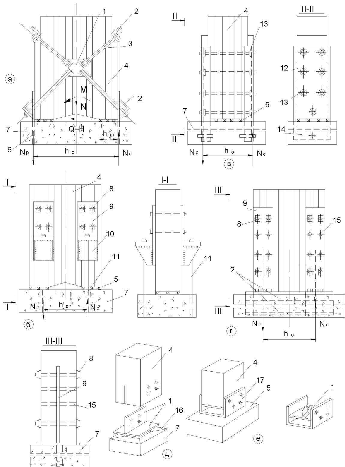
Рис. 11.11. Опорные узлы жестко защемленных (а – г) и шарнирно опирающихся сжатых стоек (д, е): 1 – фанка; 2 – уголок; 3 – тяж; 4 – стойка; 5 – изоляция; 6 – анкер из полосовой стали; 7 – фундамент; 8 – болт; 9 – планка; 10 – сварной столик; 11 – анкер из круглой стали; 12 – швеллер; 13 – зубчатая шпонка; 14 – штырь; 15 – нагель; 16 – квадратная труба; 17 – гнутая фанка
