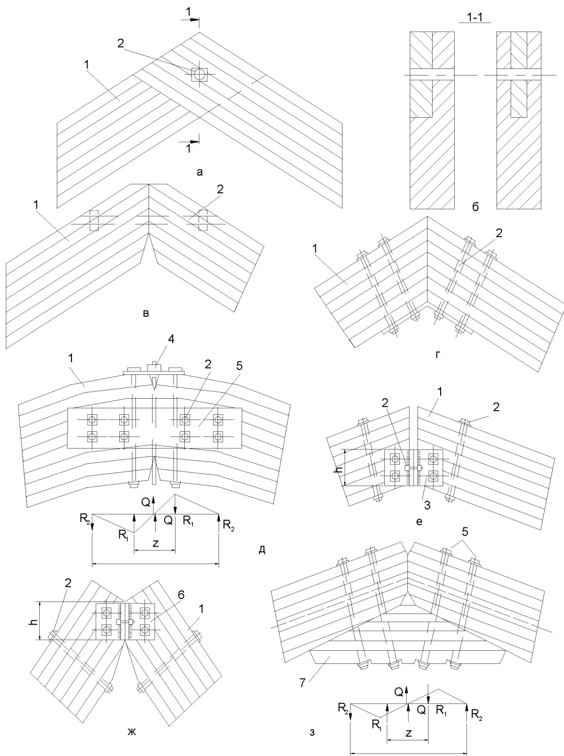
Рис. 10.4. Коньковые узлы арок и рам малых и средних пролетов:
