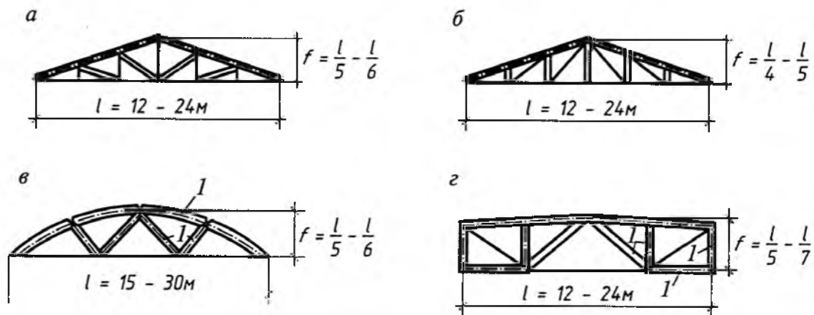
Рис. 12.1. Клеефанерные фермы:
