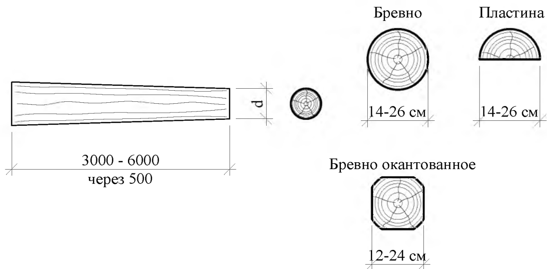
Рис. 2.1. Бревна
