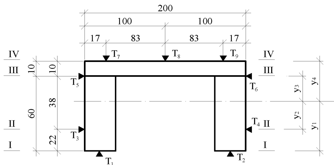
Рис. 3.3. Схема расстановки тензорезисторов
