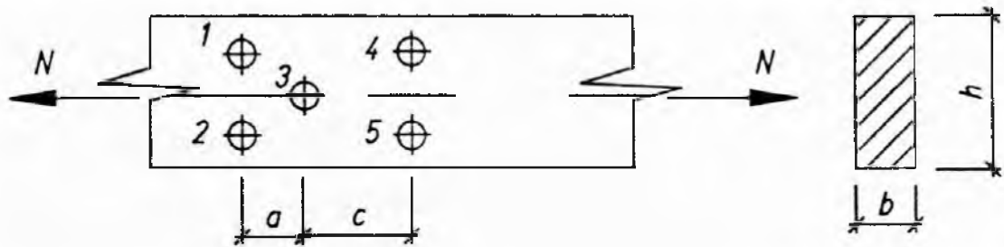
Рис. 3.1. Растянутый элемент
