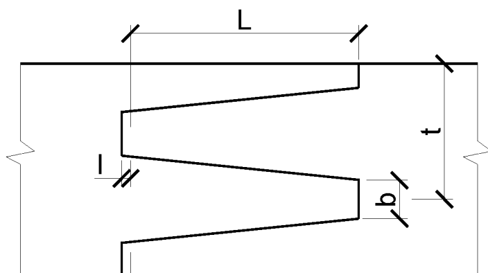
Рис 14.1. Схема зубчатых шипов после фрезерования: L – длина шипа; t – шаг шипа; b – затупление; l – зазор
