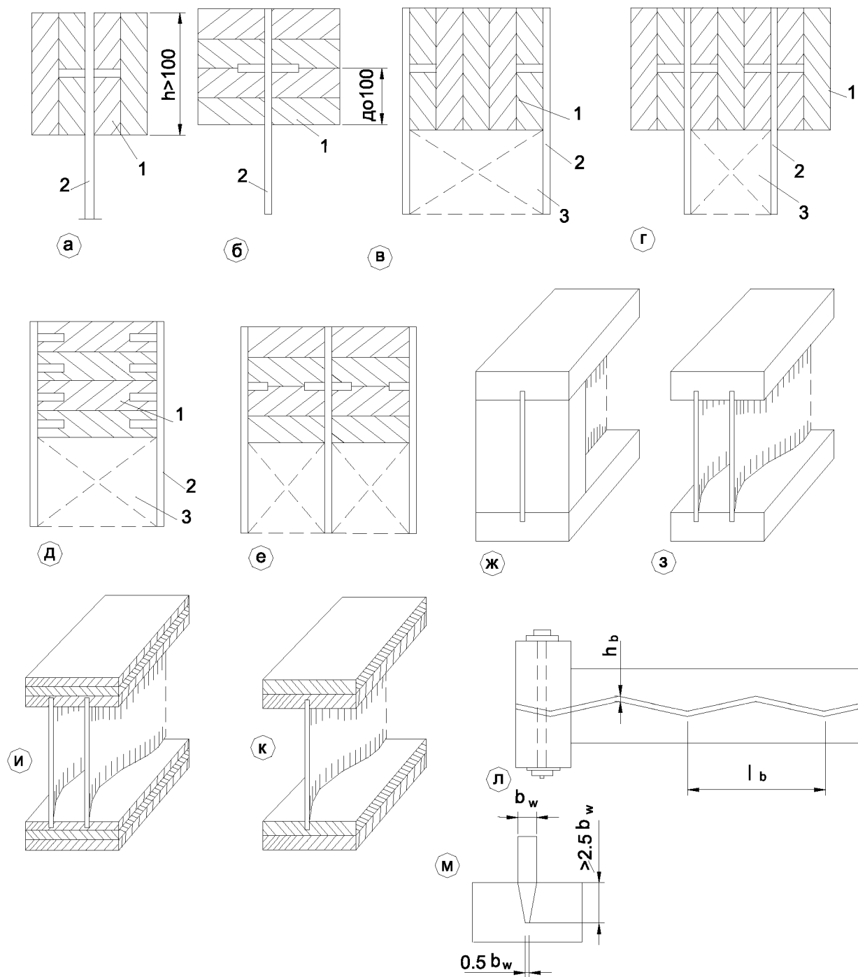
Рис. 11.6. Клеифанерные балки с плоской и волнистой стенкой:
