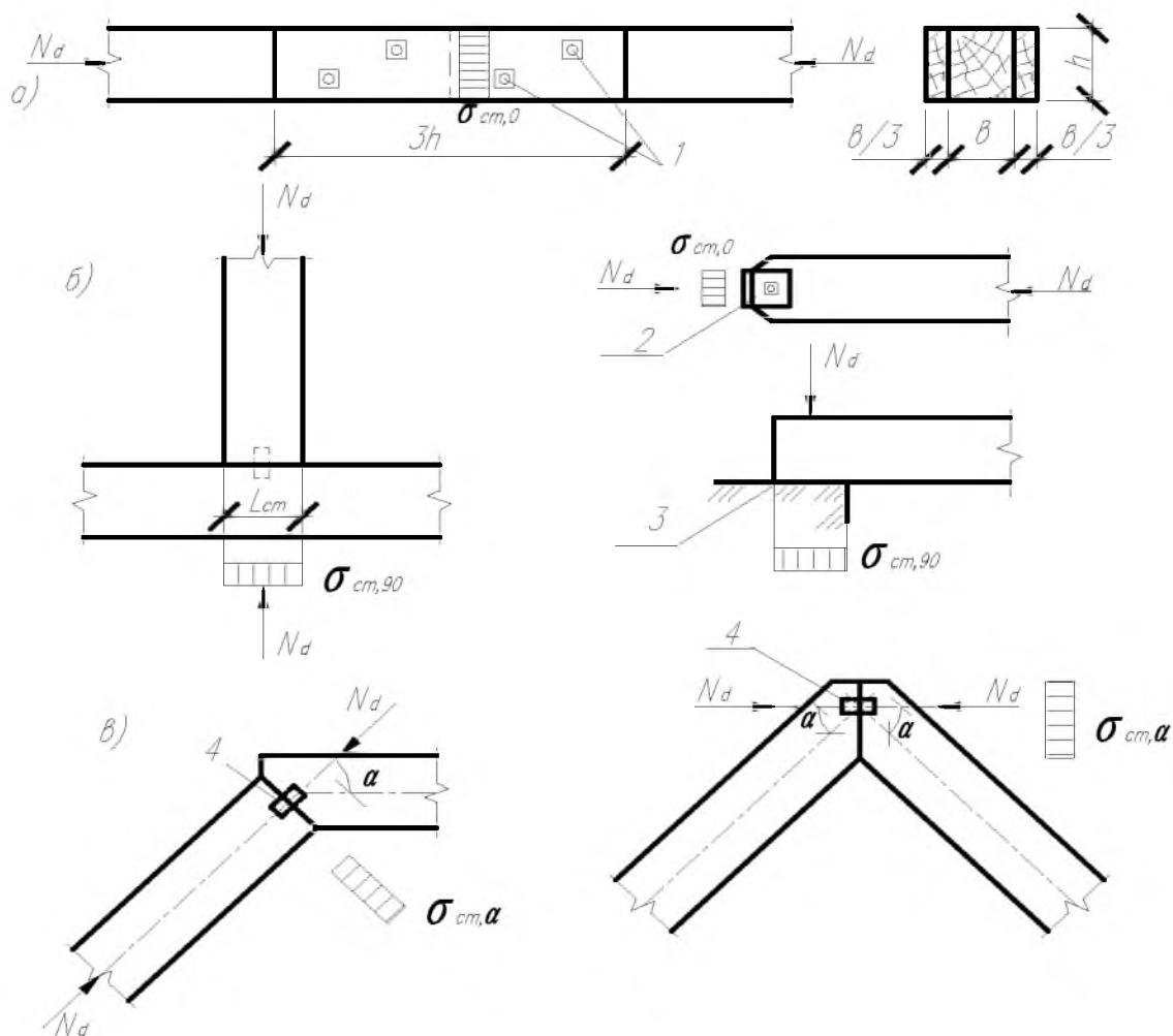
Рис. 6.2. Лобовые упоры: а – продольные; б – поперечные; в – наклонные; 1 – стяжной болт; 2 – стальное крепление; 3 – опора; 4 – штырь
