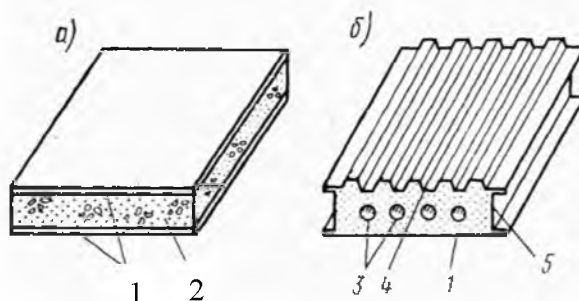
Рис. 8.10. Основные типы трехслойных панелей:
