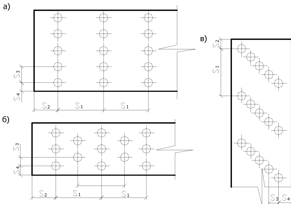
Рис. 4.2. Схемы расстановки нагелей:
