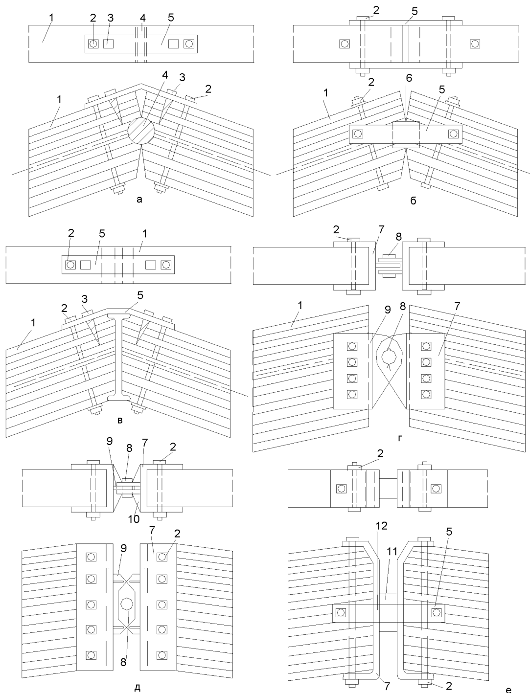
Рис. 10.3. Коньковые узлы рам средних и больших пролетов:
