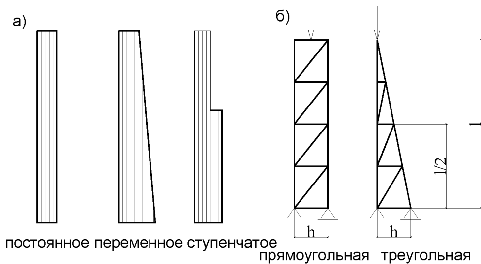
Рис. 11.9. Виды стоек:
