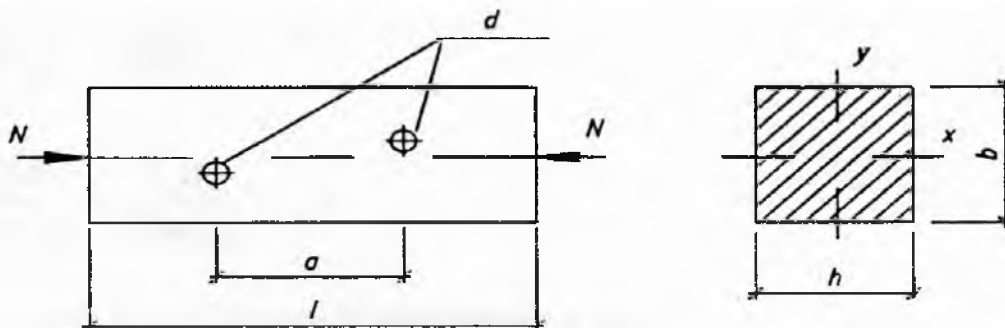
Рис. 3.2. Центрально-сжатый стержень
