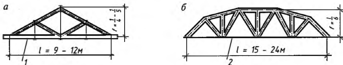
Рис. 12.2. Брусчатые фермы:
