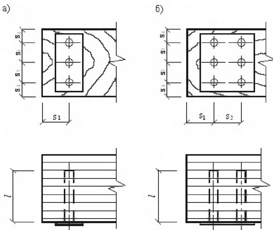
Рис. 7.3. Схема расстановки вклеенных поперек волокон древесины стержней: а – однорядная расстановка; б – двухрядная расстановка
