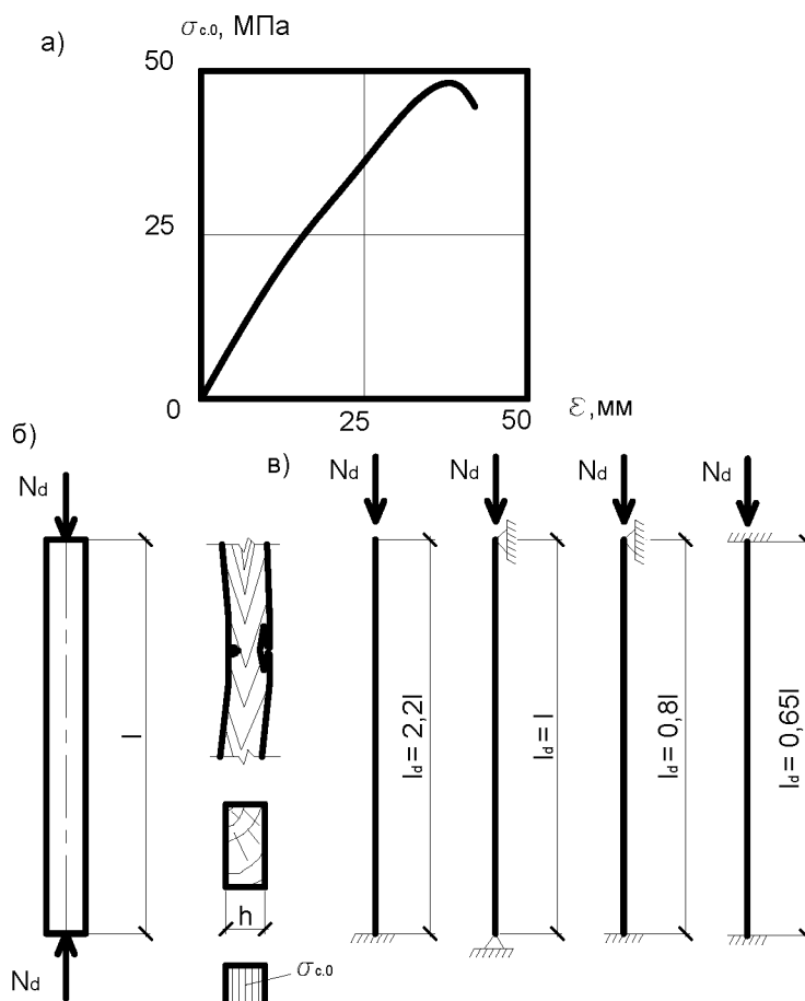
Рис. 5.2. Сжатый элемент:
