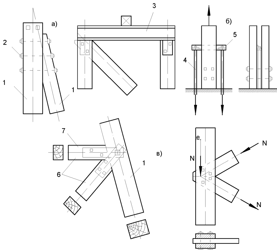
Рис. 11.10. Узлы решетчатых стоек:
