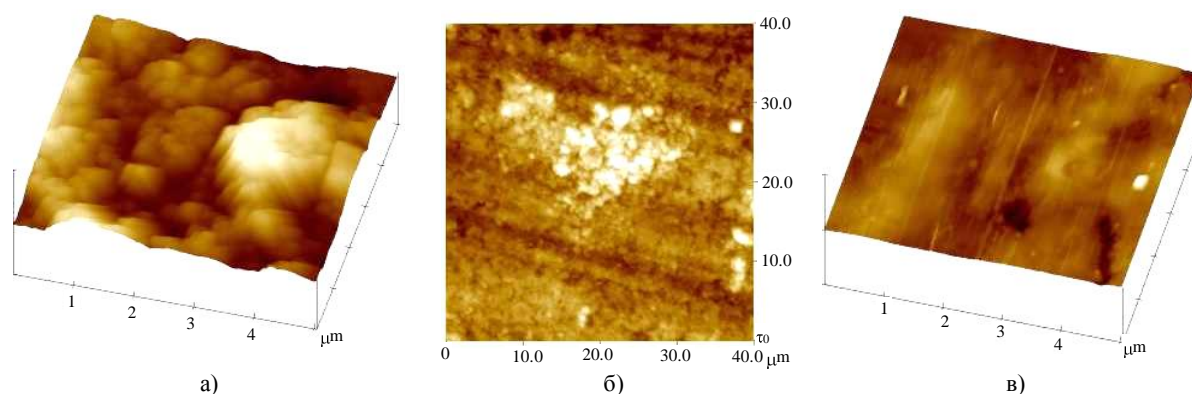
Рис. 3. Морфология поверхности твердого сплава ВК6, подвергнутого ТГХО, до (а, б) и после испытаний на трение (в) режим ТГХО: ХО в оптимальном составе TiO_2-MoO_3 при T = 100 °С, \tau = 15 мин; ТО при T = 1000 °С, \tau = 10 мин
