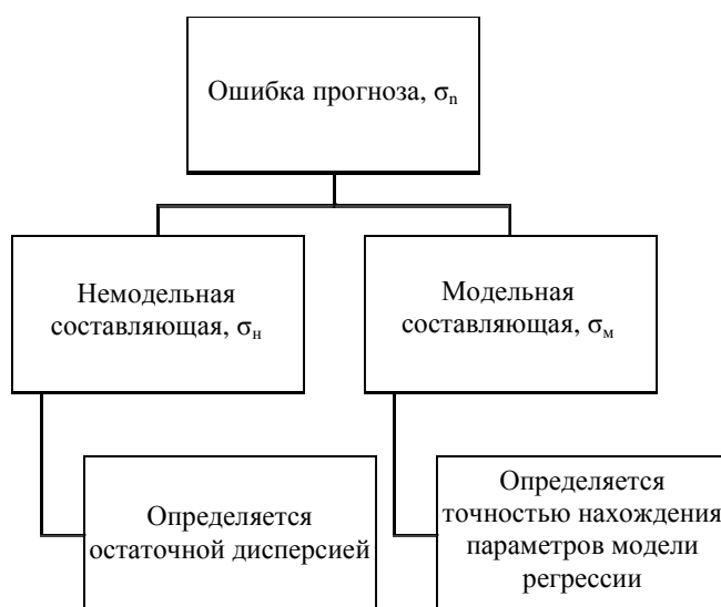
Рисунок 1. – Схема представления ошибки прогноза \sigma_n значения ВВП по паритету покупательной способности в момент времени t_n в агрегированном виде
