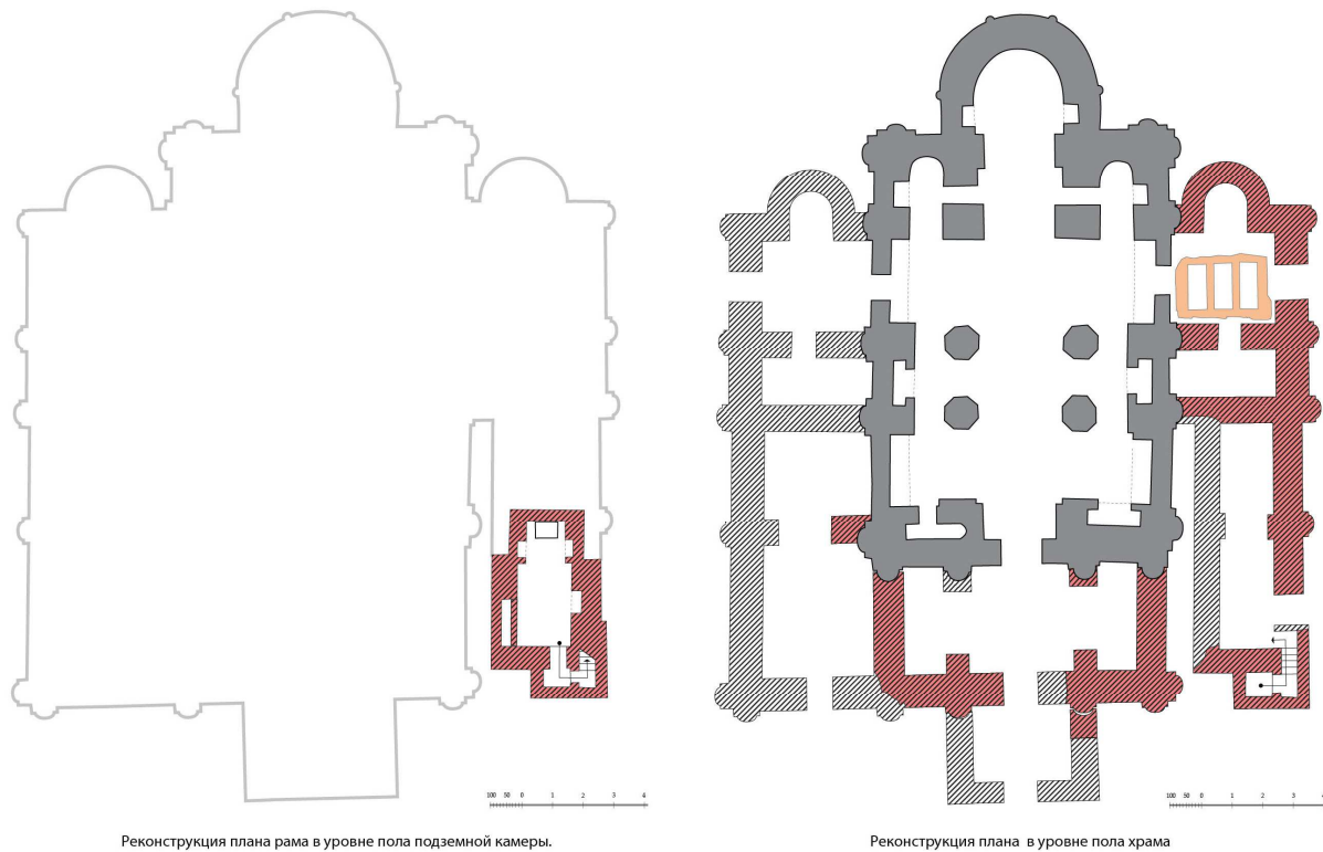
Рисунок. – Реконструкция плана Спасо-Преображенского храма Спасо-Ефросиньевского монастыря в г. Полоцке на основании данных археолого-архитектурных исследований 2015-2018 гг. (реконструкция Е.Н. Торшина и П.Л. Зыкова)
