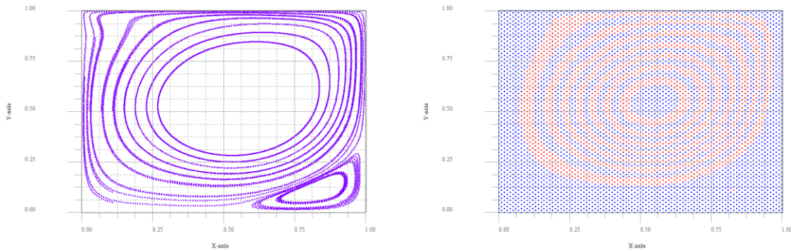
Рис.4. Поле линий тока и функции тока для Re=1000 для профиля скорости "равнобедренный треугольник" с соотношением кусочно-линейных областей как 5:0:5.
