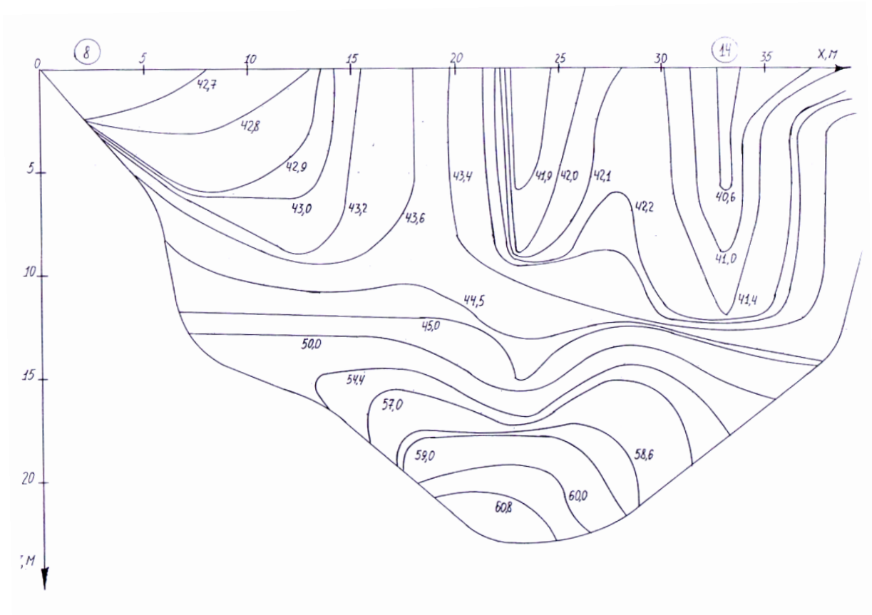
Рис.1 Разрез температурного поля геотермального озера
