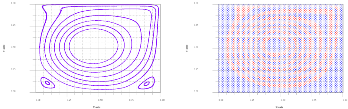
Рис.3. Поле линий тока и функции тока для Re=1000 для профиля скорости "равнобедренная трапеция" с соотношением кусочно-линейных областей как 1:8:1.
