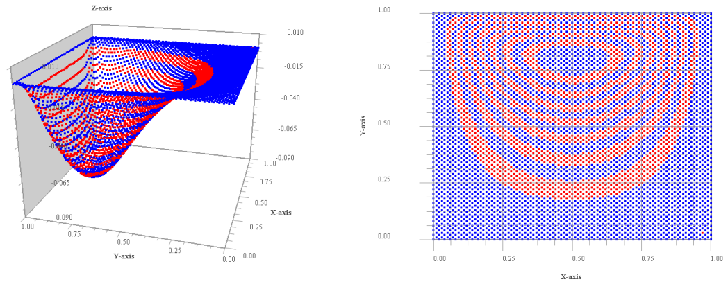
Рис.2. Поле функции тока с параметром Рейнольдса Re=1 .
