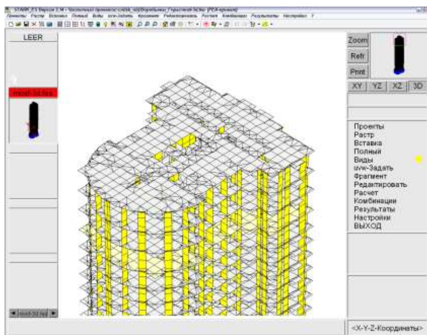
Рис. 5. Пример проекта высотного здания в StarkES (г. Москва, жилой комплекс Воробьевы горы), число этажей: всего – 52, в том числе подземных – 5; 88 377 элементов; 71 169 узлов; 427 014 неизвестных
