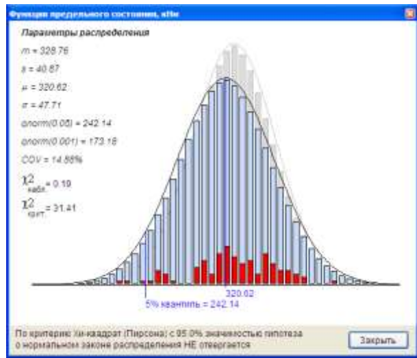
Рис. 3. Результат статистического моделирования балки из рассматриваемого примера с большим (10 %) разбросом прочностных характеристик материалов
