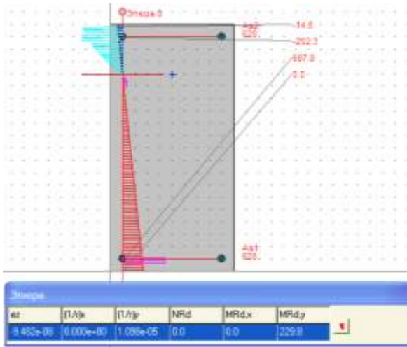
Рис. 2. Результат расчета балки при проектировании
