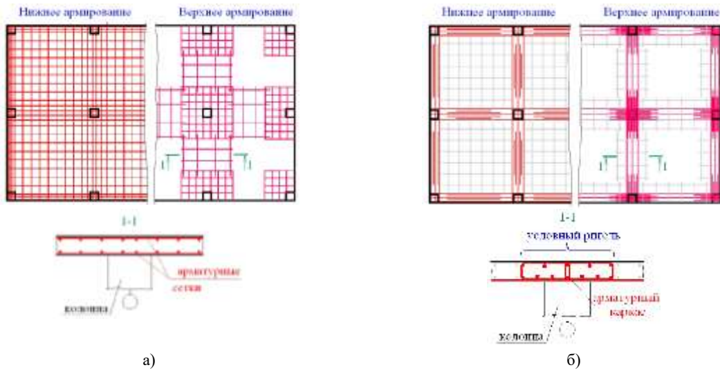
Рис. 6. Традиционная схема армирования плоских монолитных плит перекрытия (а); концентрированное «ригельное» армирование плоских плит пространственными каркасами (б)
