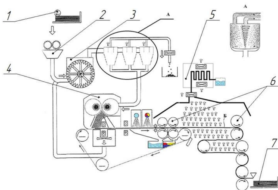
Рисунок 1. – Схема персональной станция переработки офисной макулатуры где: А – блок очистки волокна от загрязнений; 1 – блок приема бумаги; 2 – блок разрезания и измельчения бумаги; 3 – блок механического разрыва бумажной массы; 4 – блок формования; 5 – блок сушки и опреснения влаги; 6 – блок каландрирования; 7 – блок резки и вывода бумажного листа.
