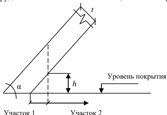
Рис. 3. Расчёт площади помещений мансардного этажа: участок № 1 – нежилая площадь (не включается в расчёт площади помещения); участок № 2 – жилая площадь (включается в расчёт площади помещения); t – толщина ограждения; \alpha – угол наклона кровли к горизонту; h – высота до наклонного потолка
