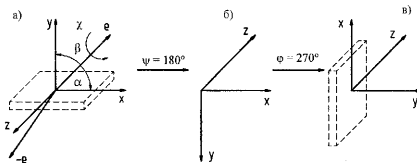
Рис. 2. Последовательность поворотов координатного триэдра и вектор конечного поворота
