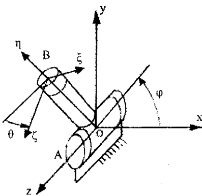
Рис. 4. Схема механизма ориентации реализующего повороты вокруг двух подвижных осей
