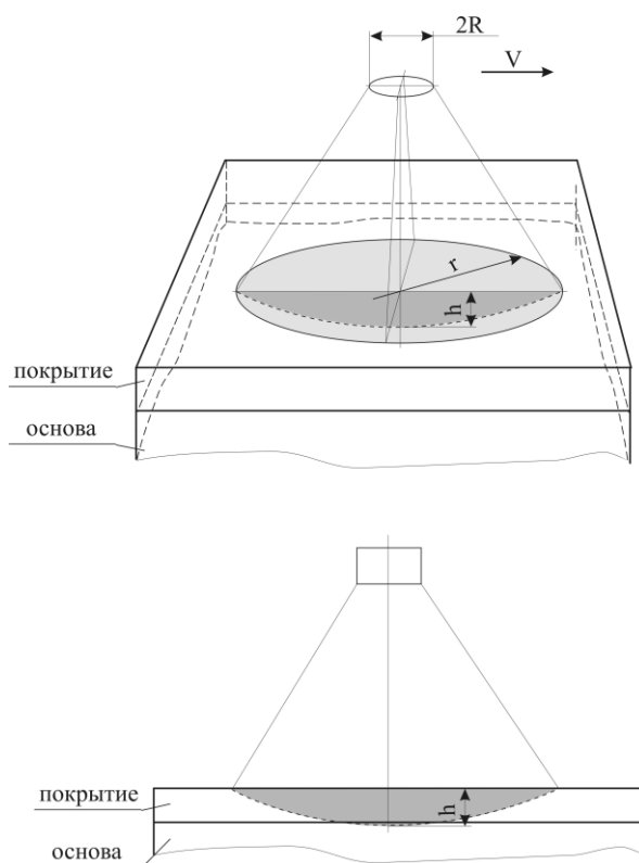
Рис. 1. Схема оплавления:
