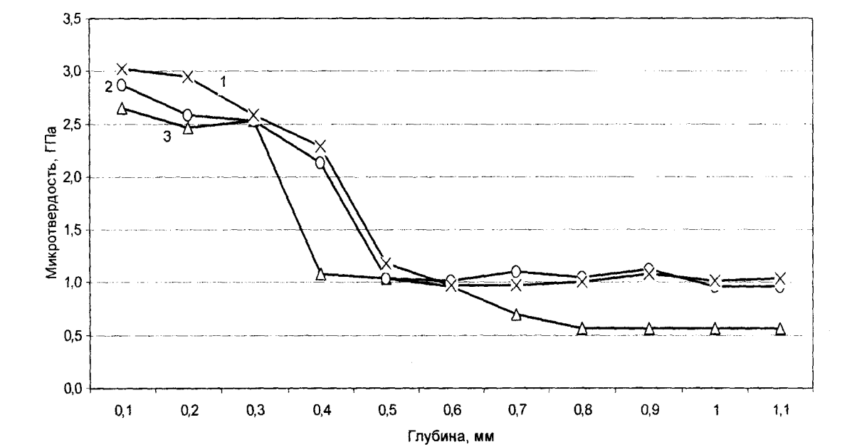
Рис. 2. Изменение микротвердости по глубине упрочненного образца с последующей термообработкой: 1 - закалка ТВЧ и отпуск; 2 - объемная закалка и отпуск; 3 - без термообработки (эталон)
