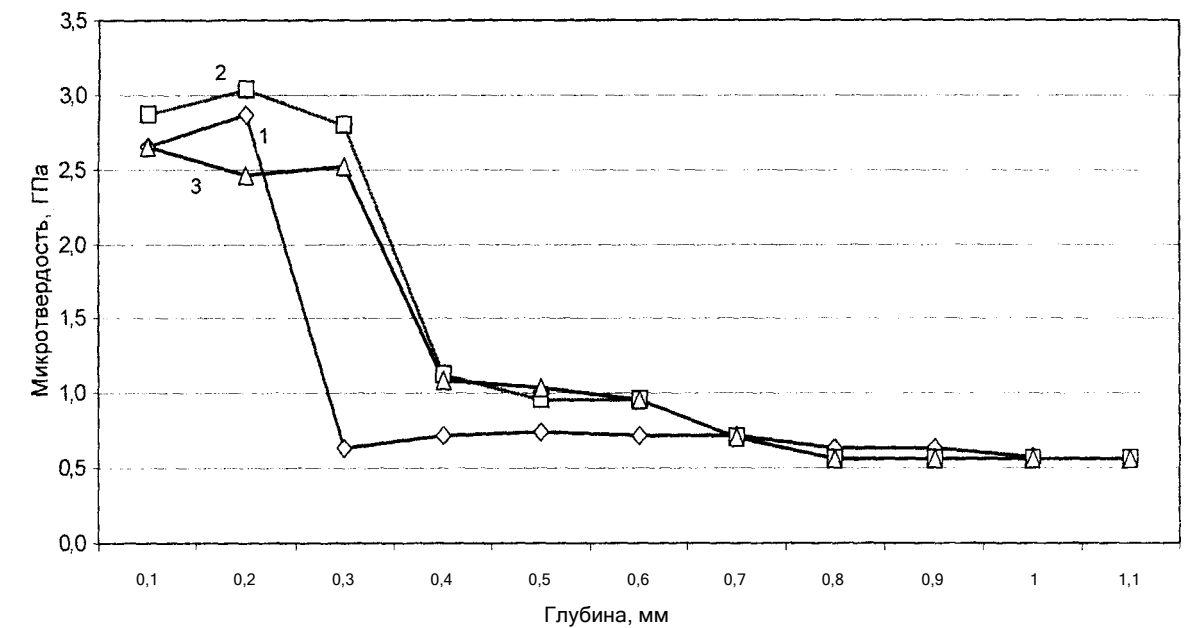
Рис. 1. Изменение микротвердости по глубине упрочненного образца: 1 - закаленная подложка; 2 - закаленная подложка с последующим отпуском; 3 - без термообработки
