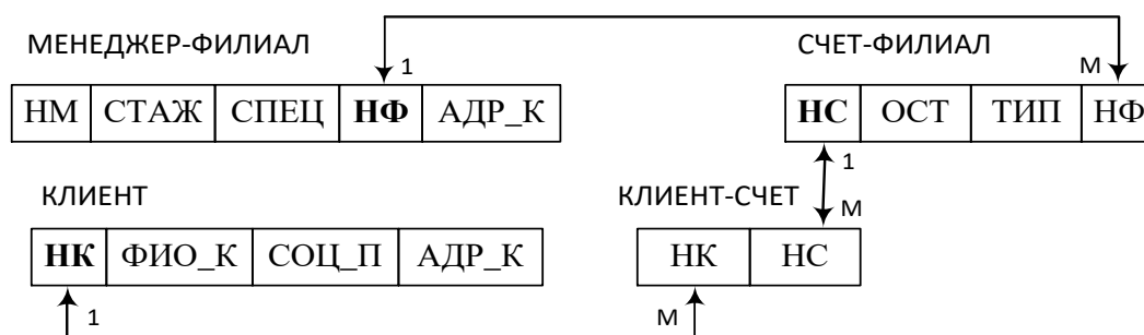
Рисунок 3.7. – Реляционная модель предметной области БАНК
