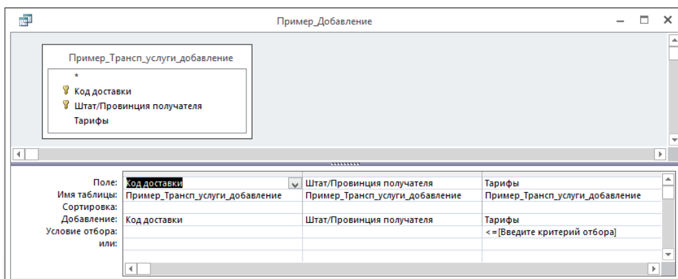
Рисунок 6.42. – Создание запроса на добавление данных в таблицу
