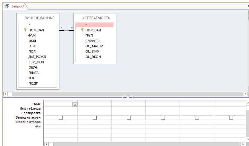
Рисунок 3.2. – Окно конструктора запроса
