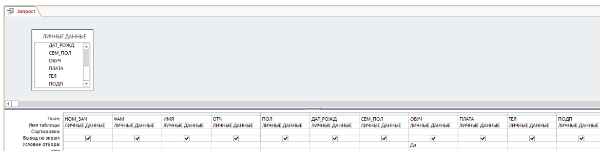
Рисунок 3.35. – Окно конструктора запроса на создание таблицы ПЛАТНИКИ
