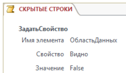
Рисунок 6.28. – Текст макроса СКРЫТЫЕ СТРОКИ
