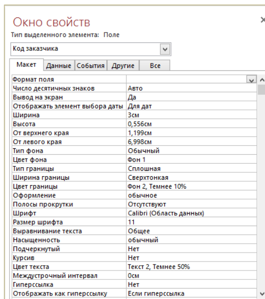
Рисунок 6.81. – Окно свойств поля «Код заказчика»
