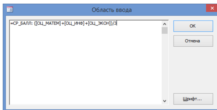
Рисунок 3.14. – Окно «Область ввода»
