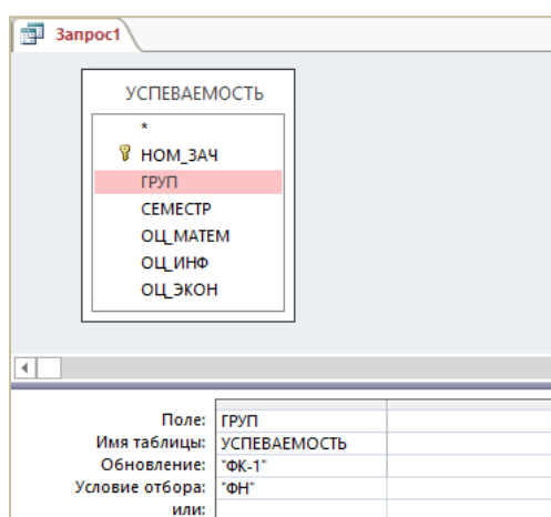
Рисунок 3.32. – Окно конструктора запроса на обновление
