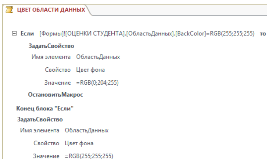
Рисунок 6.24. – Текст макроса ЦВЕТ ОБЛАСТИ ДАННЫХ
