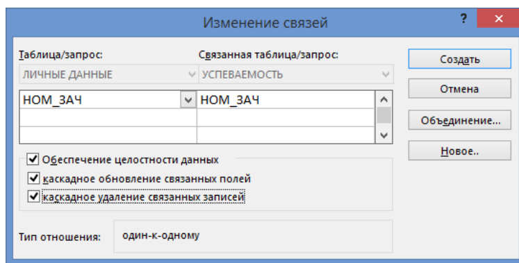
Рисунок 2.20. – Окно «Изменение связей»
