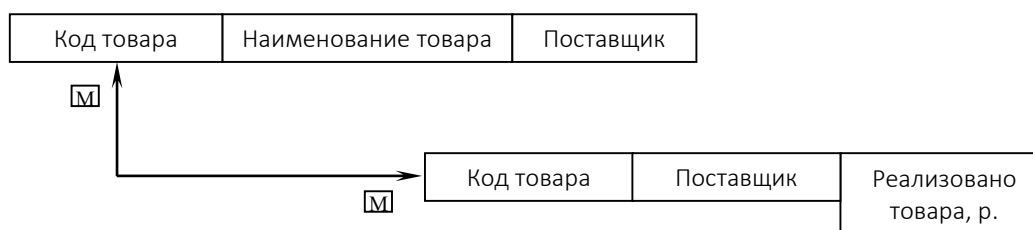
Рисунок 2.10. – Пример связи M:M
