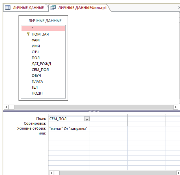
Рисунок 2.48. – Окно расширенного фильтра
