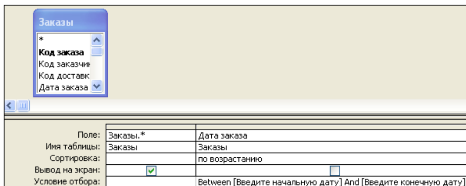
Рисунок 6.32. – Создание запроса с параметрами
