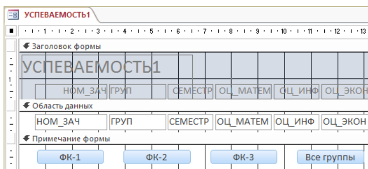
Рисунок 6.22. – Внешний вид формы УСПЕВАЕМОСТЬ1 в режиме конструктора
