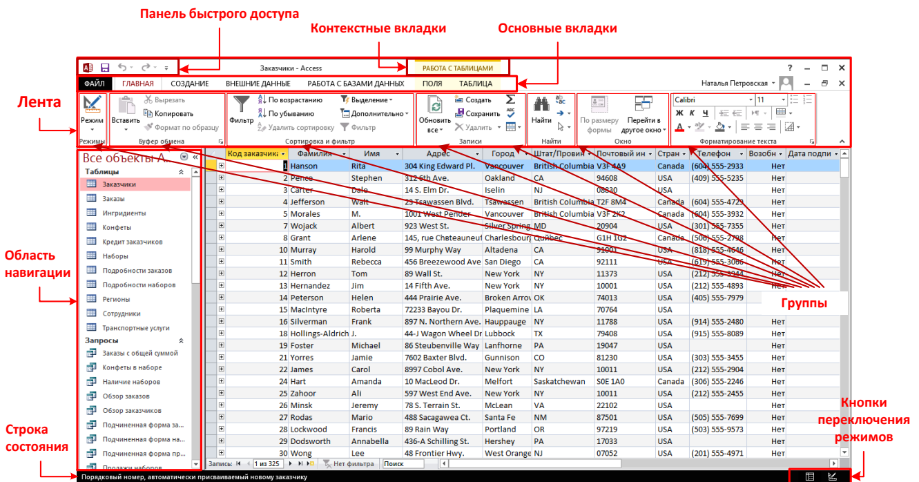
Рисунок 6.4. – Окно Microsoft Access 2013
