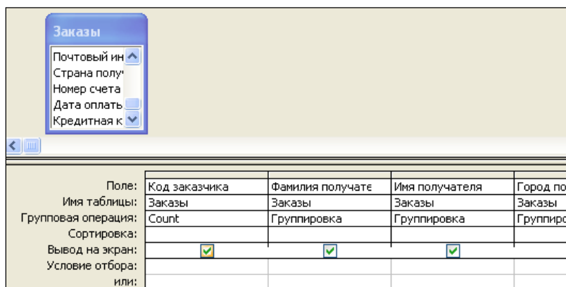
Рисунок 6.31. – Использование в запросе группировки и статистической функции
