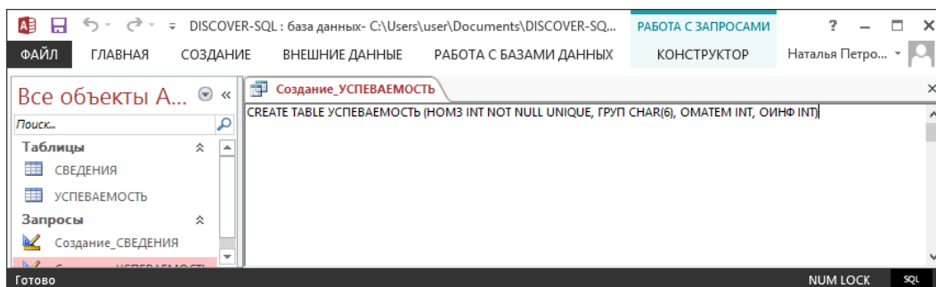
Рисунок 7.6. – SQL-запрос на создание таблицы УСПЕВАЕМОСТЬ
