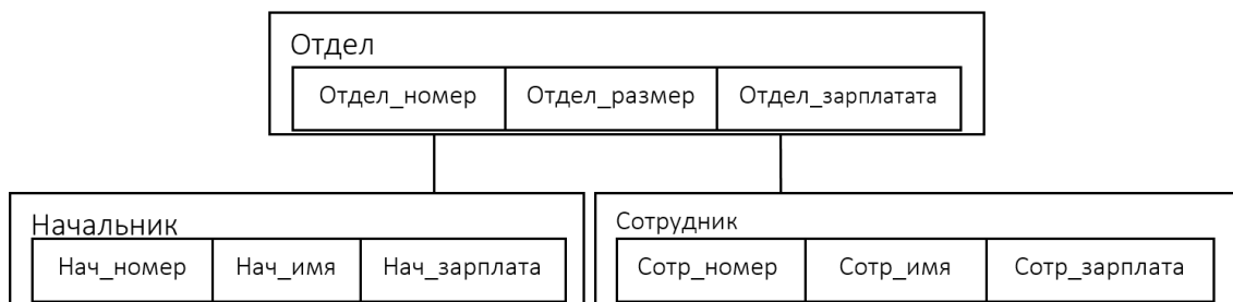
Рисунок 2.2. – Пример логической структуры иерархической БД
