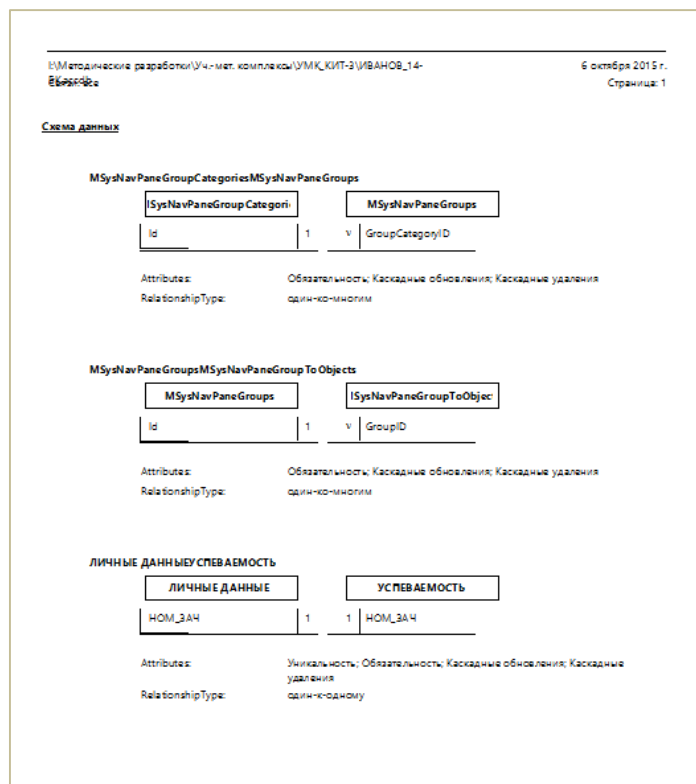
Рисунок 8.3. – Окно «Описание объектов» с информацией о связях в базе данных ФАМИЛИЯ_Группа
