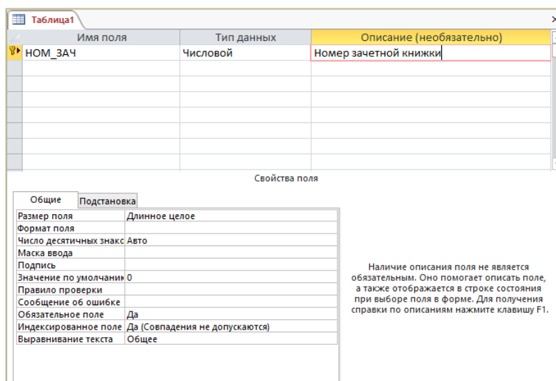
Рисунок 2.7. – Свойства поля НОМ_ЗАЧ
