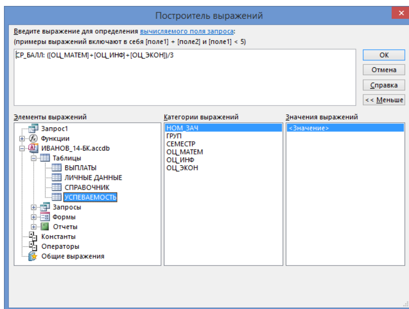
Рисунок 3.13. – Окно построителя выражений
