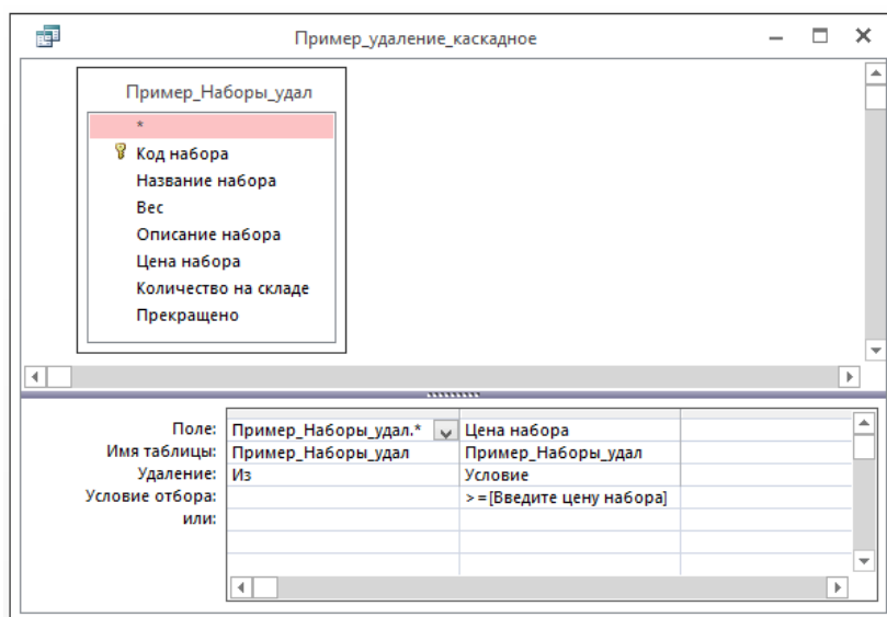
Рисунок 6.46. – Создание запроса на удаление данных из таблиц, связанных отношением 1:∞ с обеспечением целостности данных и выполнением каскадных операций
