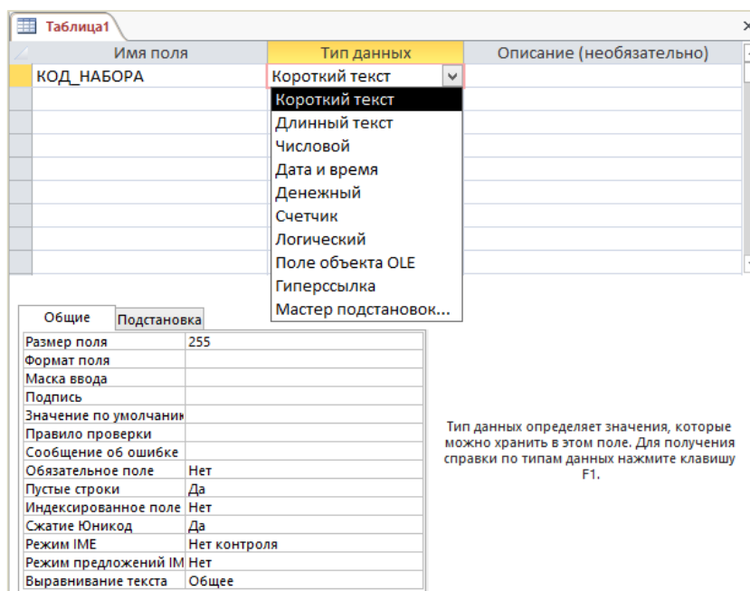
Рисунок 6.15. – Окно определения структуры таблицы в режиме конструктора
