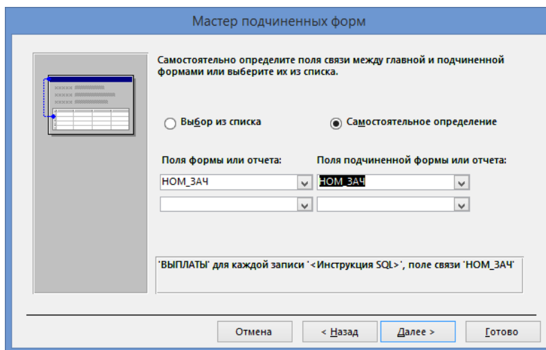
Рисунок 4.50. – 3-е окно мастера подчиненных форм
