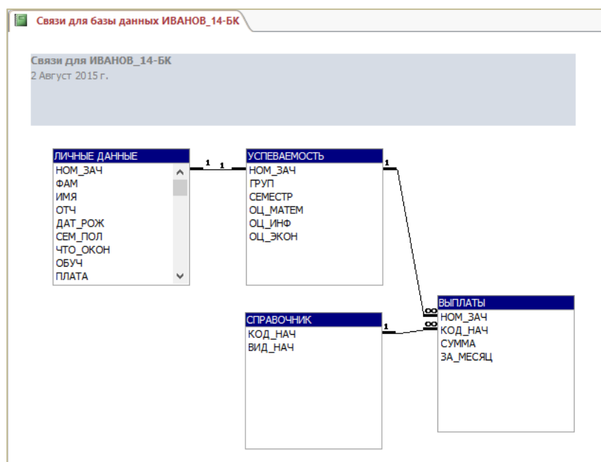
Рисунок 2.26. – Отчет об установленных в БД межтабличных связях
