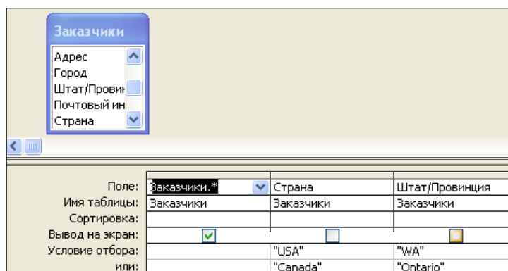
Рисунок 6.27. – Запрос выбора с использованием логических операторов And и Or
