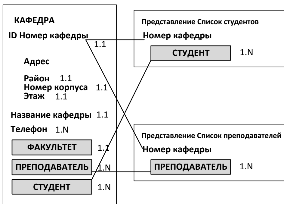
Рисунок 3.14. – Представления семантического объекта КАФЕДРА : Список студентов и Список преподавателей
