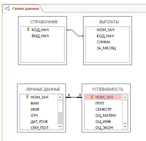
Рисунок 2.21. – Окно «Схема данных» с установленной связью между таблицами ЛИЧНЫЕ ДАННЫЕ и УСПЕВАЕМОСТЬ
