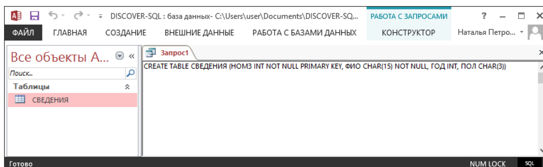
Рисунок 7.3. – SQL-запрос на создание таблицы СВЕДЕНИЯ
