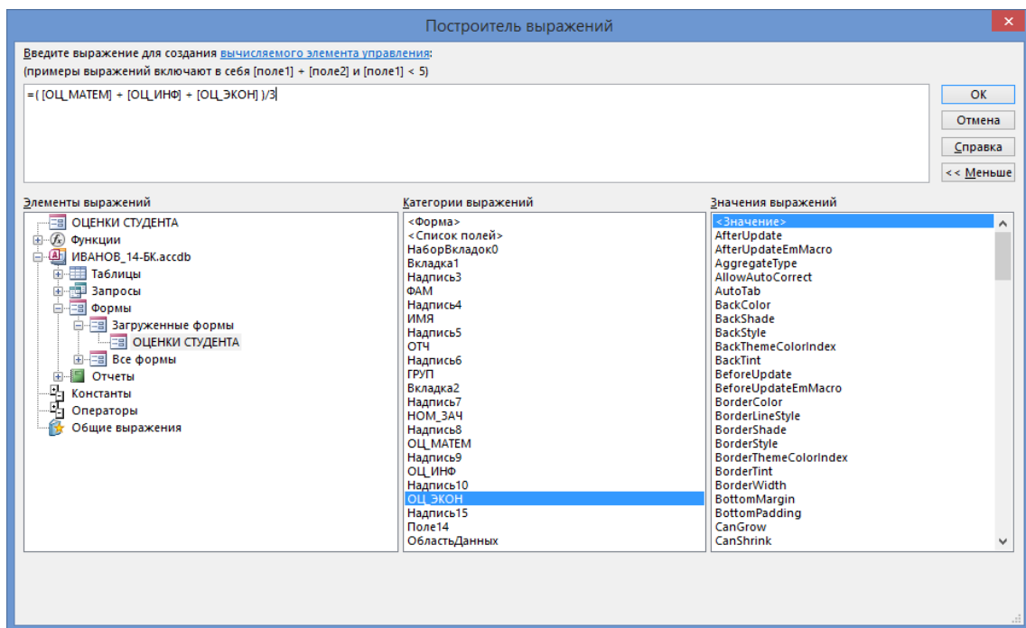
Рисунок 4.36. – Создание вычисляемого поля для формы в построителе выражений
