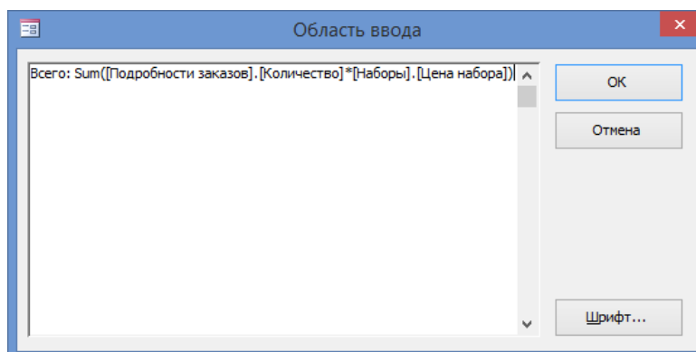
Рисунок 6.29. – Область ввода
