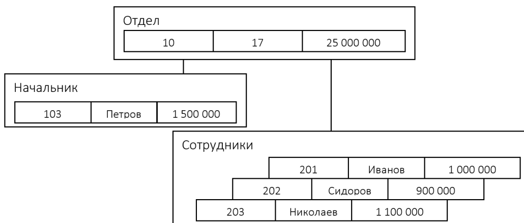
Рисунок 2.3. – Данные в иерархической базе
