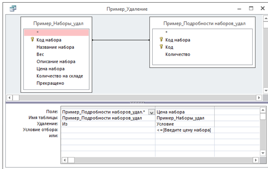
Рисунок 6.45. – Создание запроса на удаление данных из таблиц, связанных отношением 1:∞ с обеспечением целостности данных, но без выполнения каскадных операций
