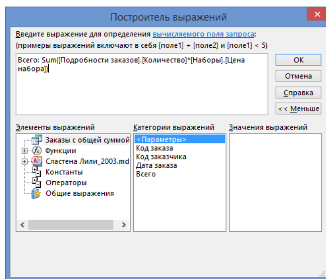
Рисунок 6.6. – Окно «Построитель выражений» при формировании вычисляемого поля запроса
