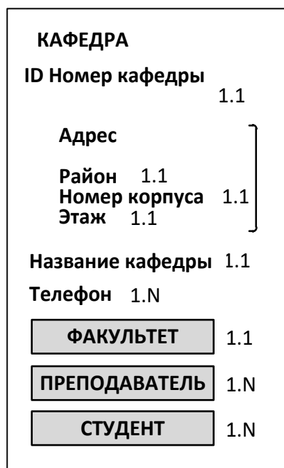
Рисунок 3.13. – Семантическая объектная диаграмма объекта КАФЕДРА
