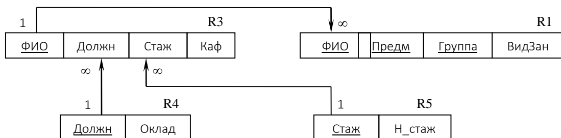
Рисунок 3.12. – Схема данных БД «Преподаватель», полученная в процессе нормализации отношений
