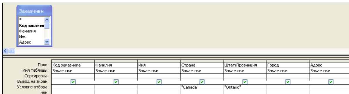
Рисунок 6.25. – Запрос выбора с использованием логического оператора And
