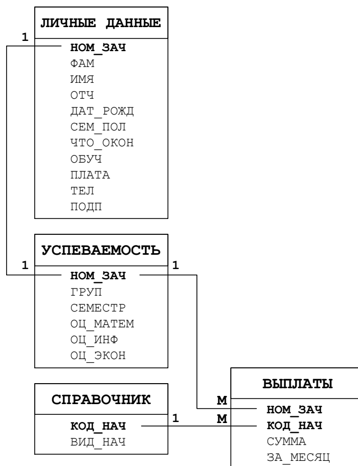
Рисунок 1.2. – Логическая модель базы данных
