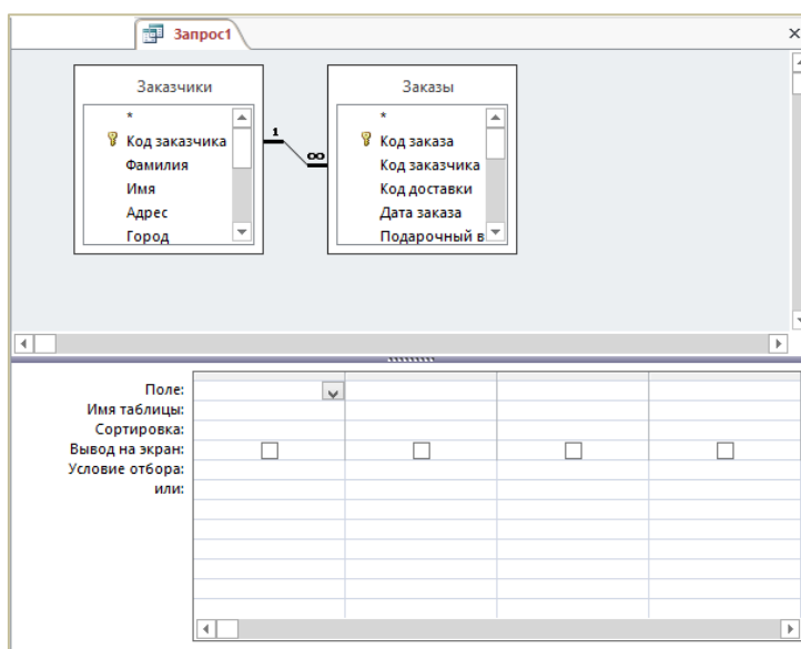
Рисунок 6.24. – Окно «Конструктор запросов»
