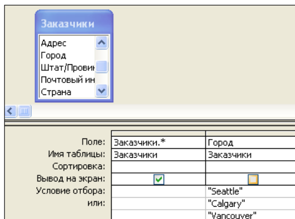
Рисунок 6.26. – Запрос выбора с использованием логического оператора Or
