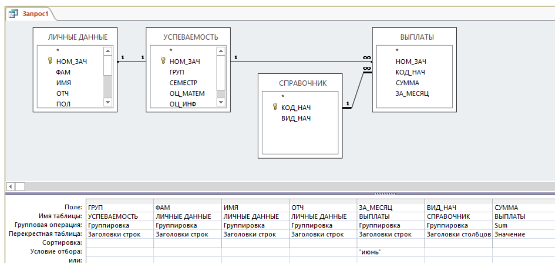
Рисунок 3.29. – Окно конструктора перекрестного запроса
