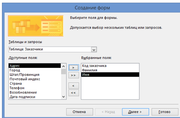
Рисунок 6.57. – Стартовое окно мастера форм
