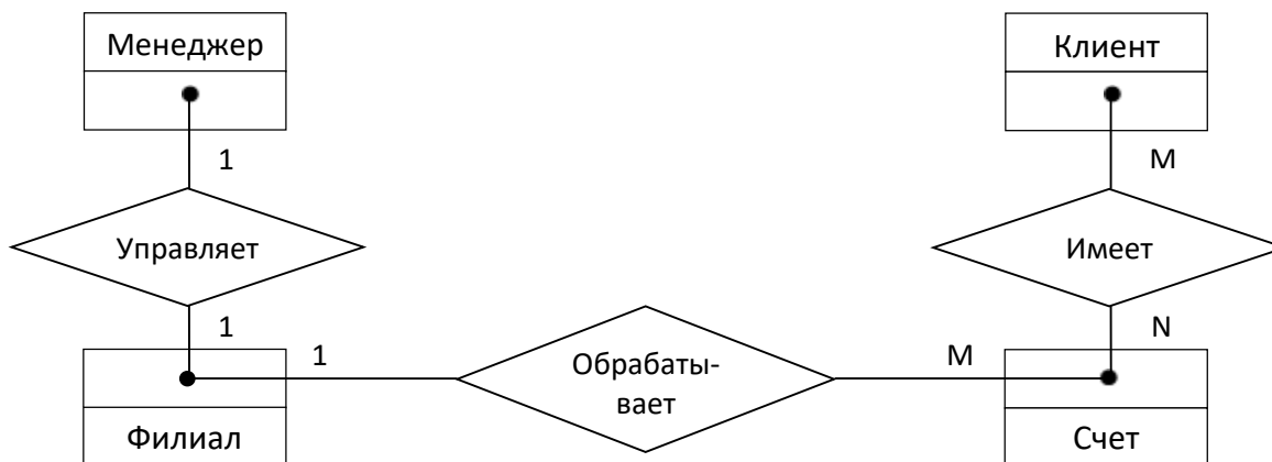
Рисунок 3.5. – Пример ER-модели предметной области БАНК
