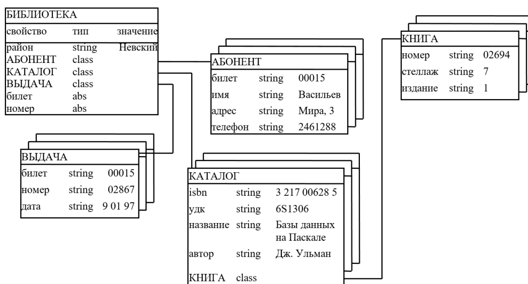
Рисунок 2.12. – Логическая структура БД библиотечного дела
