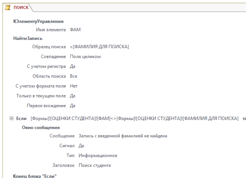
Рисунок 6.18. – Текст макроса ПОИСК
