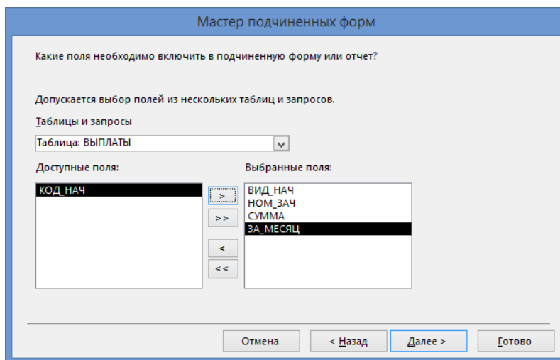
Рисунок 4.49. – 2-е окно мастера подчиненных форм
