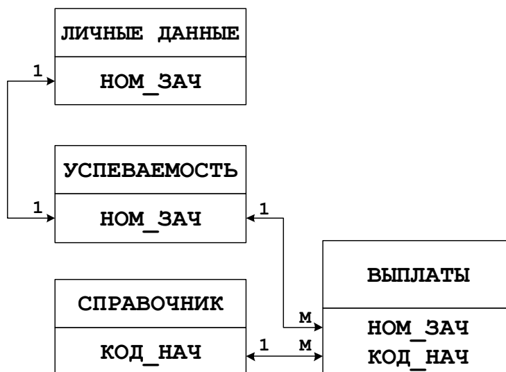
Рисунок 1.1. – Информационно-логическая модель предметной области ДЕКАНАТ-БУХГАЛТЕРИЯ
