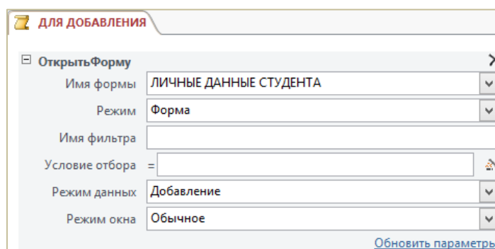
Рисунок 6.3. – Макрос ДЛЯ ДОБАВЛЕНИЯ в режиме конструктора
