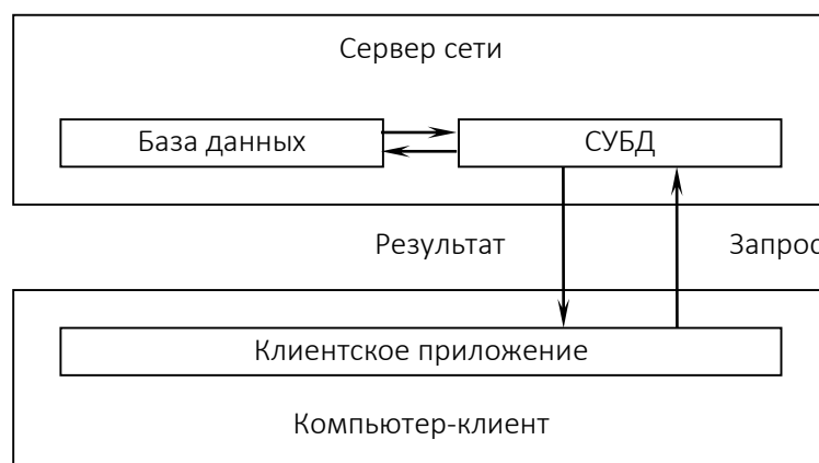
Рисунок 8.3. – Архитектура клиент-сервер
