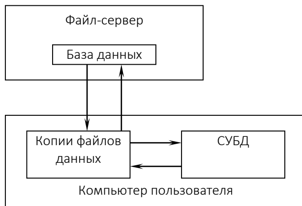
Рисунок 8.2. – Архитектура файл-сервер
