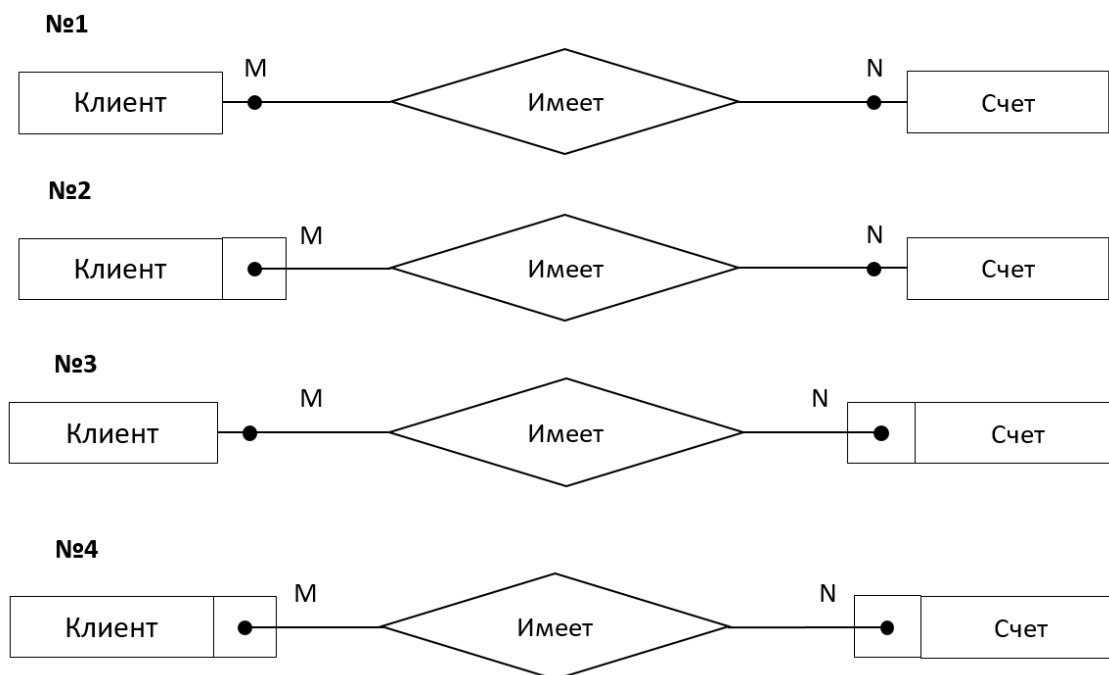
Рисунок 3.4. – ER-диаграммы связи M:N с учетом класса принадлежности сущности
