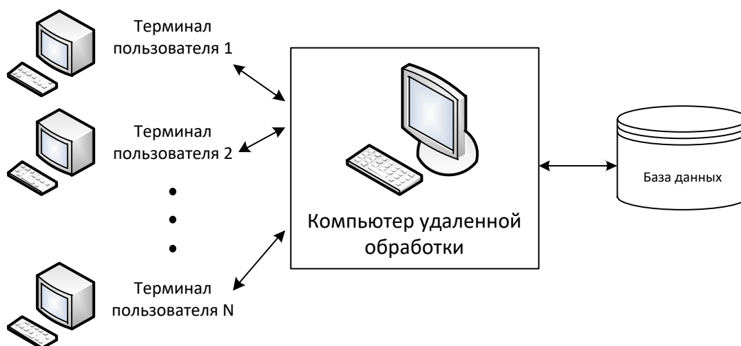
Рисунок 8.1. – Схема удаленной обработки многопользовательских БД
