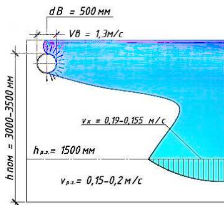
Рисунок 1. – Схема подачи воздуха через текстильный воздухораспределитель образец № 1 – боковая перфорация 180°, направленная под углом 90°
