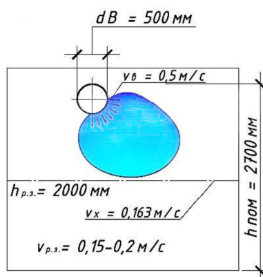
Рисунок 2. – Схема подачи воздуха через текстильный воздухораспределитель образец № 4 – микроперфорация 45°, направленная под углом 125°
