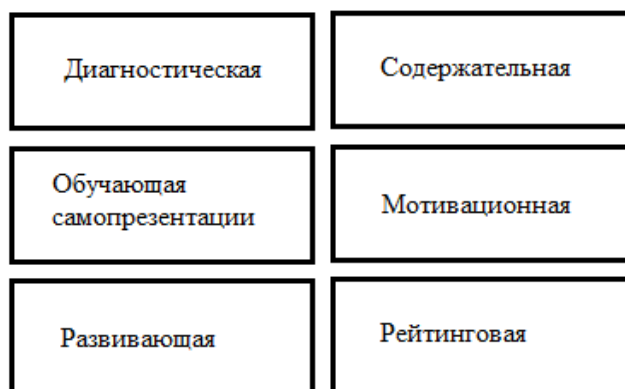
Рисунок 2. – Функции портфолио
