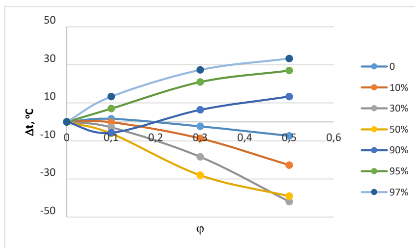
Рисунок 4. – График зависимости разности температур кипения дизельного топлива и смесей дизельного топлива с подсолнечным маслом от концентрации подсолнечного масла (цветные линии – контрольные точки кипения по ГОСТу).
