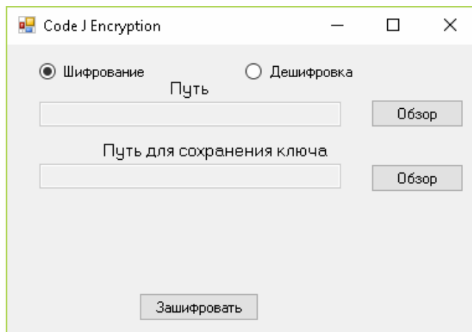
Рисунок 2. – Интерфейс шифрования
