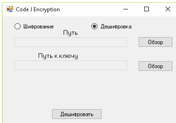
Рисунок 2. – Интерфейс дешифровки
