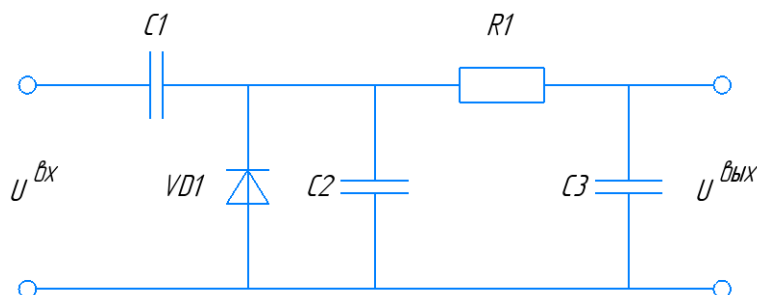
Рисунок 1. – Схема амплитудного преобразователя на германиевых диодах [2]
