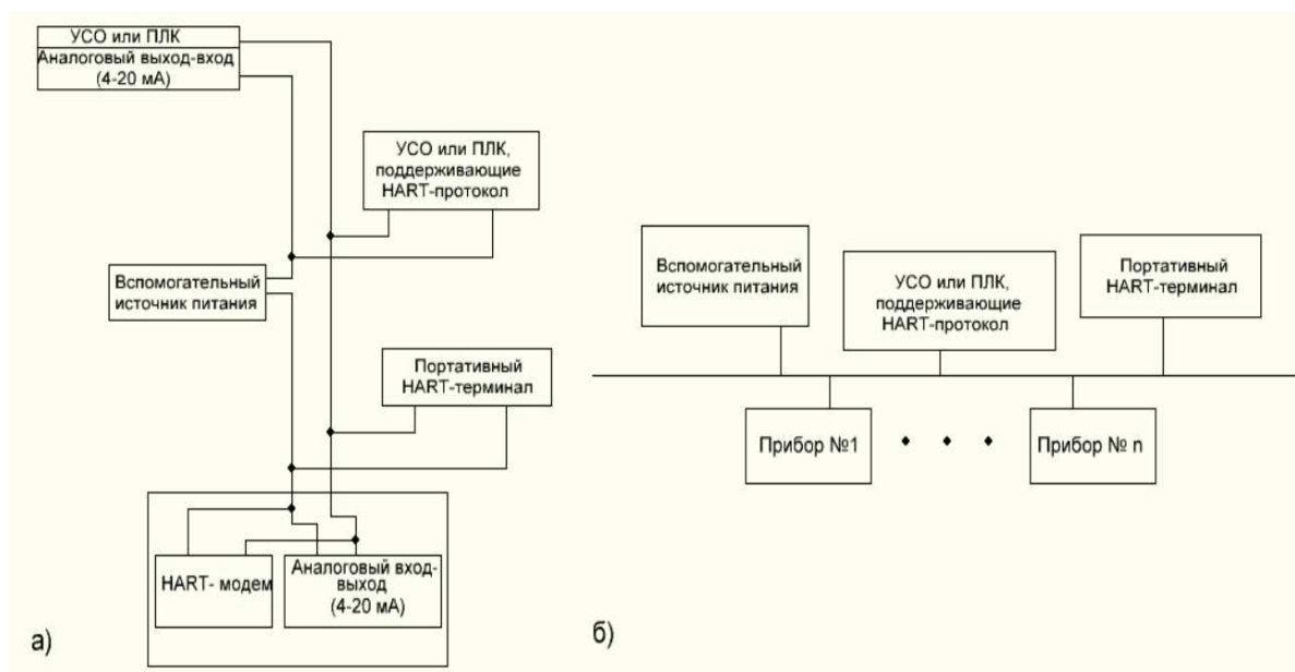
ПЛК – программируемый контроллер; УСО – устройство связи с объектом; ПК – персональный компьютер; a – стандартный вариант – цифровой канал «точка-точка» с аналоговым сигналом; б – многоточечный вариант – цифровой канал (топология-шина) без передачи аналогового сигнала, но с удаленным питанием по цепям связи
