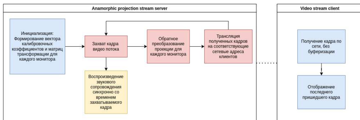
Рисунок 2. – Структурная схема системы синхронного анаморфного проецирования видео
