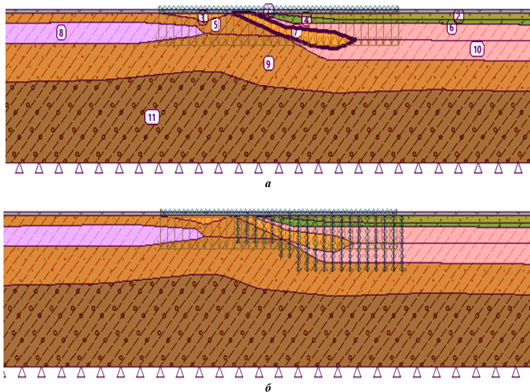
Рисунок 3. – Расчетные схемы фундамента для продольного разреза на естественном (а) и усиленном вертикальным армированием (б) основаниях
