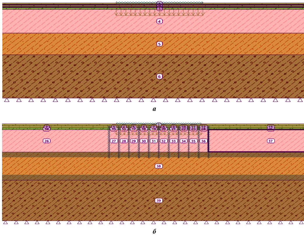
Рисунок 2. – Расчетные схемы фундамента на естественном (а) и усиленном вертикальным армированием (б) основаниях по скважине 15
