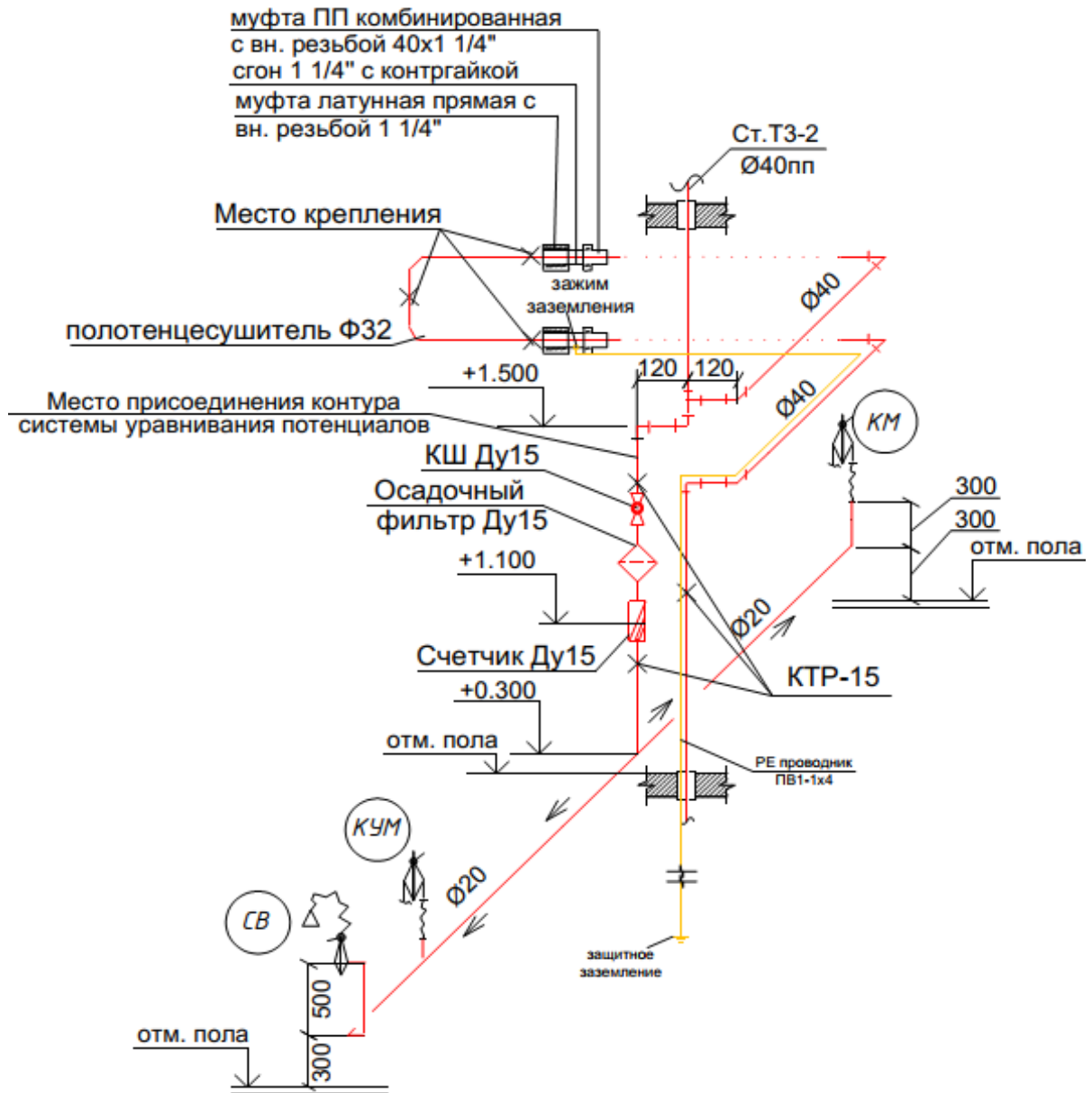
Рисунок 2.5. – Пример размещения водоразборной и запорной арматуры, счетчика расхода воды, фильтра, полотенцесушителя и подающих горячую воду трубопроводов на квартирном этажестояке
