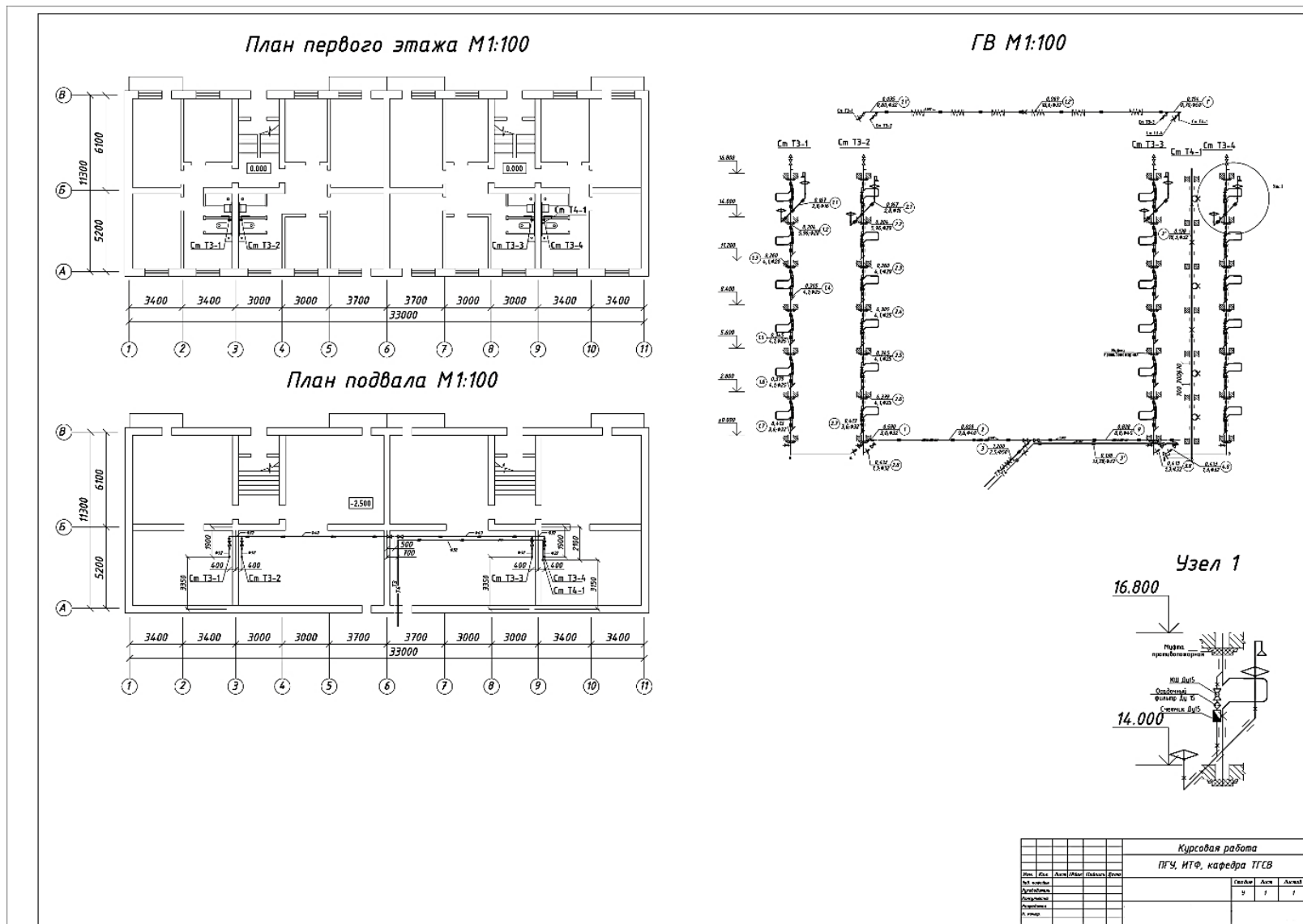
Рисунок 2.3. – Пример оформления результатов конструирования трубопроводов СГВ
