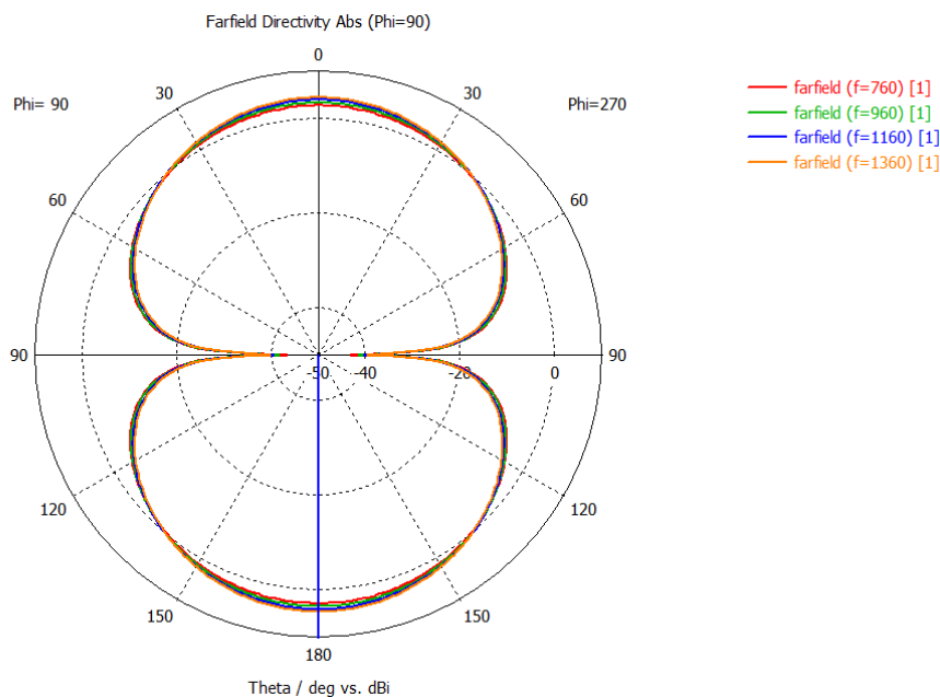
Рисунок 2. – ДН дипольной эллиптической антенны
