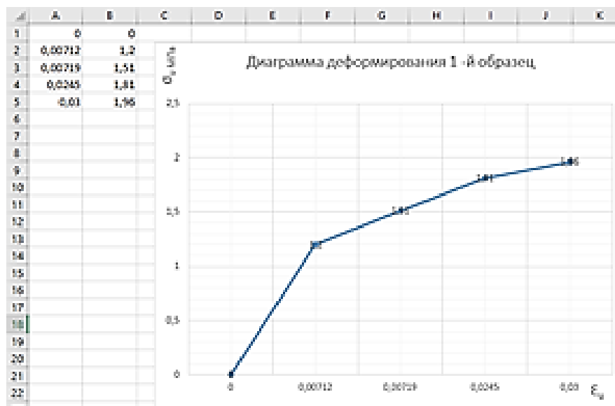
Рисунок 1. – Диаграмма деформирования 1-го образца
