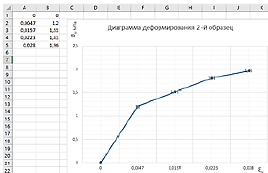
Рисунок 2. – Диаграмма деформирования 2-го образца
