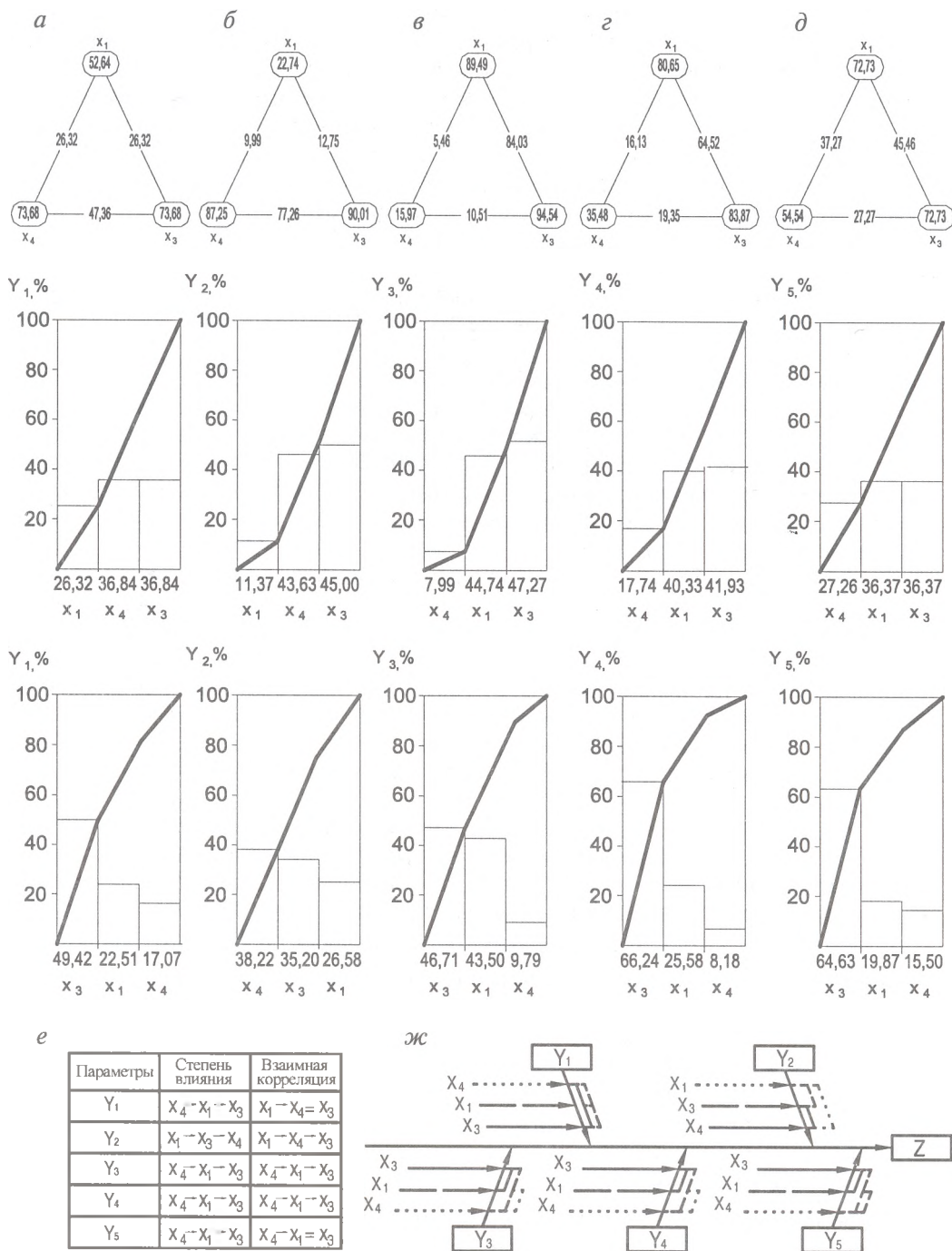
Рис. 2. Управление специальным процессом комбинированной упрочняюще-размерной термомеханической обработки износостойкого покрытия порошком ПГ-10Н-01 по комплексу параметров: HRC (а), U_H (б), Sp_w (в), Ra (г), K (д), с учетом влияния и взаимосвязи факторов (е) на диаграмме «причины—результат» (ж)
