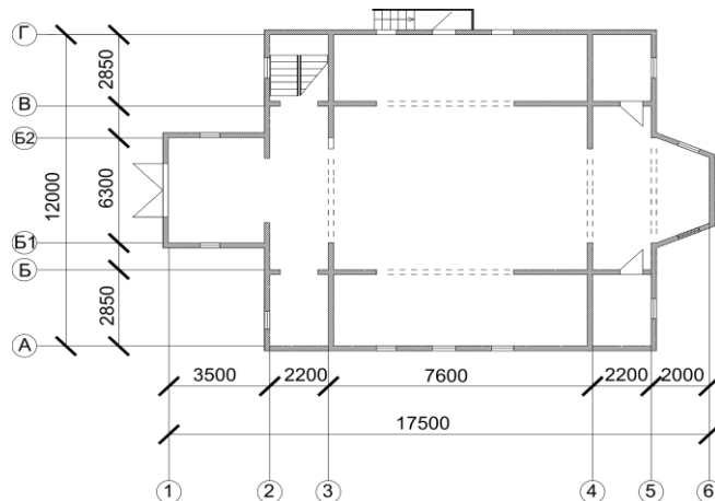
Рисунок 1. – План Свято-Никольского храма в Минске (чертеж авторов)
