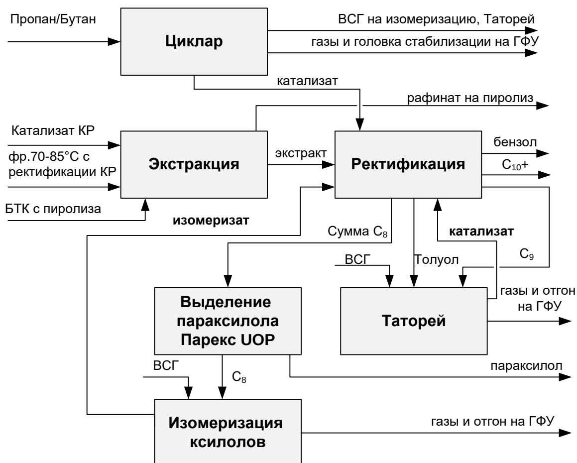
Рисунок 2.9. – Комплекс установок по получению индивидуальных ароматических углеводородов
