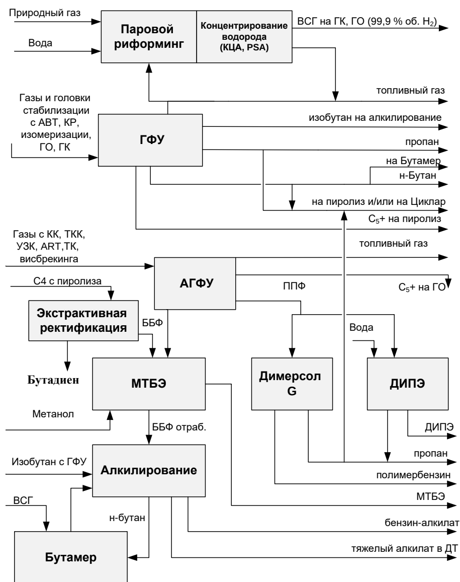
Рисунок 2.8. – Комплекс установок по переработке углеводородных газов, производству и концентрированию водорода
