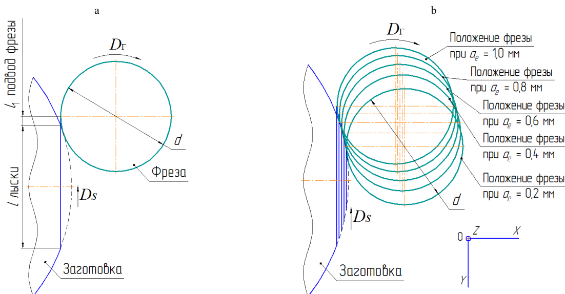
Рис. 5. Схема обработки лыски заготовки (a) и начальные положения фрезы при срезании слоя с глубиной врезания a_{ei} (b)
