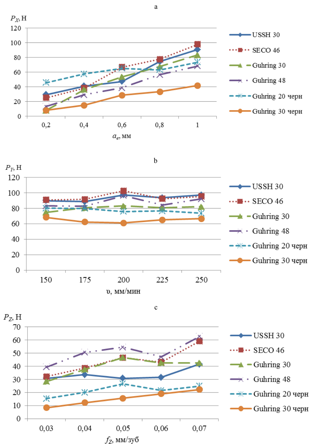
Рис. 9. Графики изменения составляющих P_x , P_y , P_z силы резания для различных фрез в зависимости от глубины врезания a_e (a), скорости резания v (b) и подачи на зуб f_z (c) Fig. 9. Graphs of changes in the components P_x , P_y , P_z of the cutting force for various cutters depending on the cutting depth a_e (a), cutting speed v (b) and feed to the tooth f_z (c)
