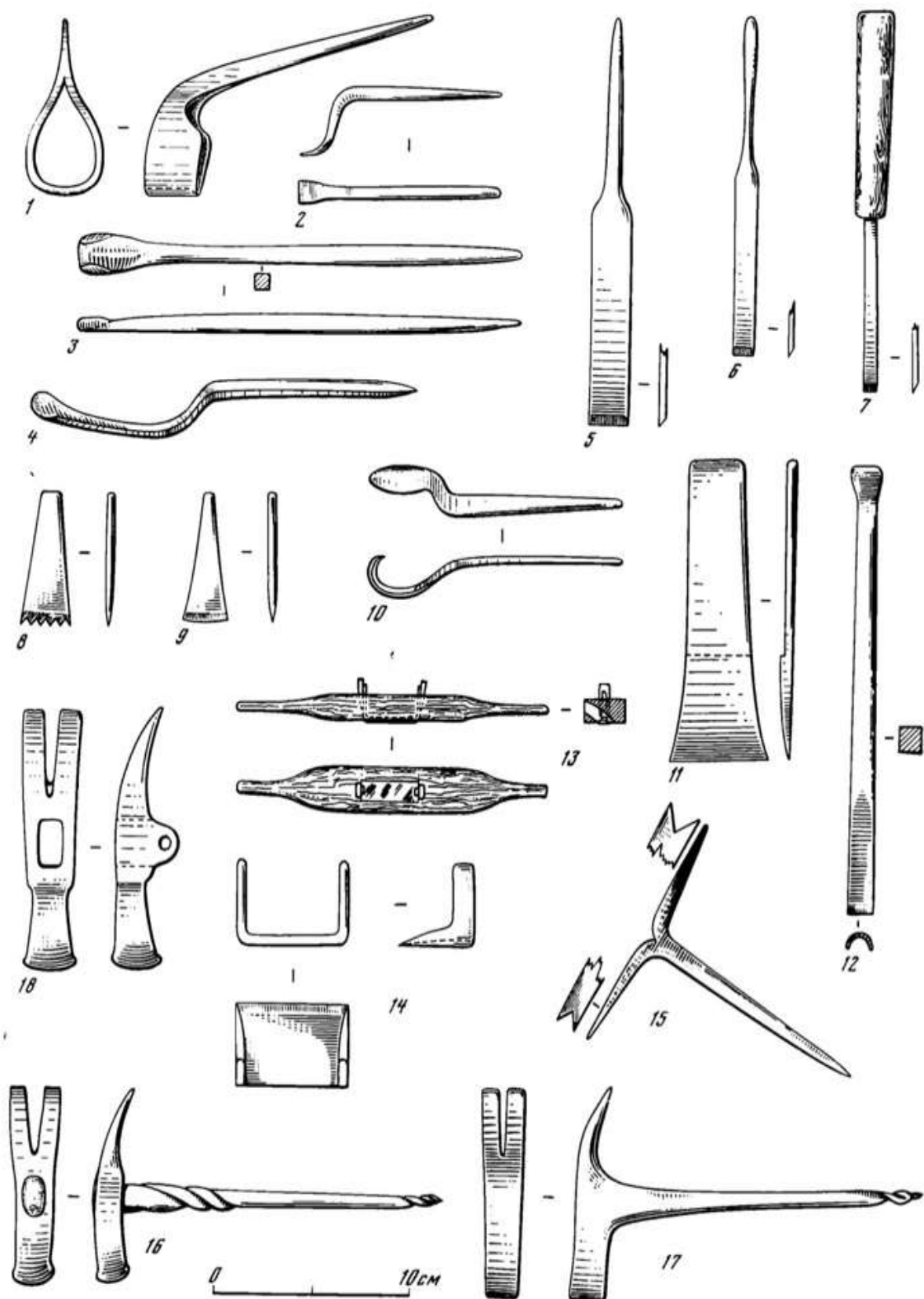
1 – бондарная скобелка; 2–4 – резцы по дереву; 5–7 – стамески; 8–9 – уторные пилки; 10 – резец-ложкарь; 11 – лезвие от рубанка; 12 – долото; 13–14 – наструг; 15 – чертилка; 16–18 – молотки-гвоздодеры
