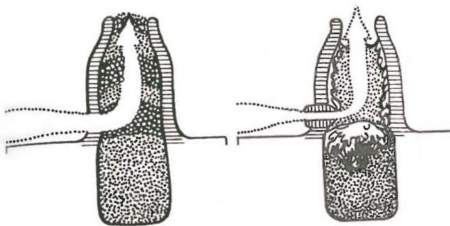
Рисунок 22. – Реконструкция сыродутного процесса (по В.Л. Янину)
