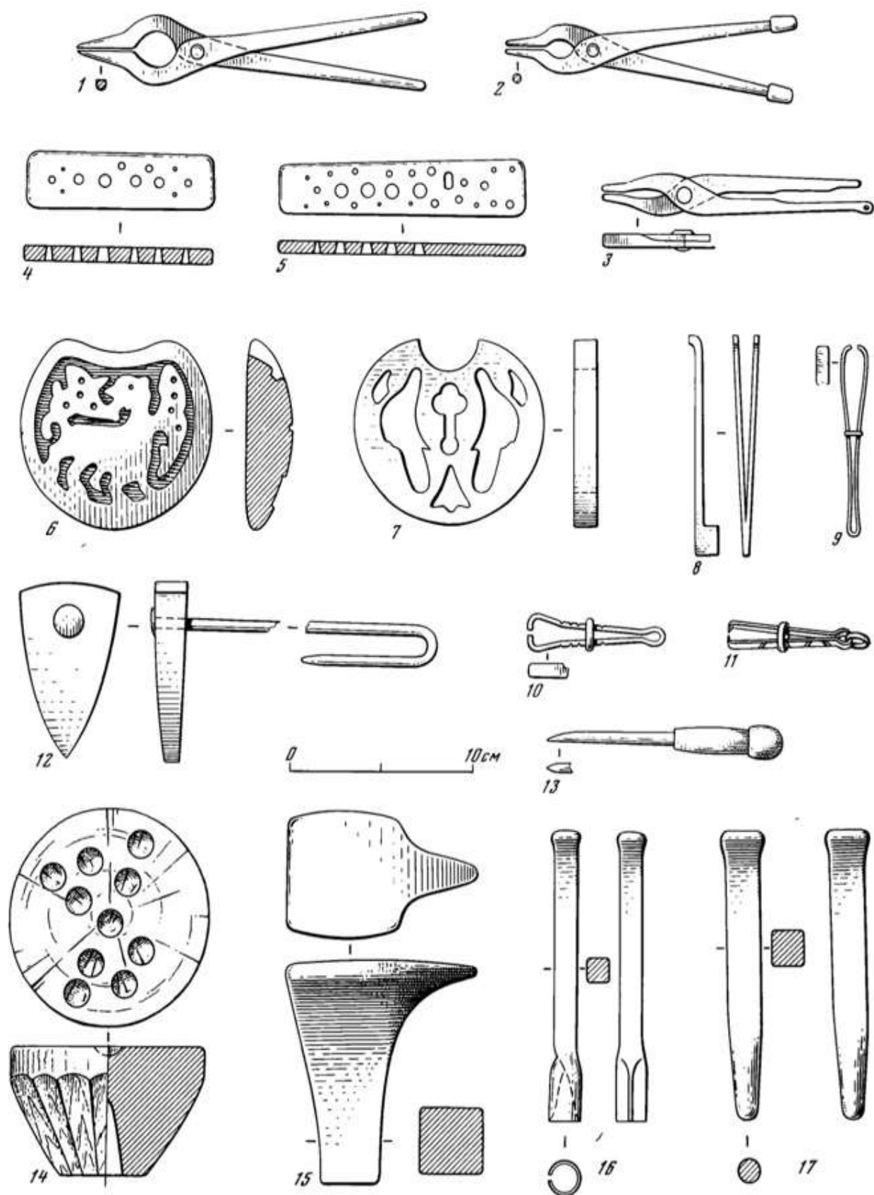
1-3 – клещи-плоскогубцы и круглогубцы; 4-5 – волочильные доски; 6, 7 – матрицы для изготовления колтов; 8-11 – пинцеты; 12 – паяльник; 13 – резец по металлу; 14 – деревянная наковальня; 15 – наковальня; 16 – пуансон; 17 – чекан
