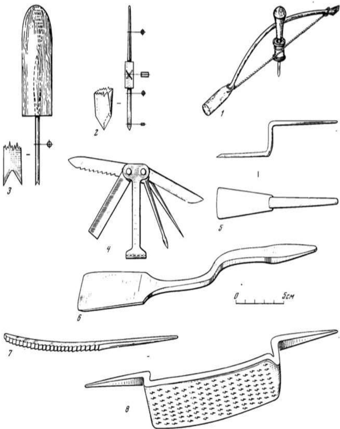
1 – лучковое сверло; 2 – рабочая часть лучкового сверла; 3 – циркульный резец; 5, 6 – резцы для снятия мездры; 7 – напильник; 8 – рашпиль Рисунок 13. – Инструменты для обработки кости в Древней Руси (по Б.А. Колчину)
