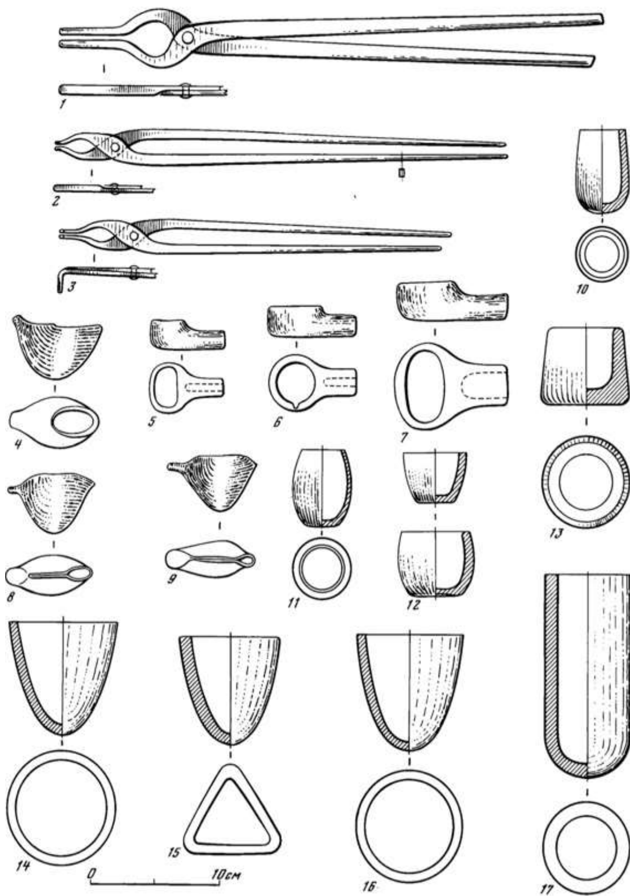
1–3 – тигельные клещи; 4–7 – льячки; 8, 9 – тигли-ляжки; 10–17 – тигли Рисунок 18. – Инструменты литейщика
