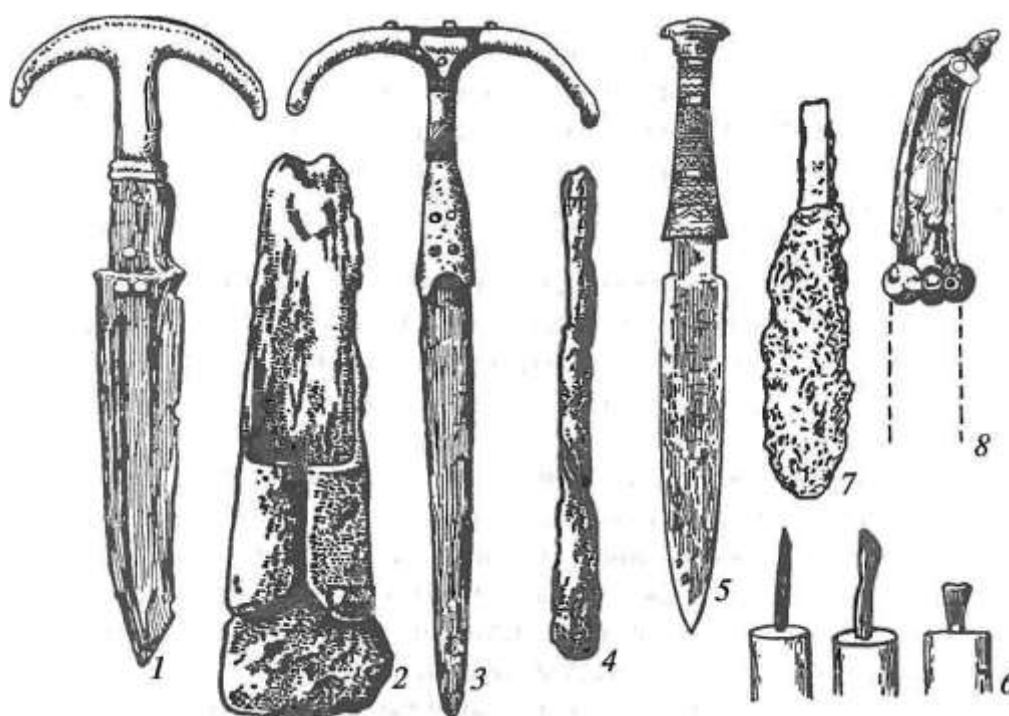
1, 3 – железные кинжалы с рукоятью, обложенной золотом (Ур, Аладжа-Хейюк); 2, 4 – железное тесло с медным захватом для рукояти и железное долото (древняя культура); 5, 6 – кинжал и железные лезвия (гробница Тутанхамона), 7 – нож с медной рукоятью (катакомбная культура); 8 – железная рукоять кинжала (Словакия)
