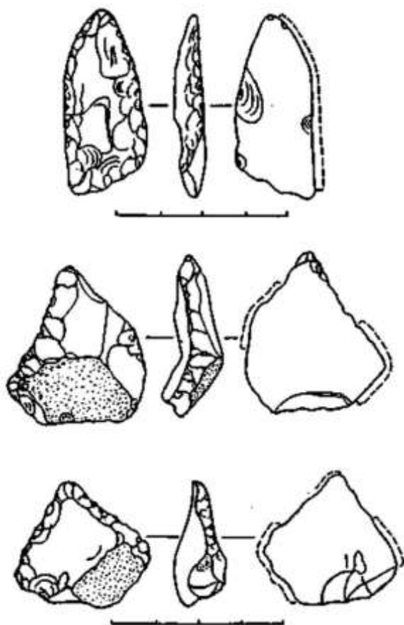
Рисунок 8. – Кремневые скобели для обработки дерева и кости эпохи мустье (по С.А. Семёнову)
