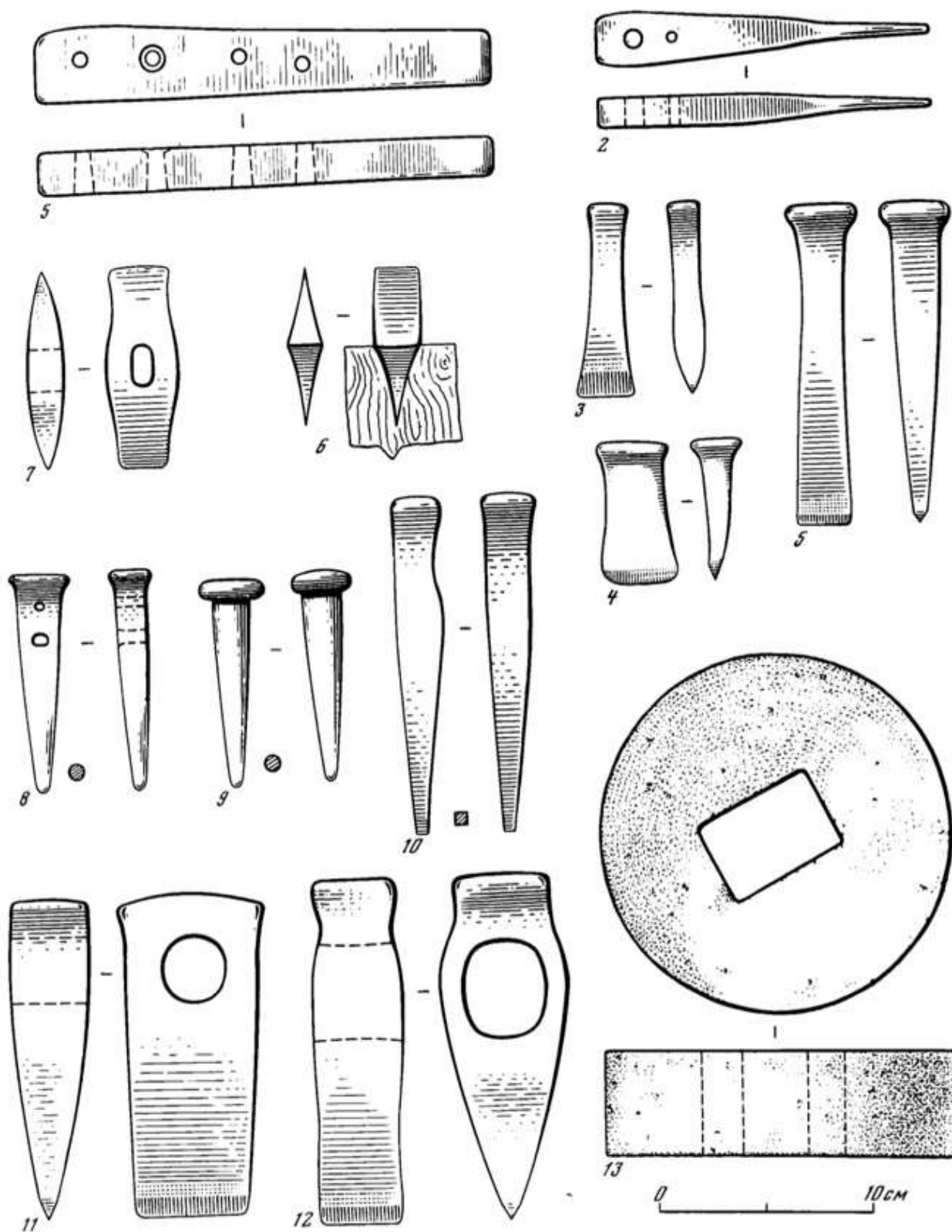
1, 2 – гвоздильни; 3-5 – зубила; 6 – кузнечная подсека; 7 – зубильный молоток, 8-10 – пробойники, бородки; 11-12 – зубила для горячей рубки; 13 – наждачный круг
