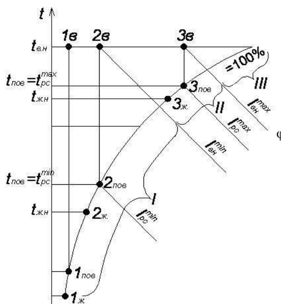
Рисунок 4 – I - d диаграмма с изображением параметров воздуха и жидкости для различных условий работы воздухоохладителя: I – «сухой» теплообмен; II – конденсация на части поверхности; III – конденсация на всей поверхности
