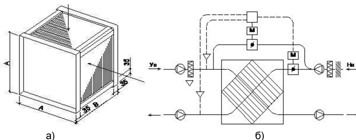
Рисунок 2 – а) схема перекрестно-точного пластинчатого рекуперативного теплообменника; б) схема компоновки диагонального теплообменника в установке с учетом исключения инеобразования
