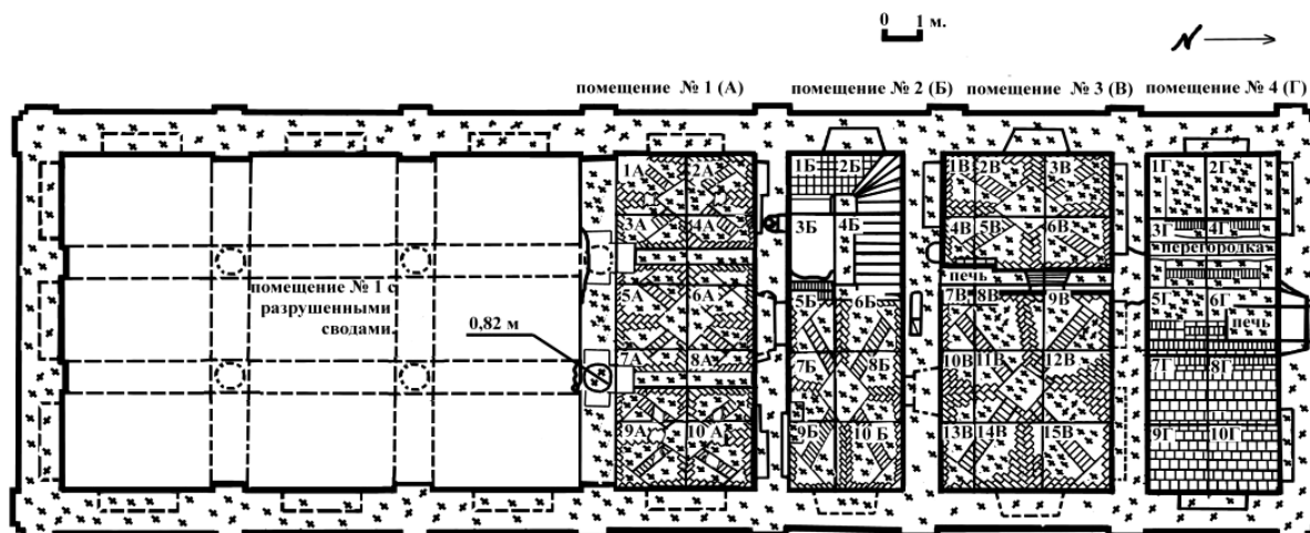
Рис. 2. План остатков второго этажа после расчистки от засыпки сводов
