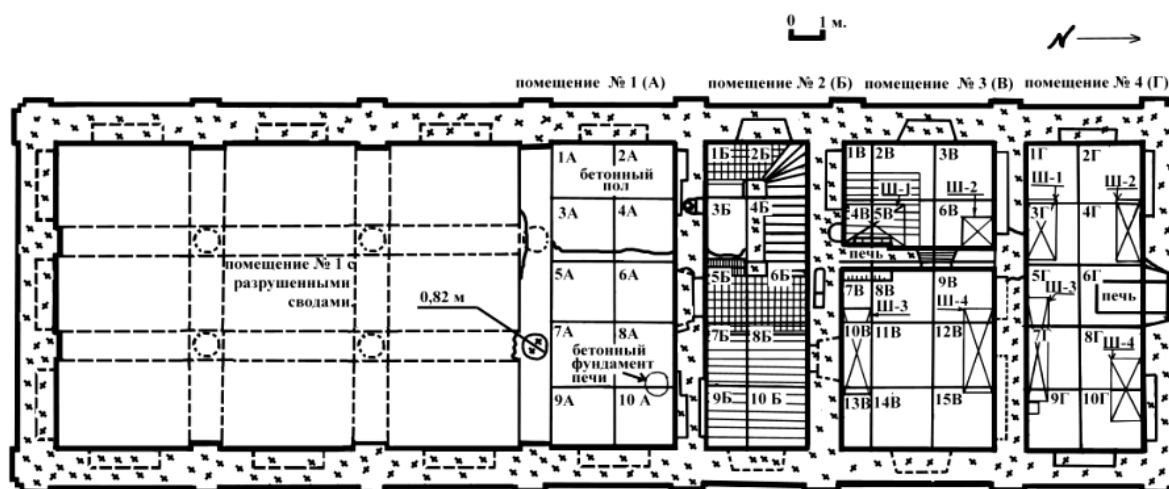
Рис. 1. План остатков второго этажа после снятия крыши и расположение шурфов
