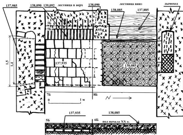
Рис. 4. Фрагмент помещения № 2
