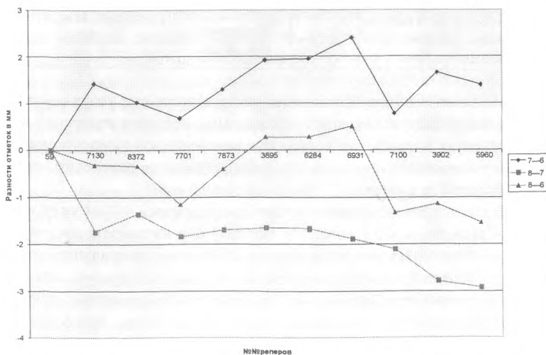
Рис. 2. Графики вертикальных движений нивелирных знаков на Полоцком профиле
