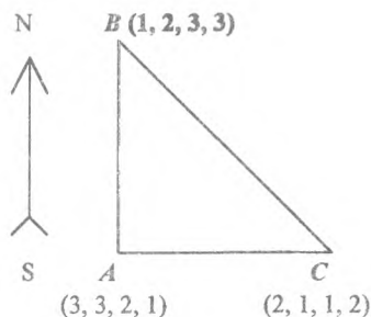
Рис. 4. Схема эталонного GPS-полигона
